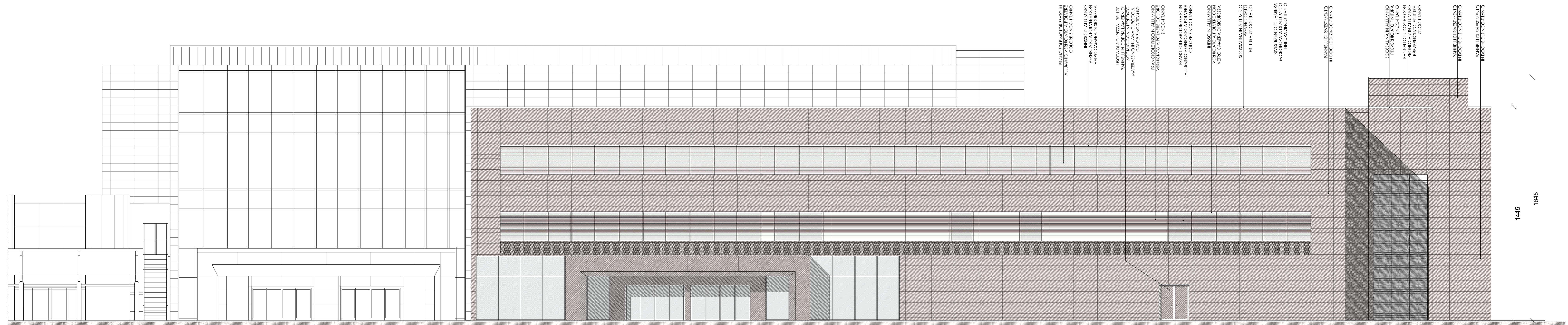
PROSPETTO LANDSIDE
