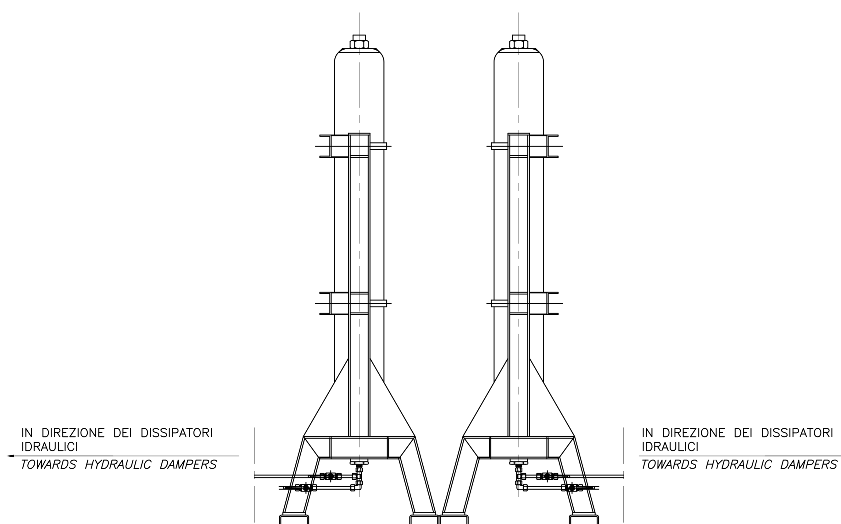
SEZIONE A-A NON IN SCALA SECTION A-A NOT TO SCALE
