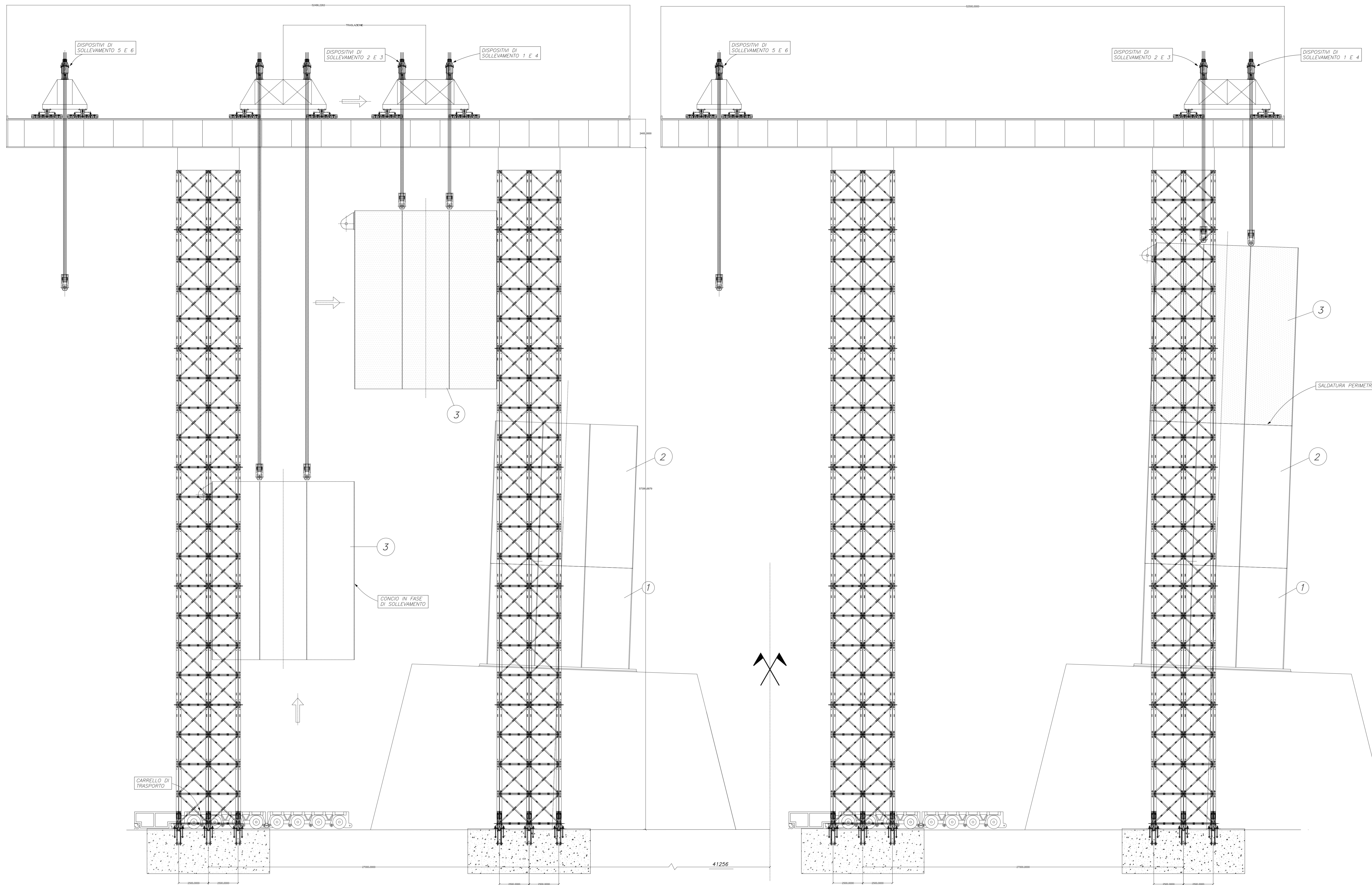
...SOLLEVAMENTO E TRASLAZIONE DEL CONCIO 3 VERSO LA POSIZIONE DI MONTAGGIO.
