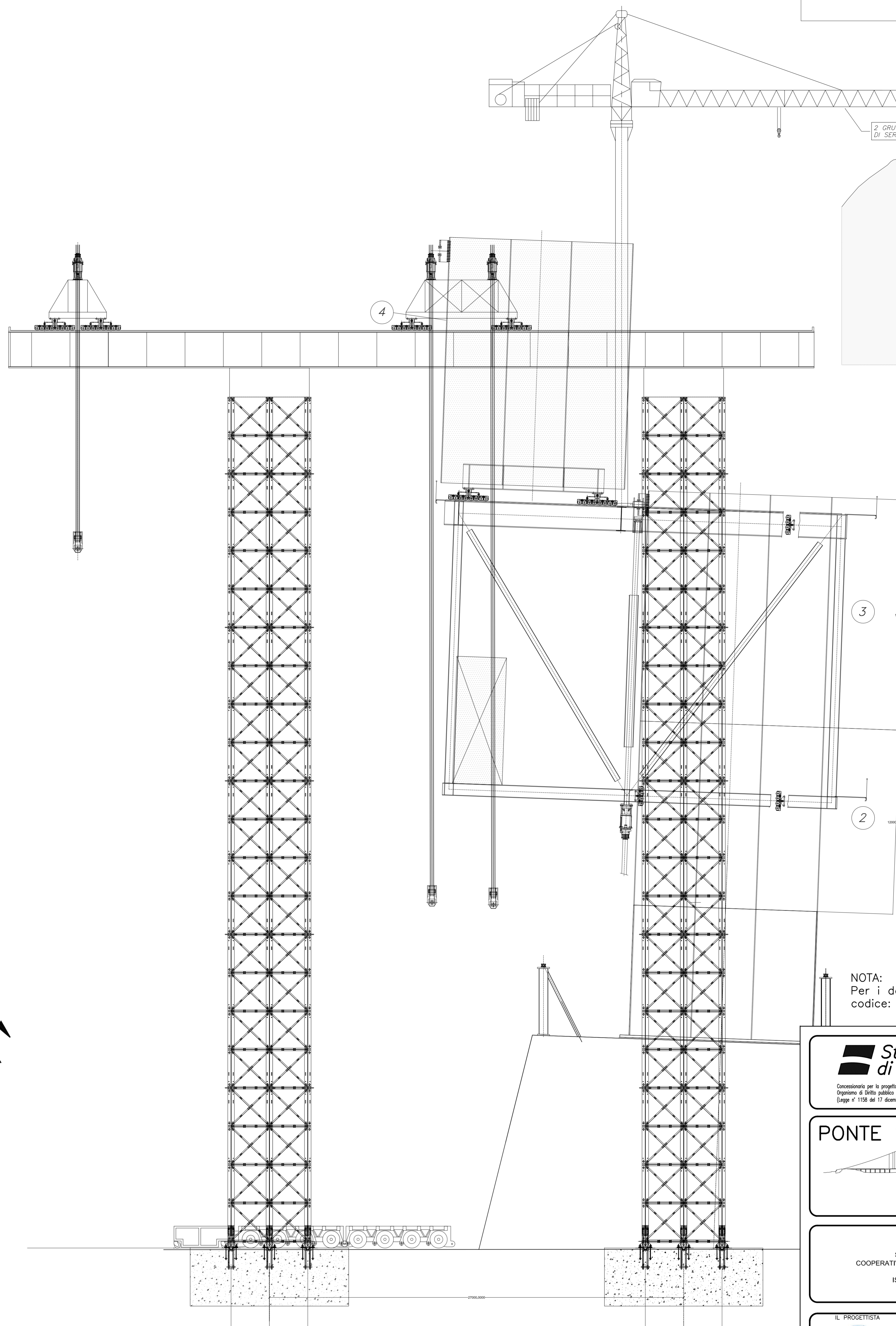
SOLLEVAMENTO DELL'ATTREZZATURA CON IL CONCIO 4 FINO ALLA QUOTA DI TRASLAZIONE
