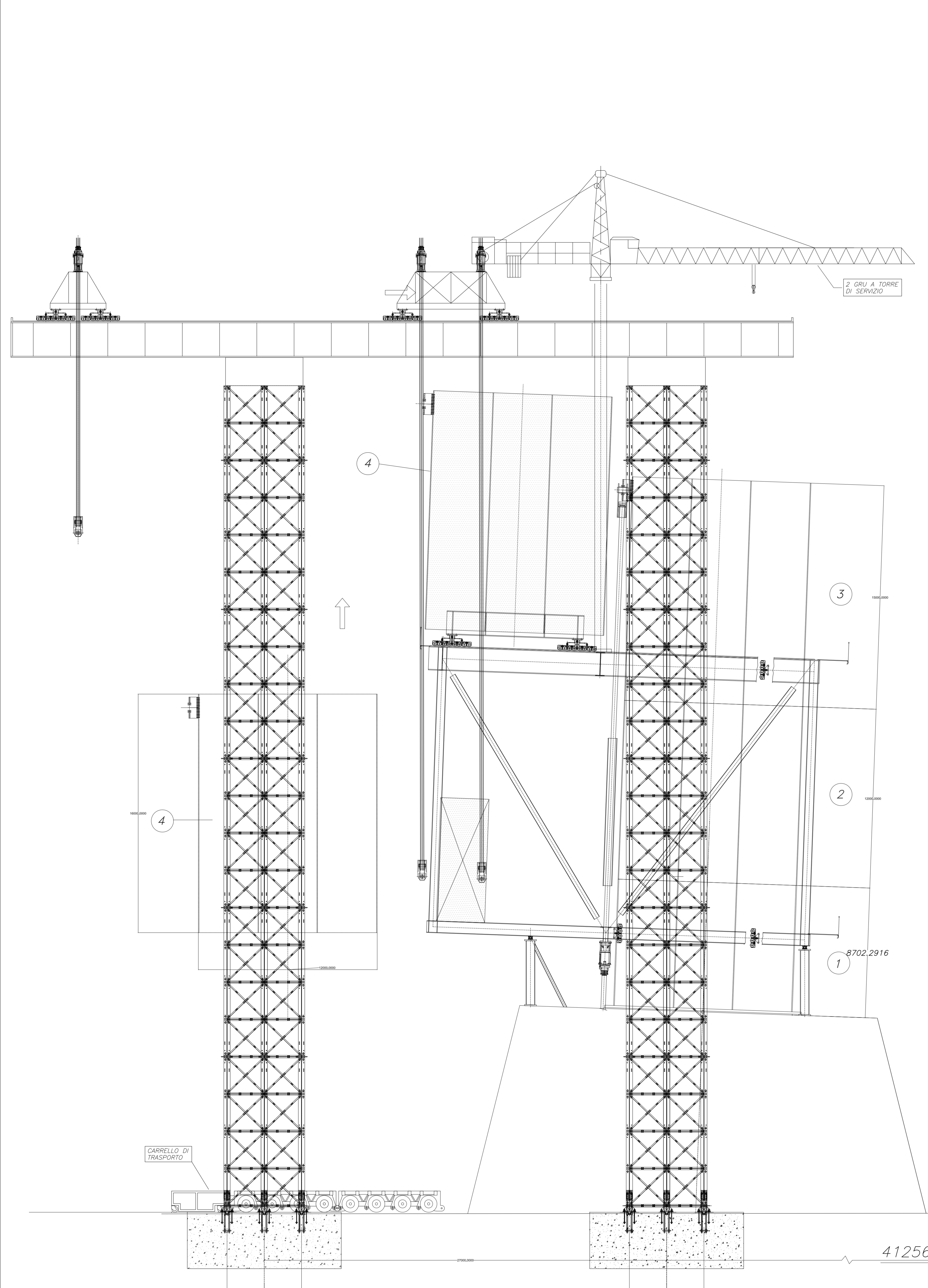
SOLLEVAMENTO E COLLOCAZIONE DEL CONCIO 4 SULLE GUIDE DELL'ATTREZZATURA
