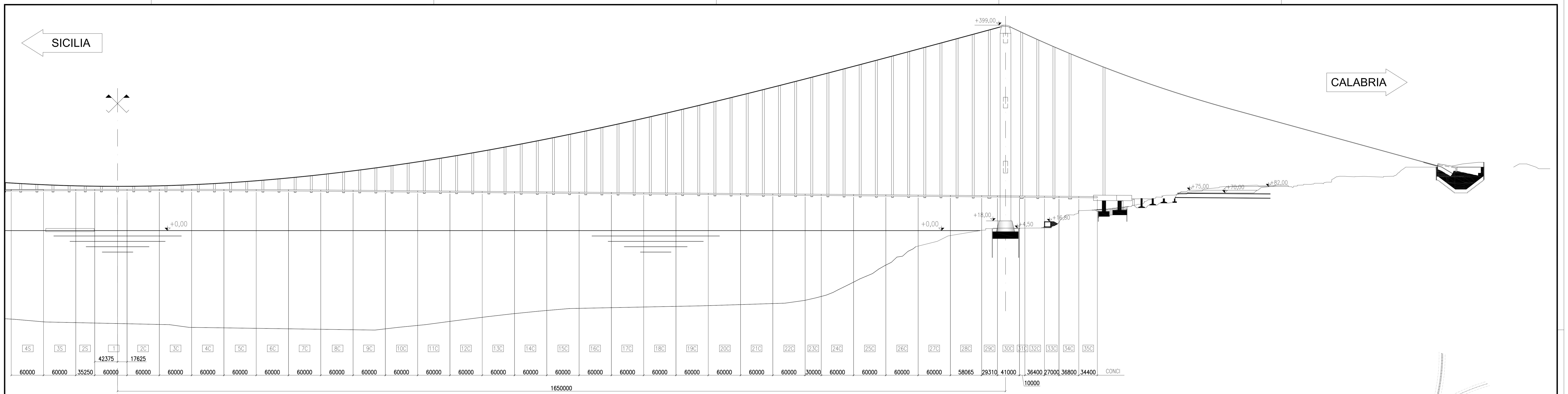
PROSPETTO LATO CALABRIA Scala 1:2500
