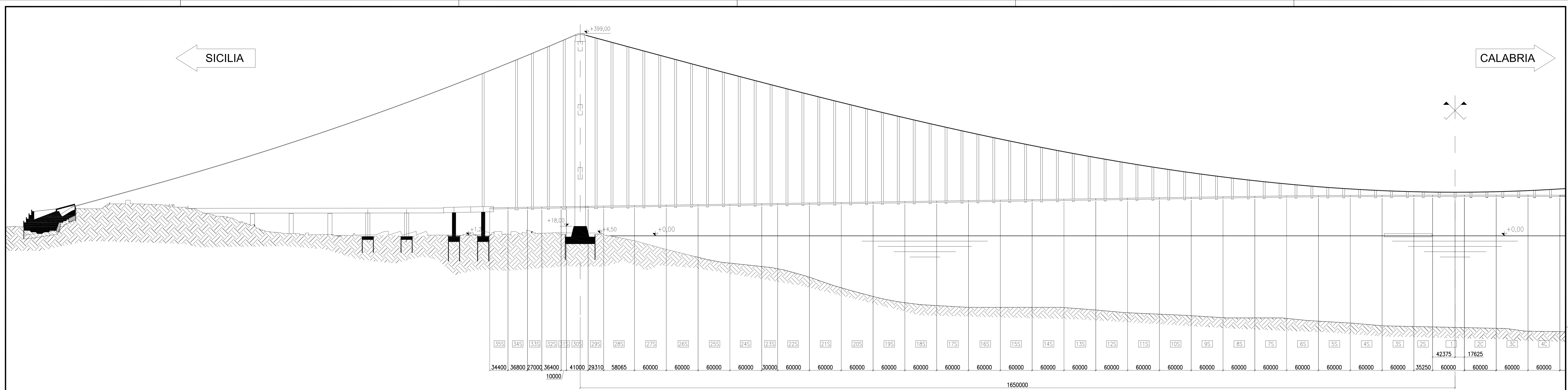
PROSPETTO LATO SICILIA Scala 1:2500
