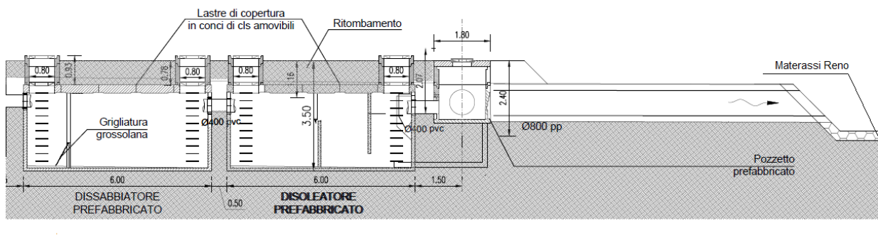
Figura 13: Scarico da vasca in corpo idrico ricettore
