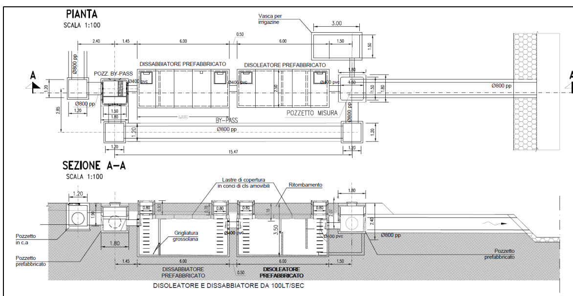
Figura 11: Vasca di prima pioggia
