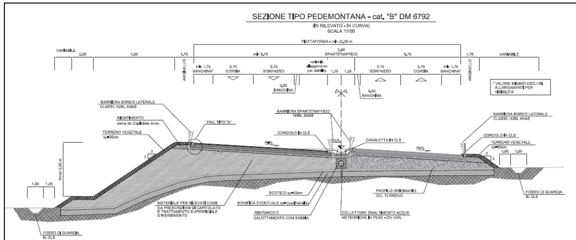
Figura 3: Schema del drenaggio per tratti in curva, con sistema di raccolta di tipo chiuso inter-carreggiata
