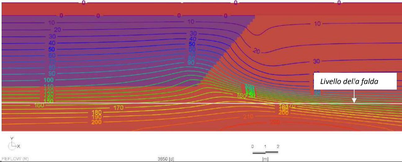
Figura 29 – Distribuzione delle isocrone [giorni] dopo 10 anni di percolazione delle particelle attraverso il deposito dei materiali di smarino, assumendo una porosità del deposito pari al 30%. Si può osservare come l'isocrona t=0 corrisponda alla superficie del deposito.
