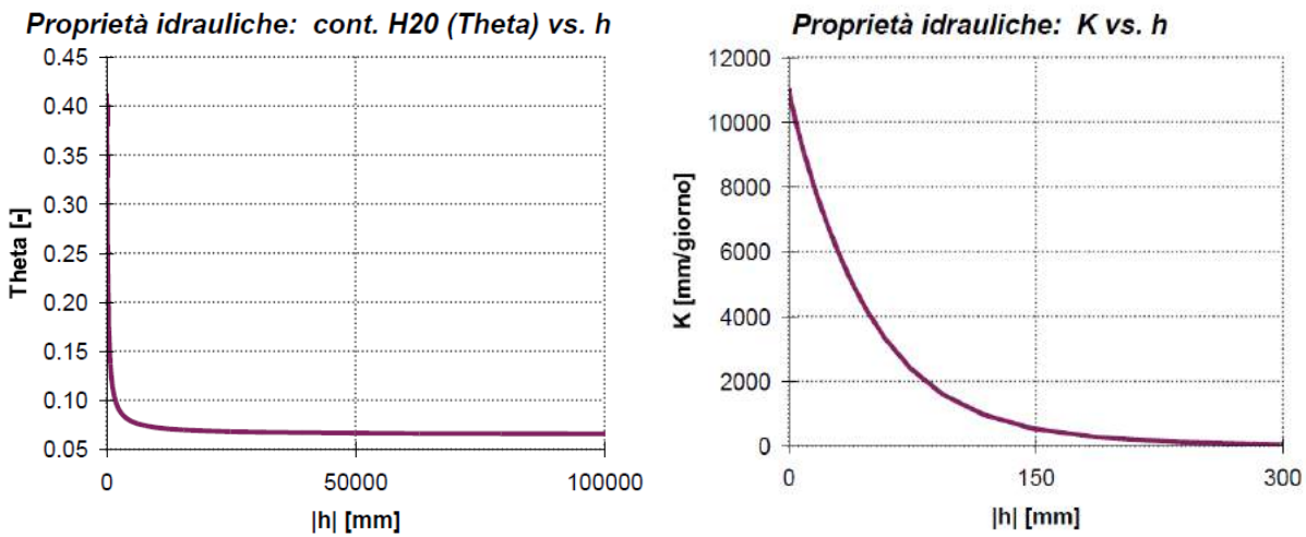
Figura 26 – Rappresentazione grafica delle proprietà dei materiali (contenuto d’acqua vs. carico idraulico e conducibilità idraulica vs. carico idraulico) derivante dall’adozione dei parametri illustrati nella figura precedente.
