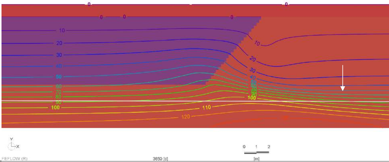
Figura 30 – Distribuzione delle isocrone [giorni] dopo 10 anni di percolazione delle particelle attraverso il deposito di materiali, assumendo una porosità dei materiali di smarino pari al 15%. Si può osservare come l'isocrona t=0 corrisponda alla superficie del deposito.
