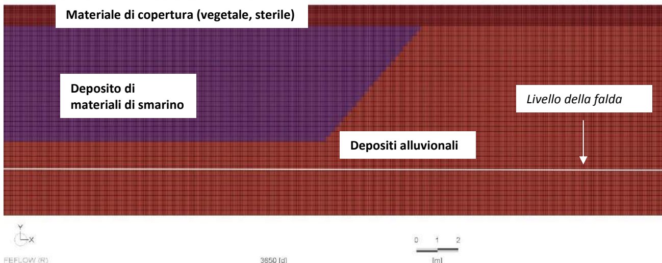
Figura 28 – Geometria del modello realizzato in sezione verticale con rappresentazione dei vari materiali considerati nella simulazione per il settore di terreno insaturo.
