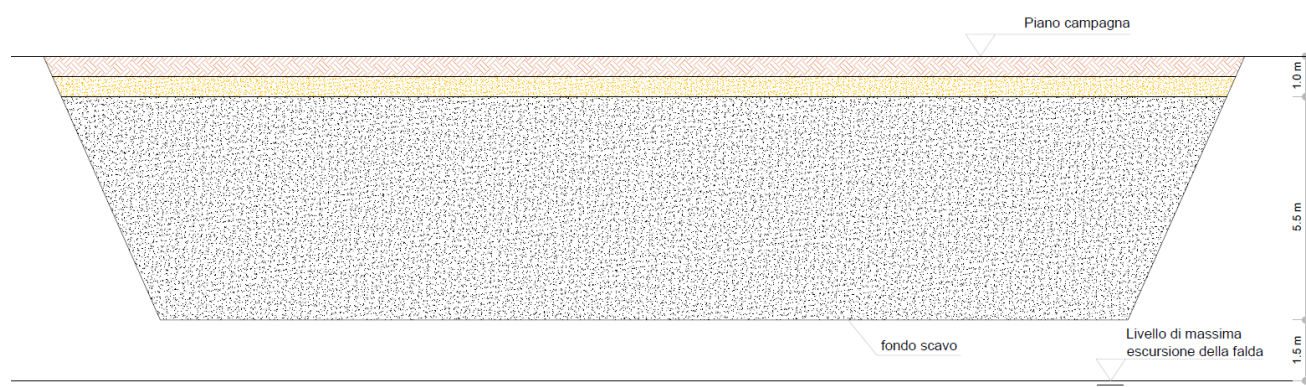
Figura 1 – Sezione tipologica della riqualifica
