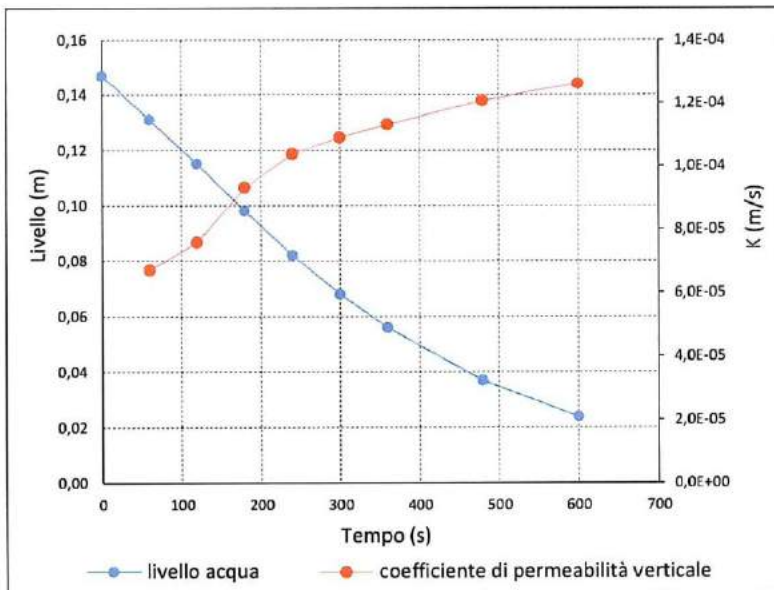
Figura 5 - Fotografia relativo al test di infiltrazione e grafico relativo al monitoraggio degli abbassamenti del livello nel tempo.
