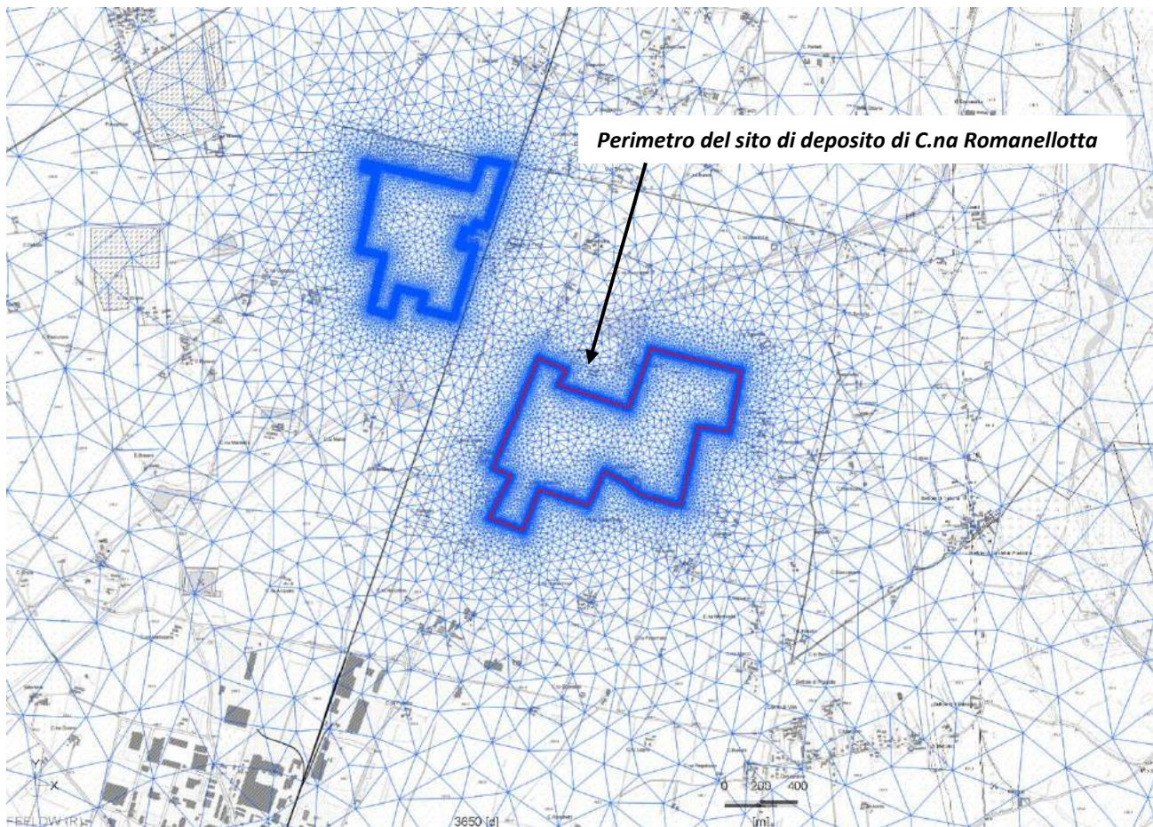
Figura 33 – Geometria della griglia di elementi finiti triangolari utilizzati per la simulazione 2D di flusso e di massa in falda.
