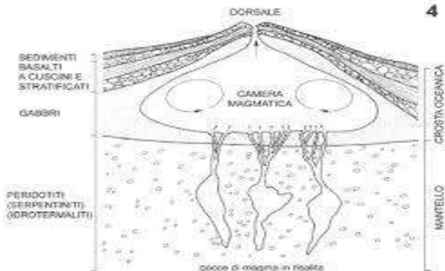
Figura 1. Formazione e composizione delle ofioliti (fonte: Calanchi , 1999)
