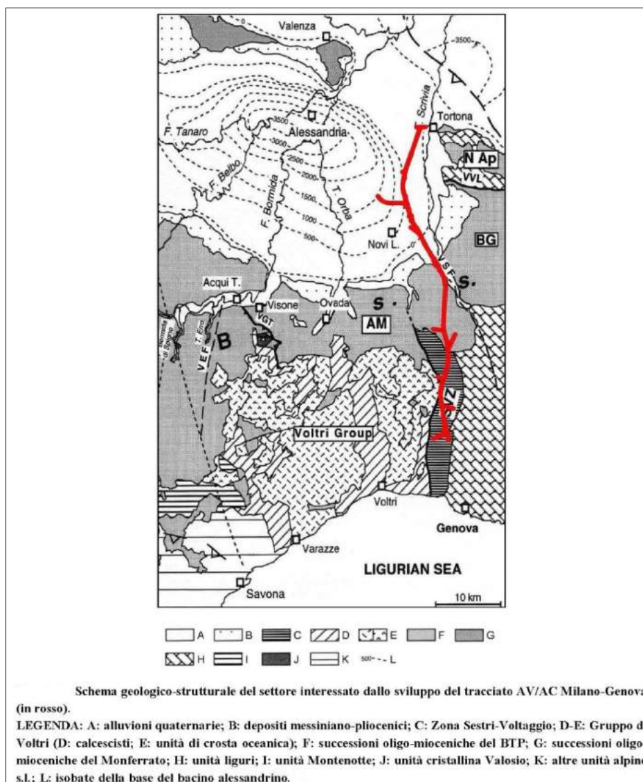
Figura 1 – Schema geologico strutturale del settore interessato dalla realizzazione del Terzo Valico
