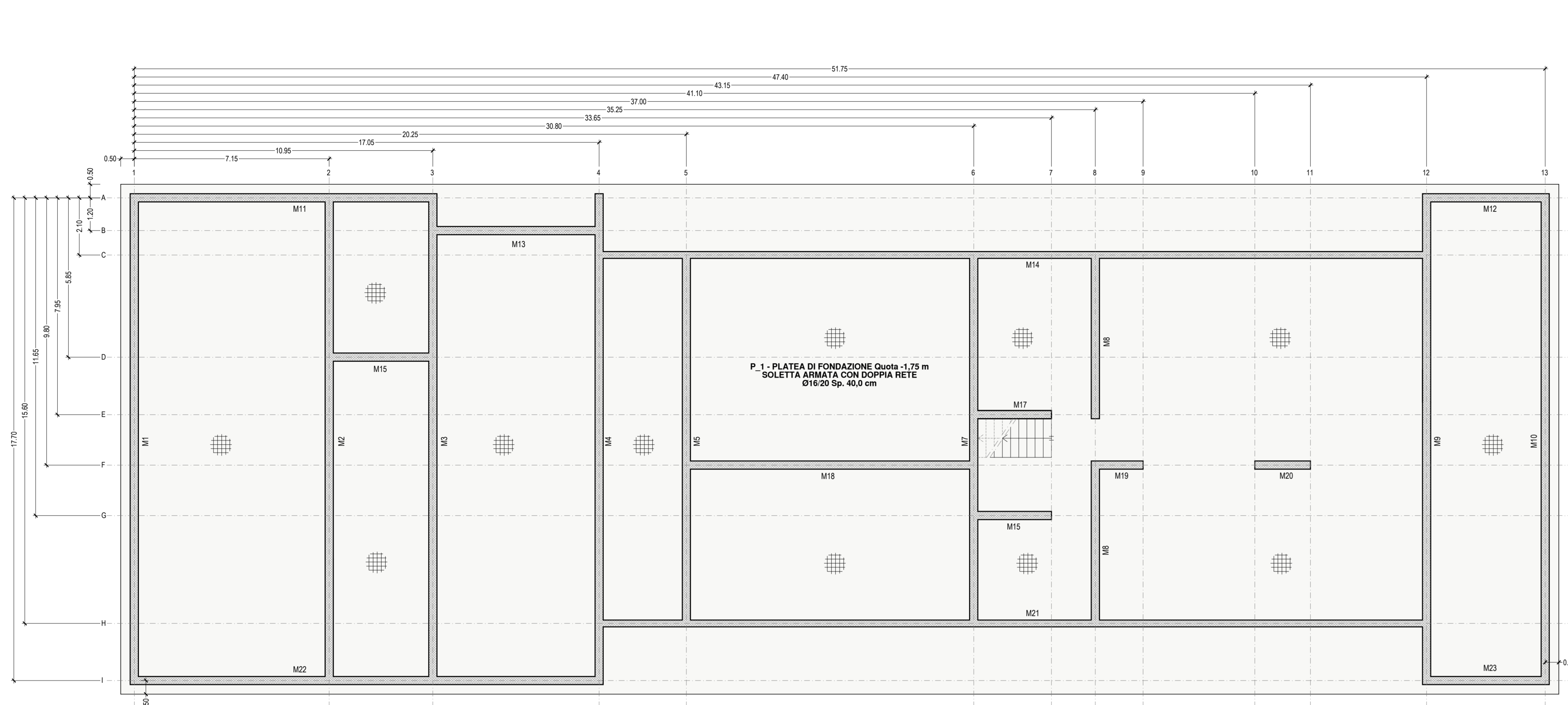
PIANTA DELLE FONDAZIONI A QUOTA -1,75 m - Scala 1:100
