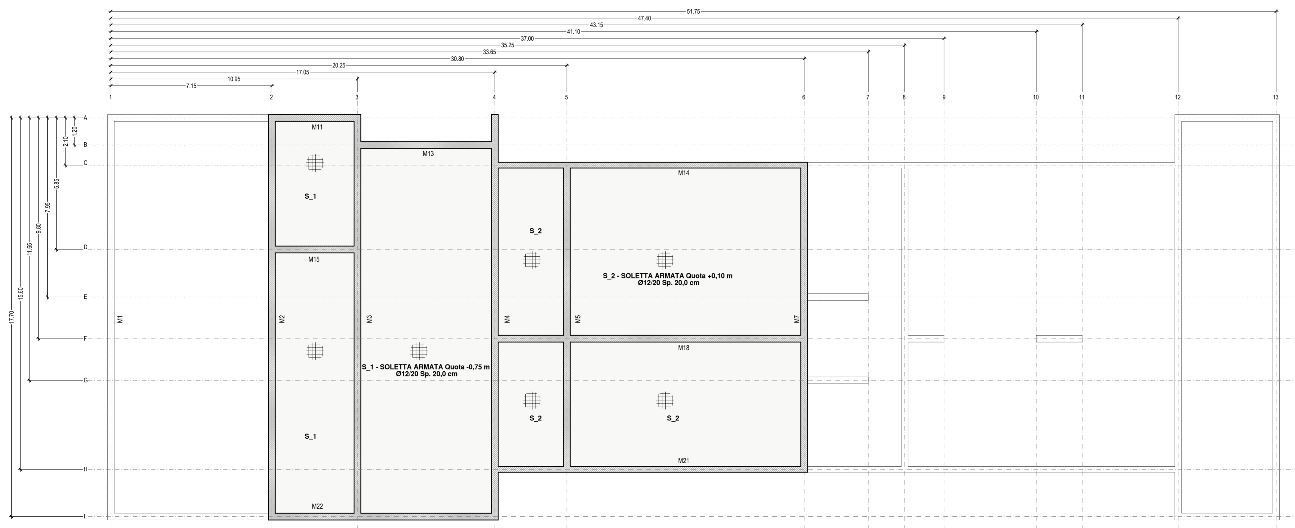
CARPENTERIA A QUOTA -0.75 E +0.10 - Scala 1:100
