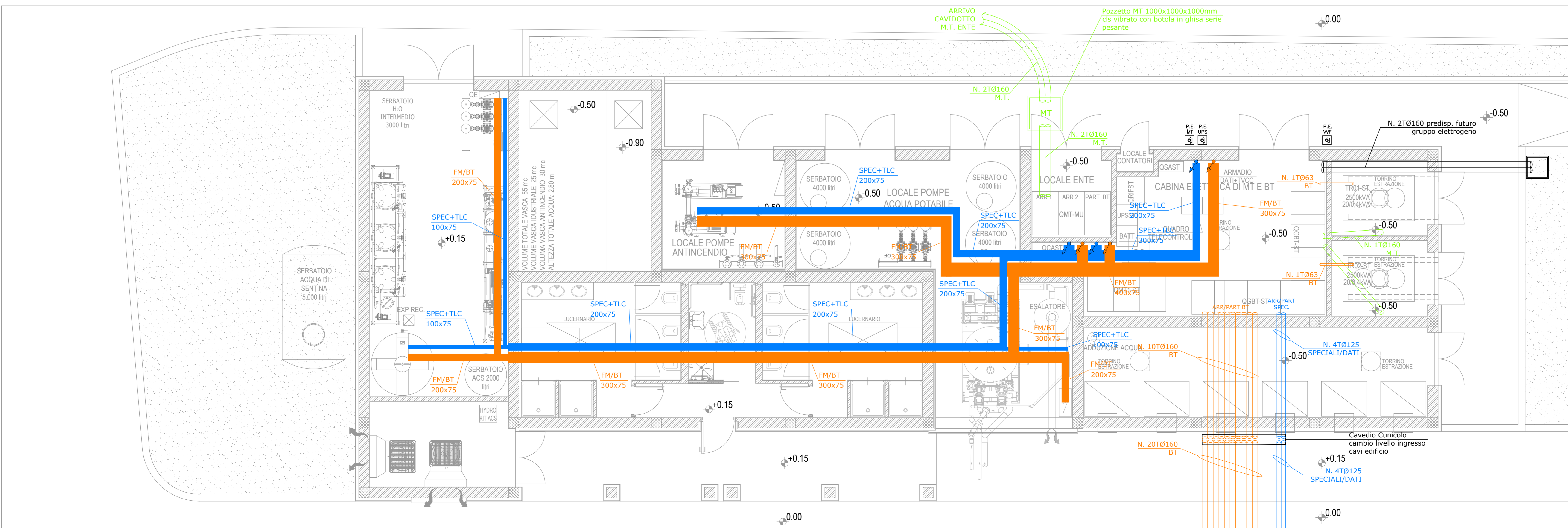
PLANIMETRIA CANALIZZAZIONI ELETTRICHE - EDIFICIO SERVIZI SAN TEOFANIO Scala 1:50
