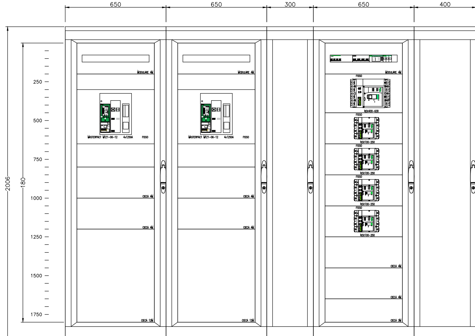
QGBT-PU FRONTE QUADRO GENERALE BASSA TENSIONE PORT UTILITIES
