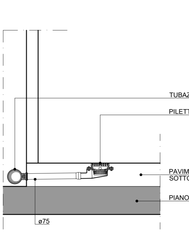
DETTAGLIO SCARICO PILETTA
