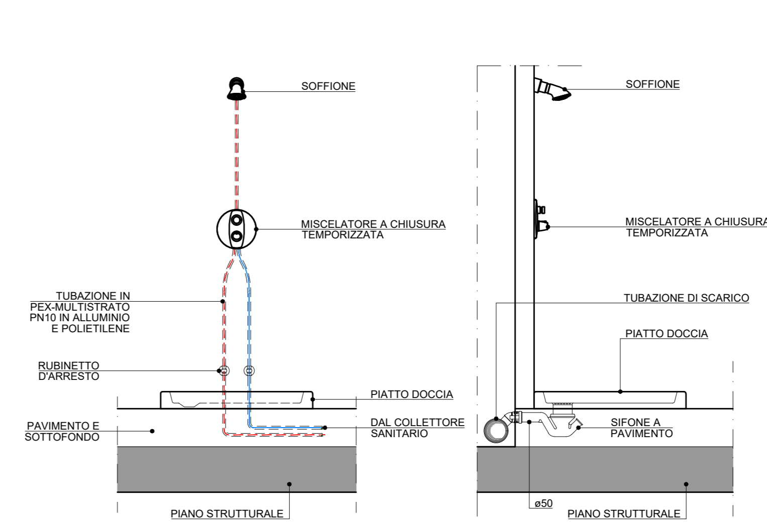
DETTAGLIO ALLACCIO E SCARICO DOCCIA
