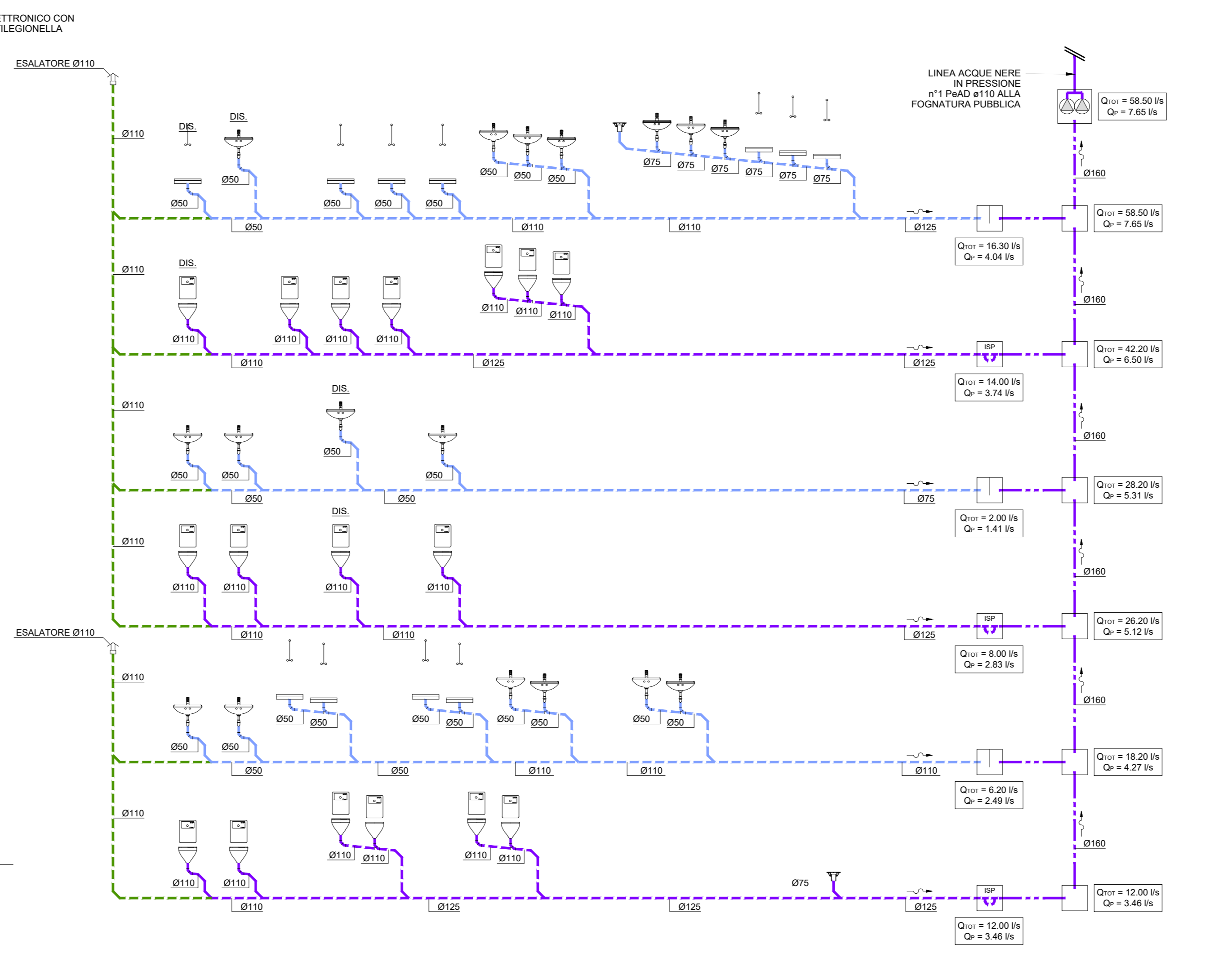
SCHEMA FUNZIONALE IMPIANTO DI SCARICO
