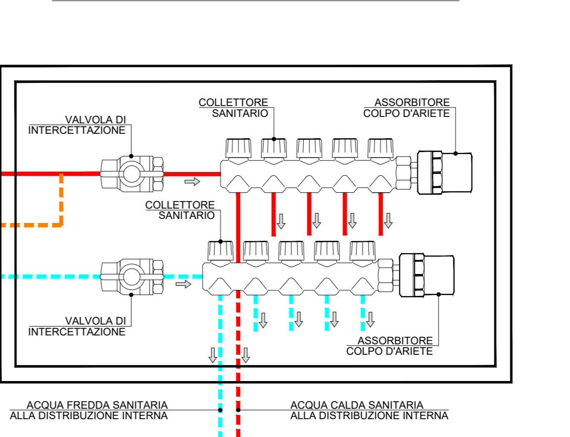
SCHEMA STANDARD COLLETTORE SANITARIO
