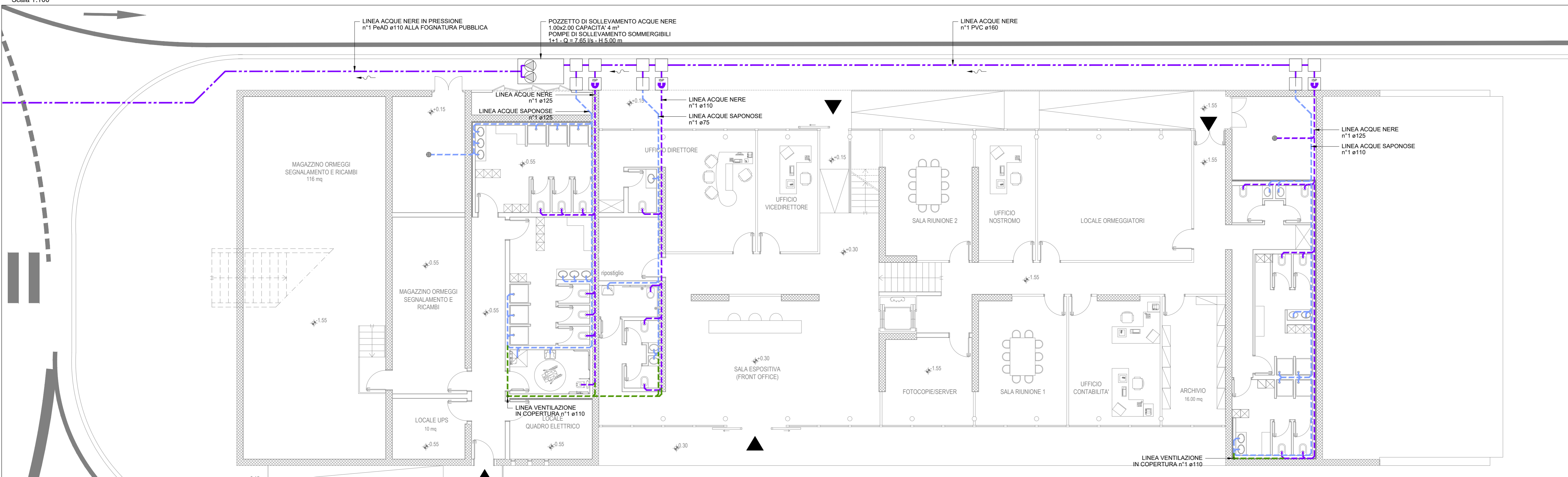
PIANTA PIANO TERRA - IMPIANTO IDRICO ED ANTINCENDIO Scala 1:100
