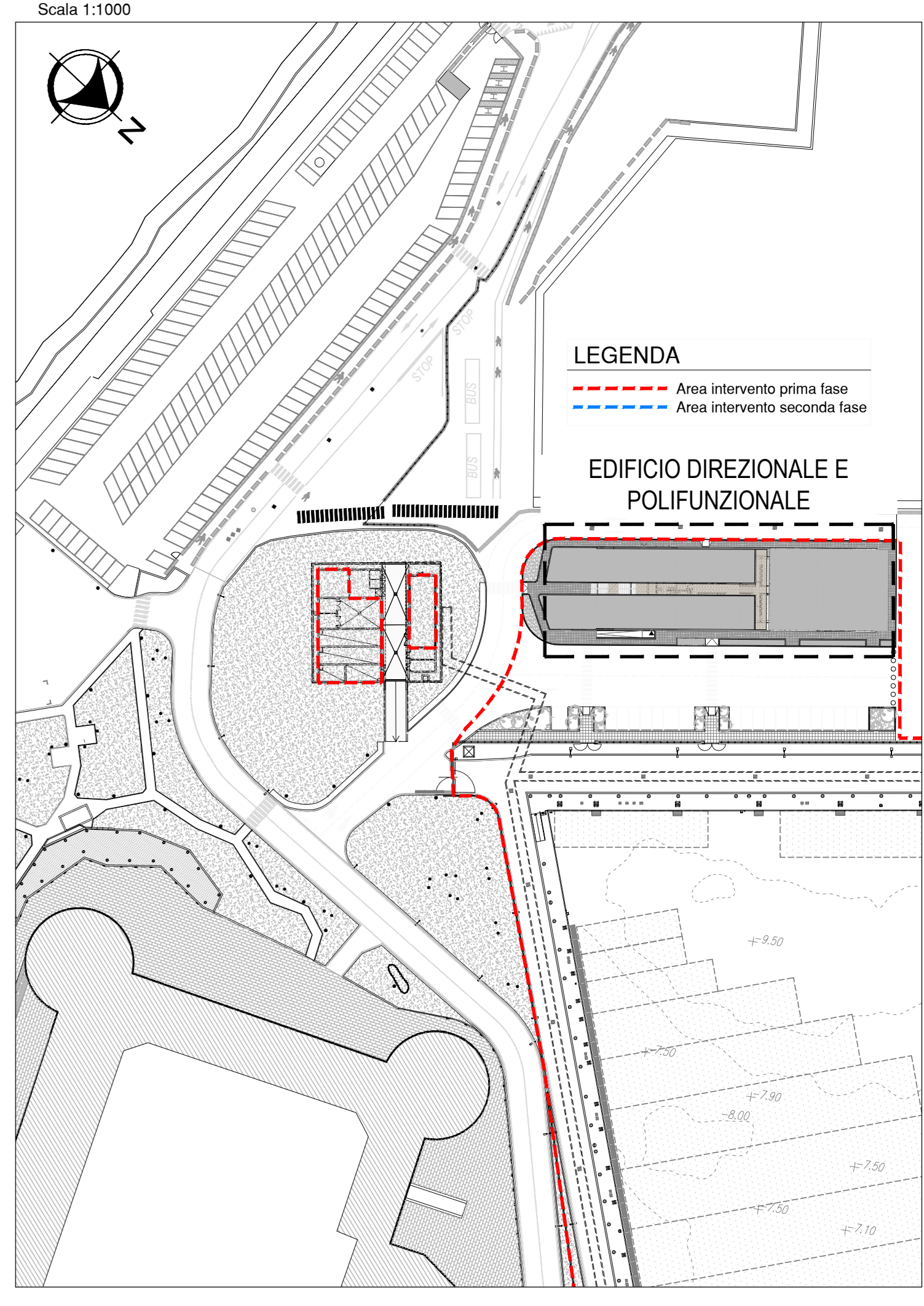
PLANIMETRIA GENERALE DI INQUADRAMENTO Scala 1:1000
