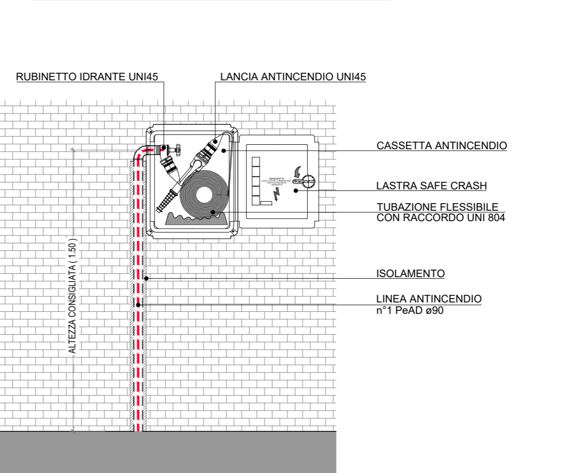
DETTAGLIO IDRANTE UN45 A CASSETTA
