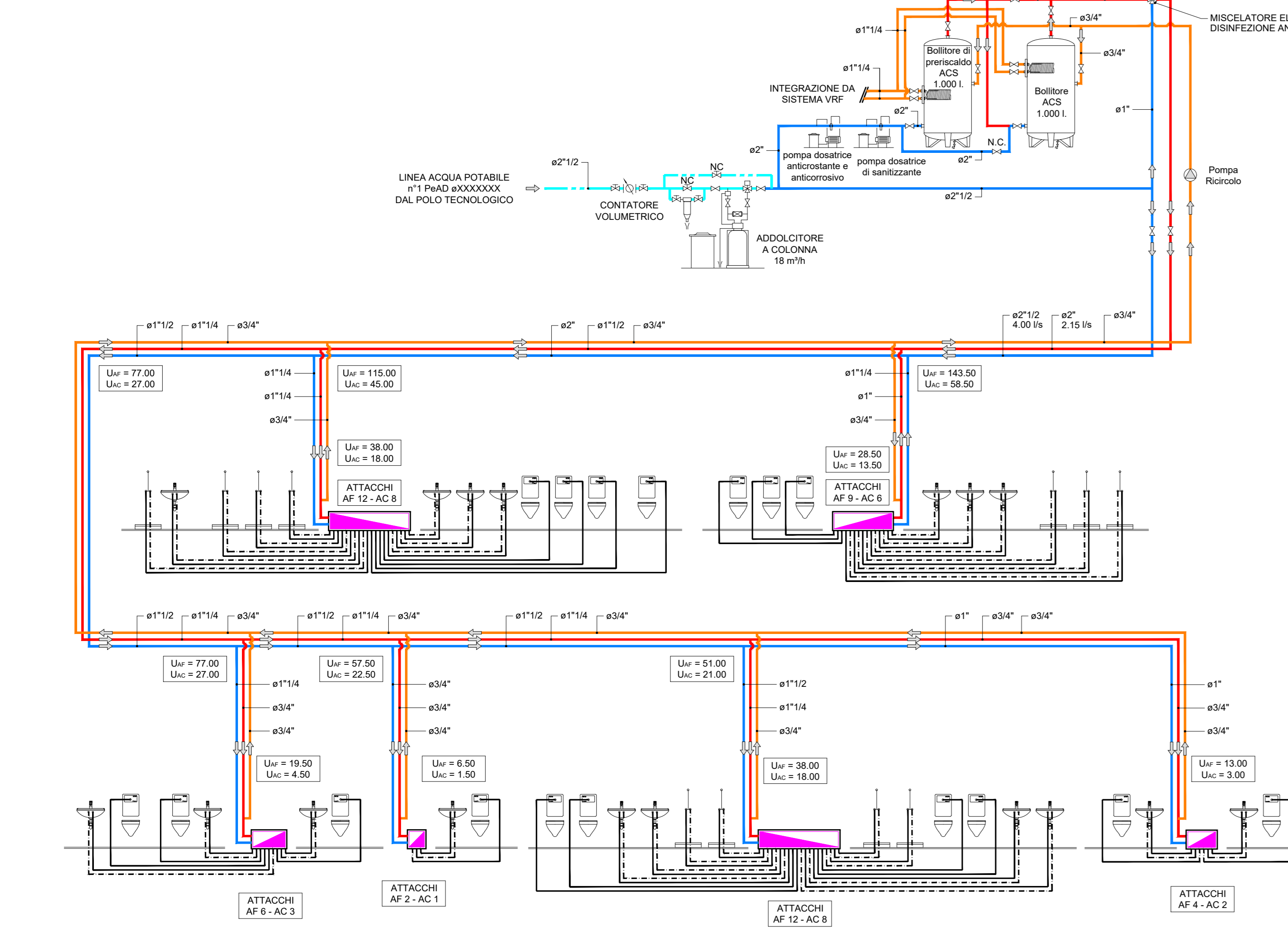
SCHEMA FUNZIONALE IMPIANTO IDRICO
