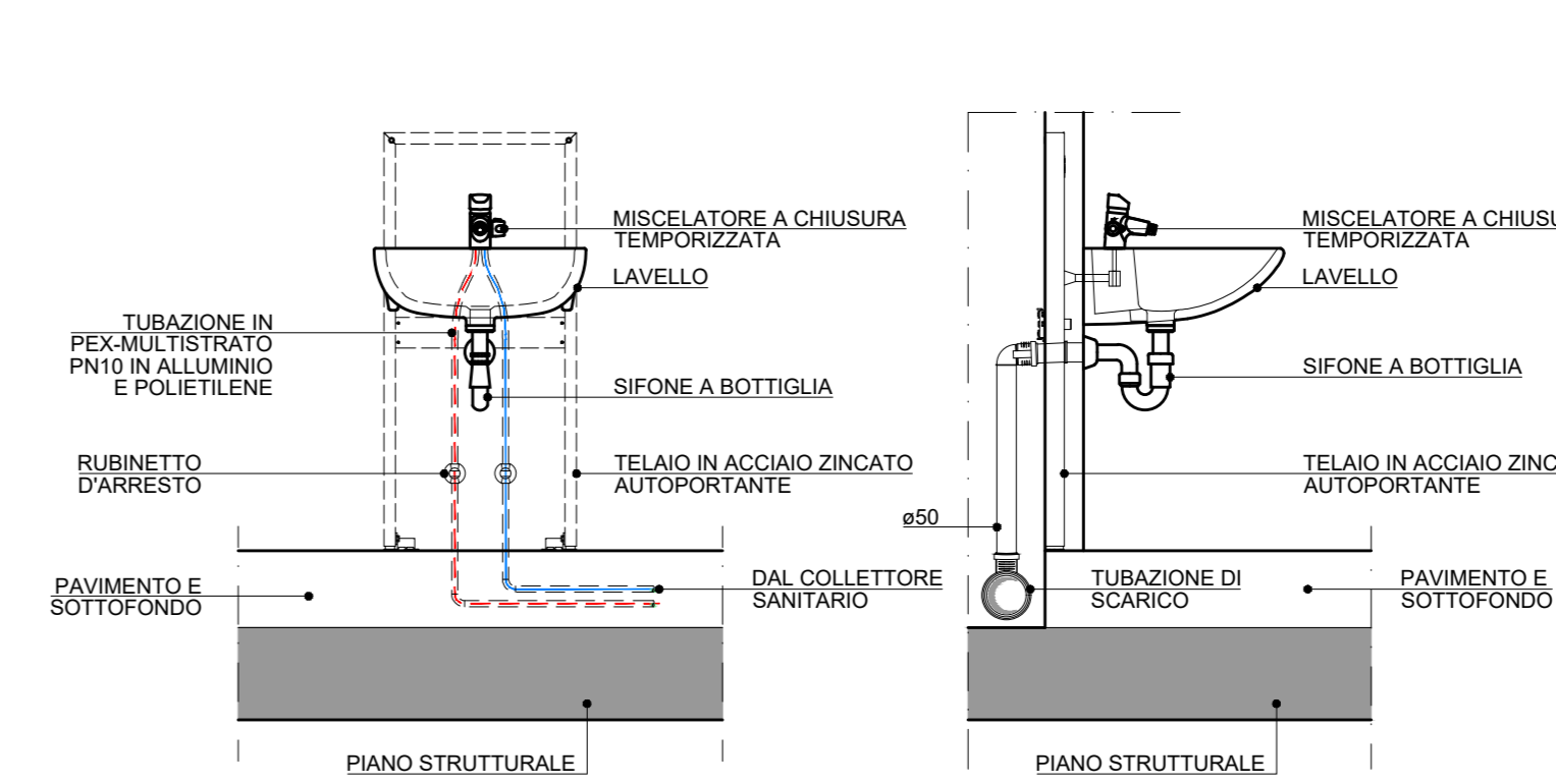
DETTAGLIO ALLACCIO E SCARICO LAVABO
