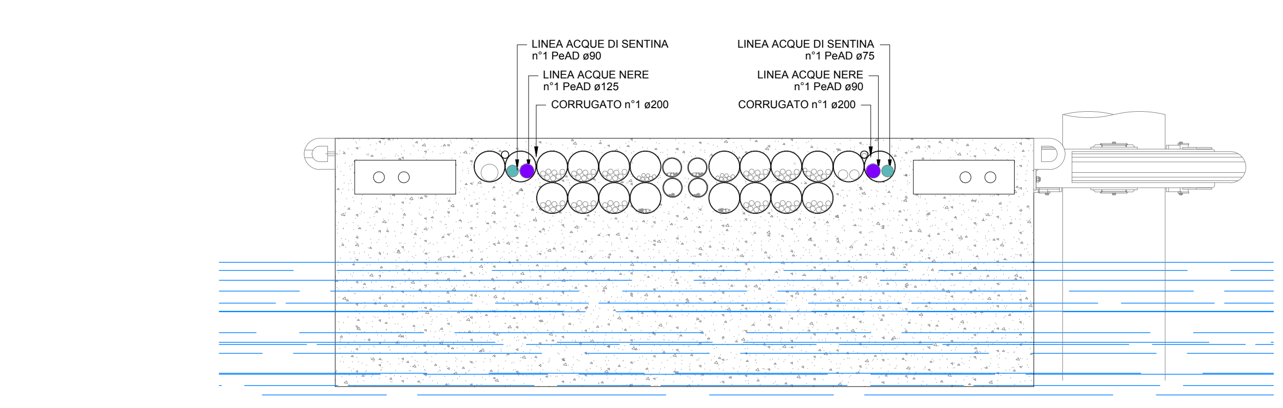
SEZIONE B-B Scala 1:25
