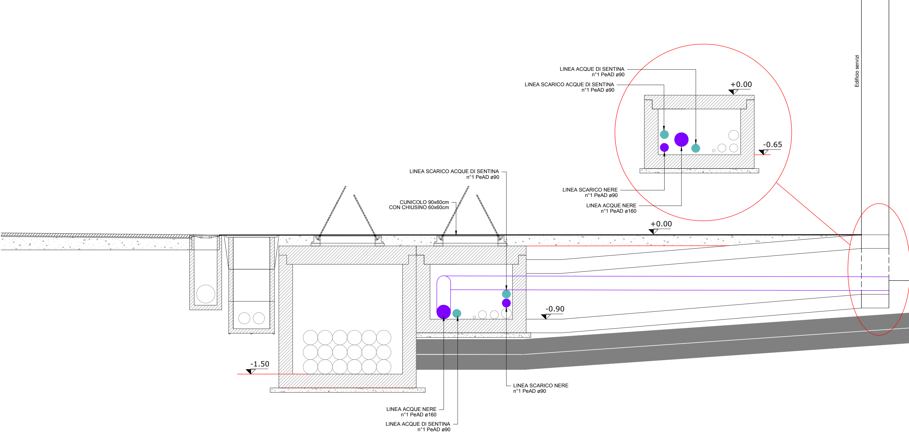
SEZIONE C-C Scala 1:25
