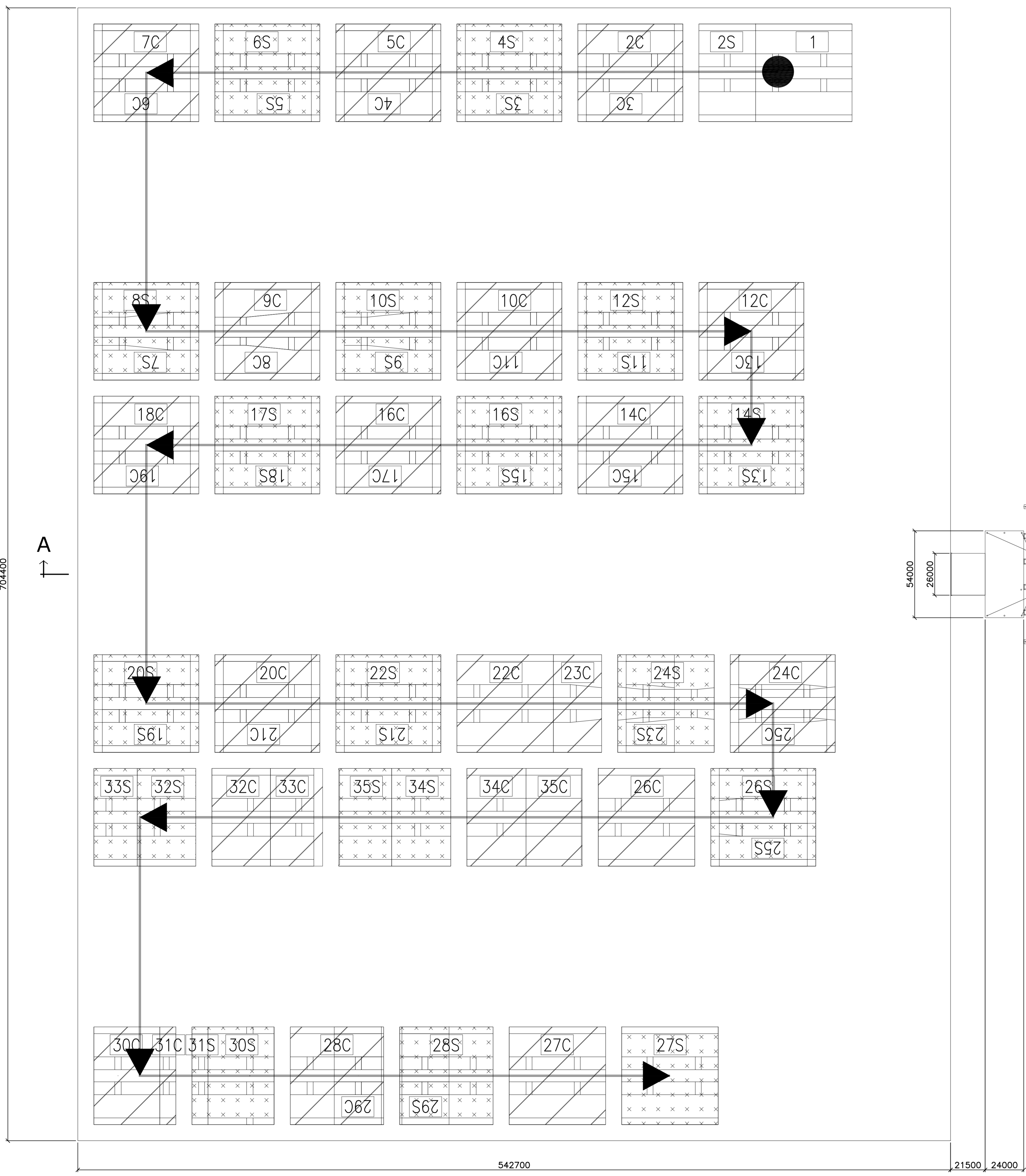
PIANTA AREA DI STOCCAGGIO CONCI DI IMPALCATO Scala 1:1250
