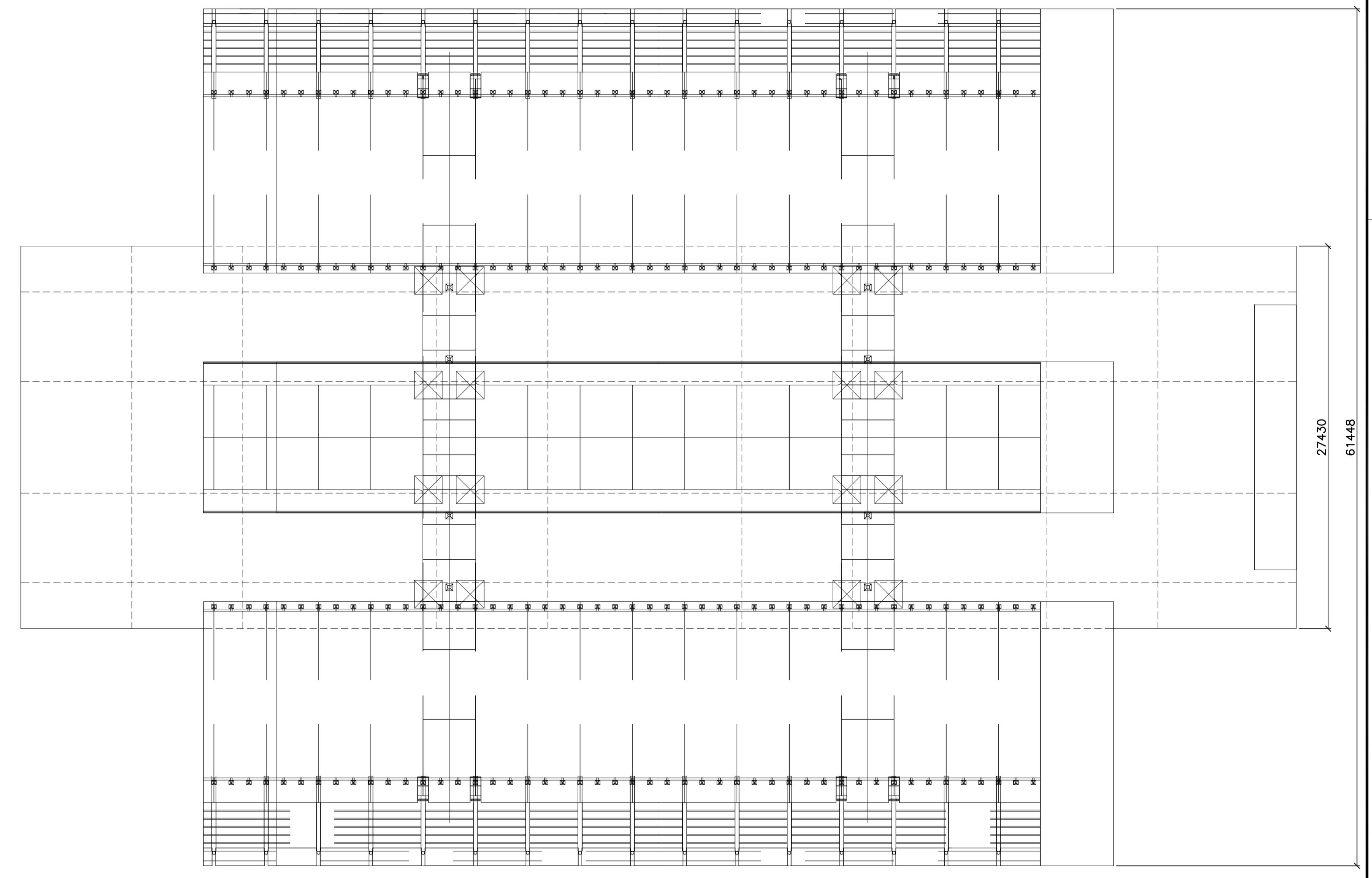
CONFIGURAZIONE DI TRASPORTO SU CHIATTA CONCIO TIPICO DI IMPALCATO Scala 1:200
