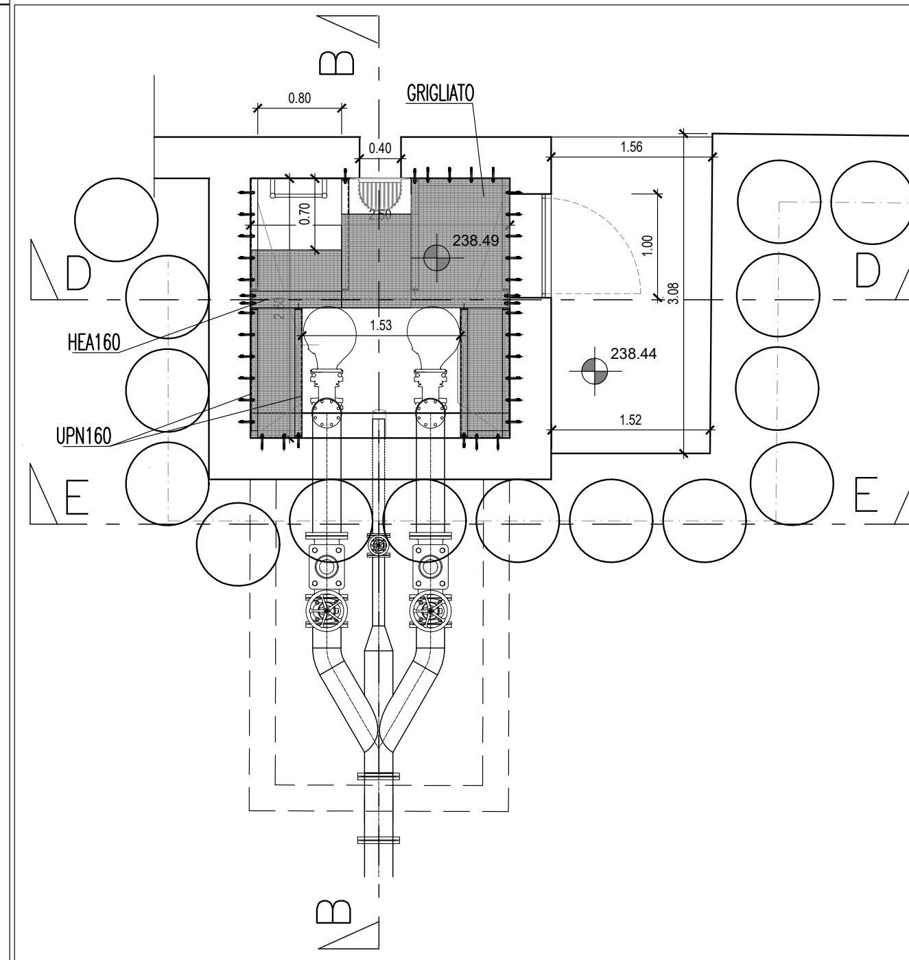
PIANTA A QUOTA 238.49 - 1:50
