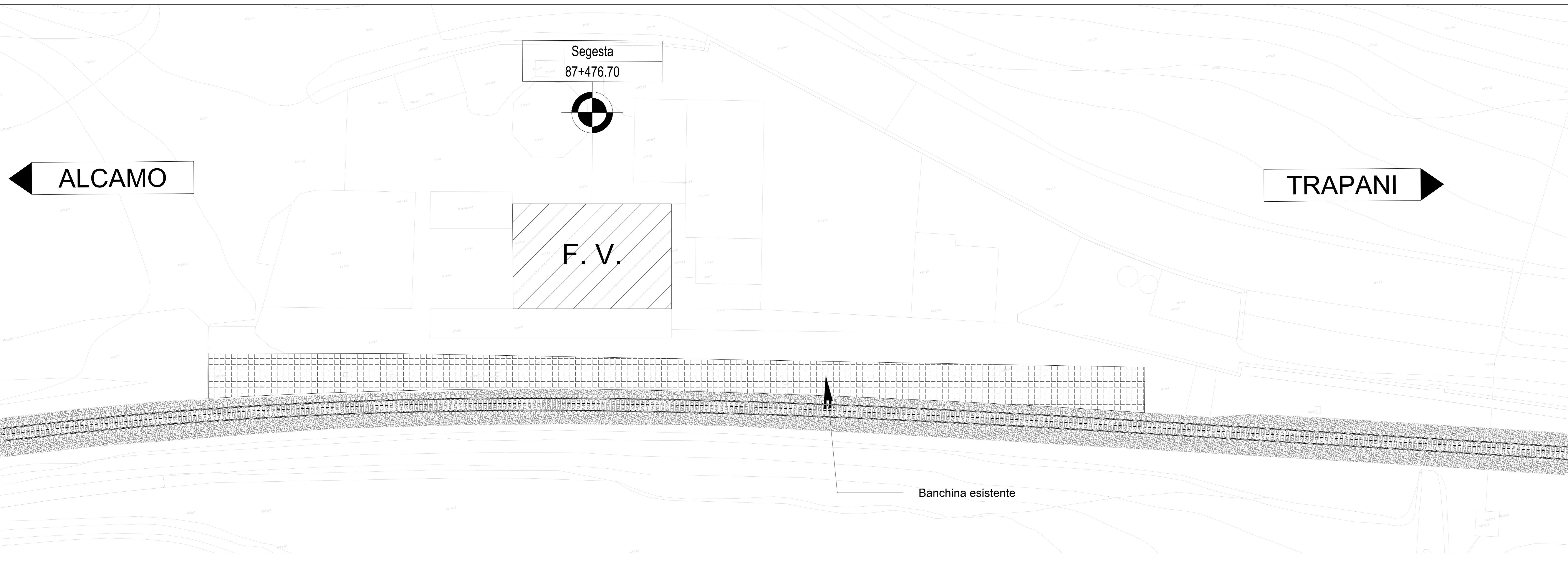
PLANIMETRIA STATO DI FATTO 1:200
