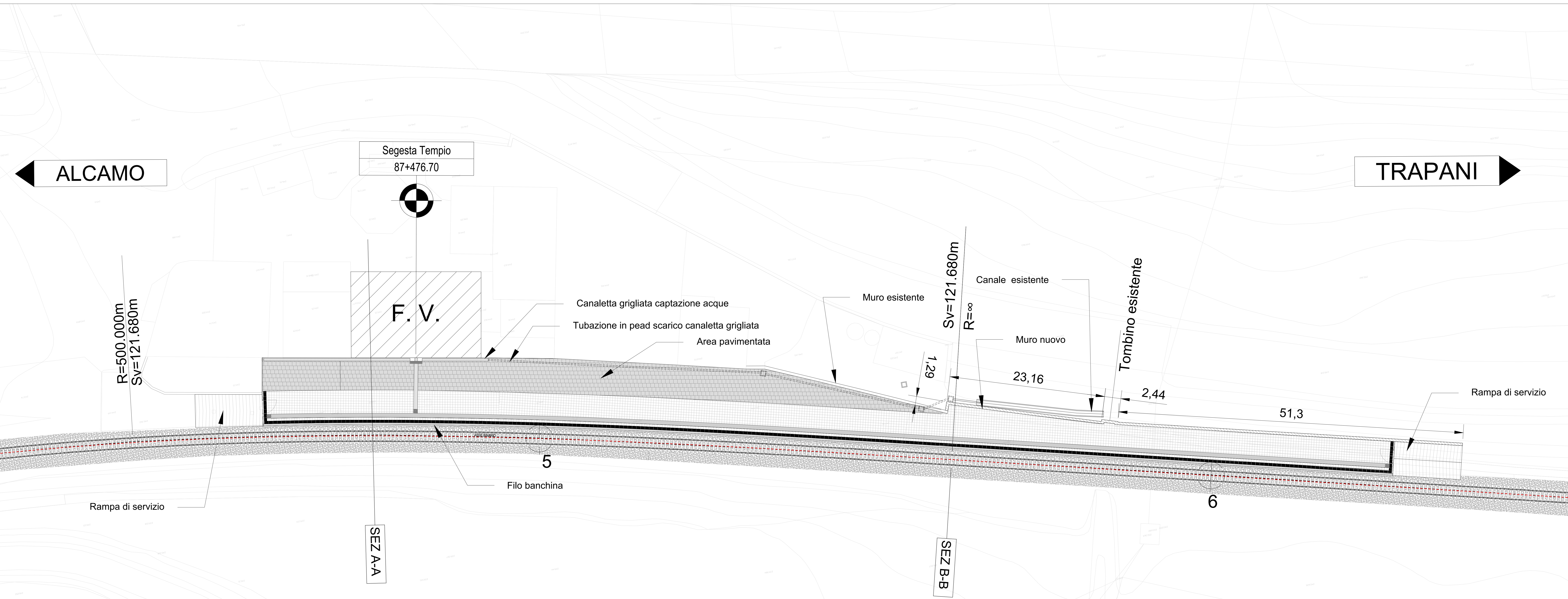
PLANIMETRIA STATO DI FATTO 1:200
