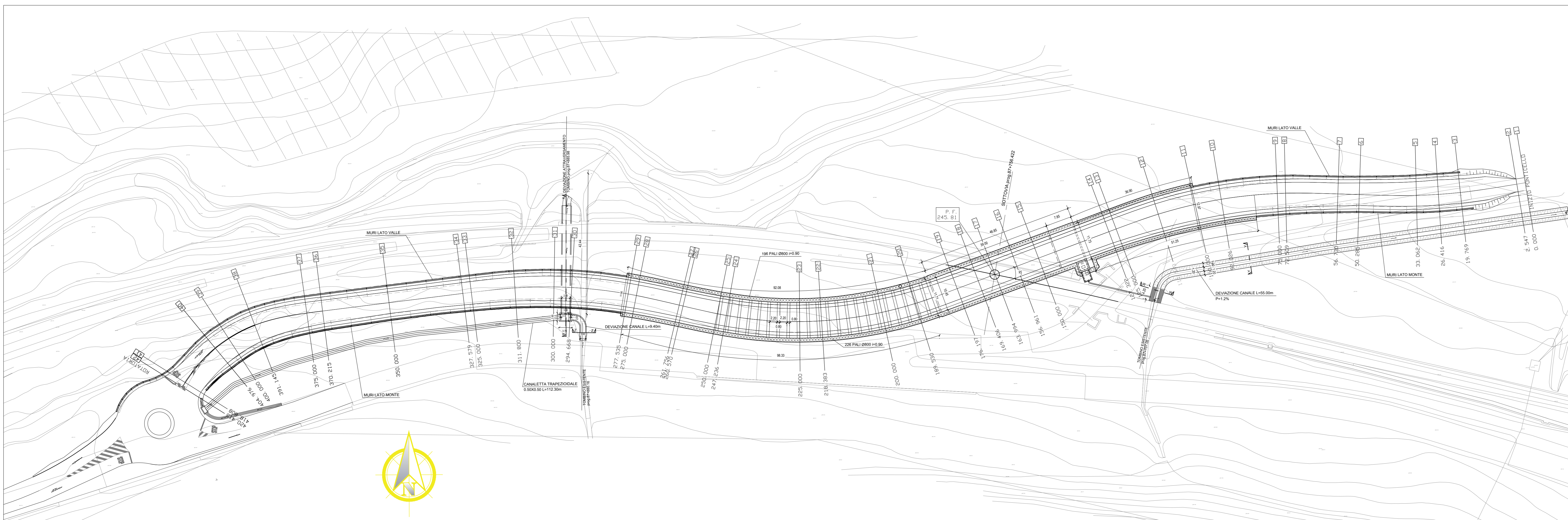
STRALCIO PLANIMETRICO SOTTOVIA SEGESTA ALLA Prog.87+756.422 - 1:500
