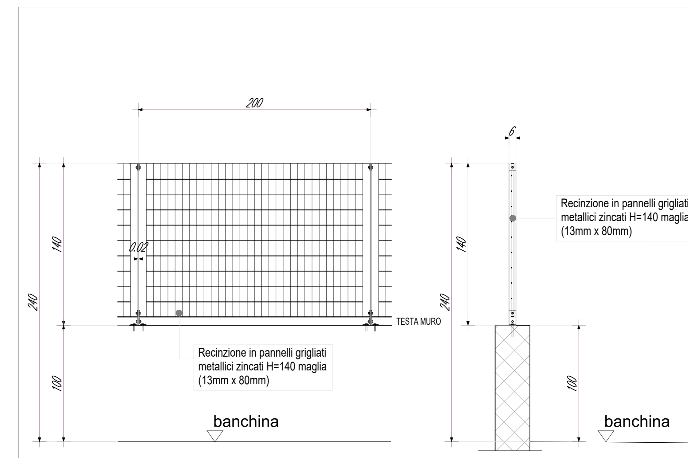
DETTAGLIO RECINZIONE 1:20
