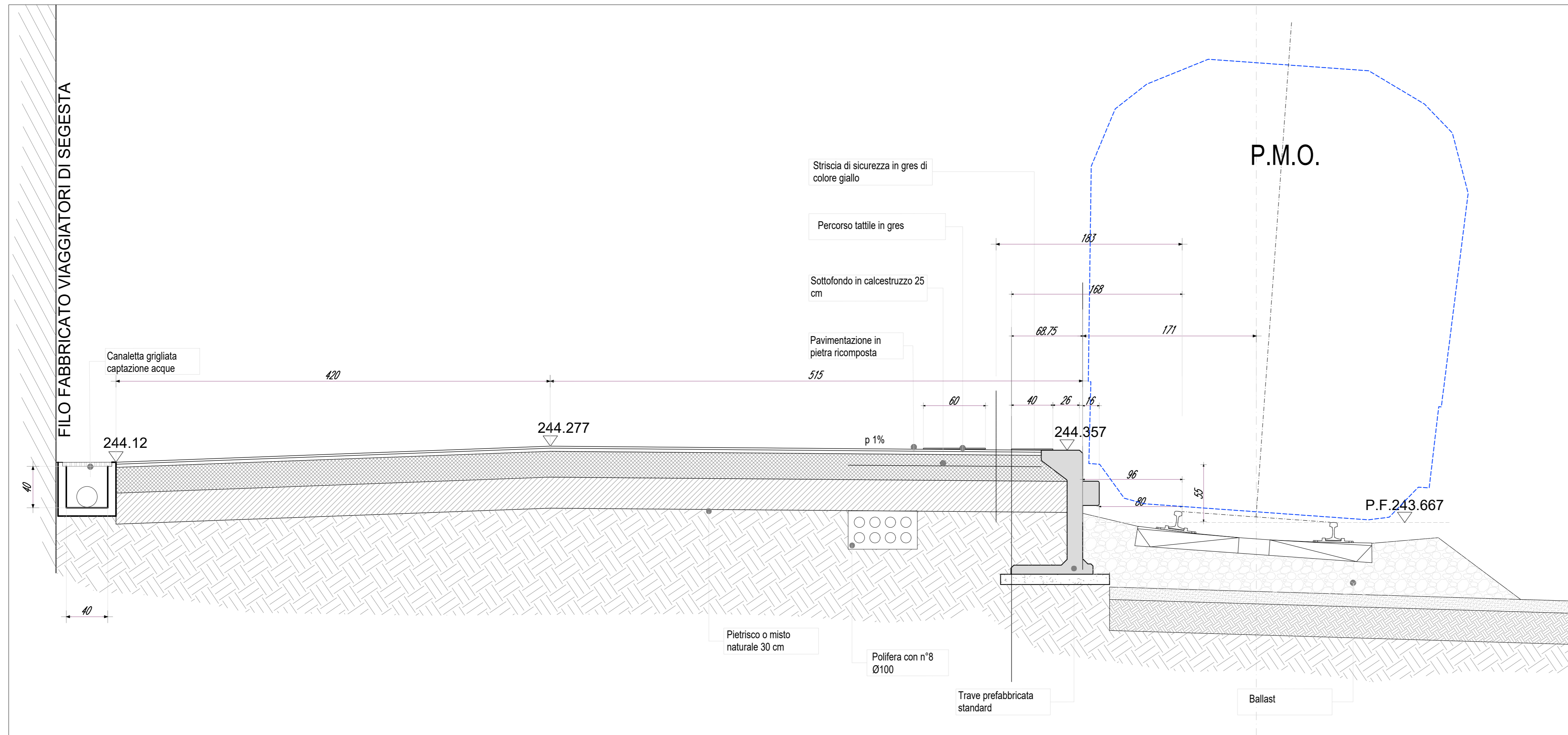
SEZIONE A-A 1:20
