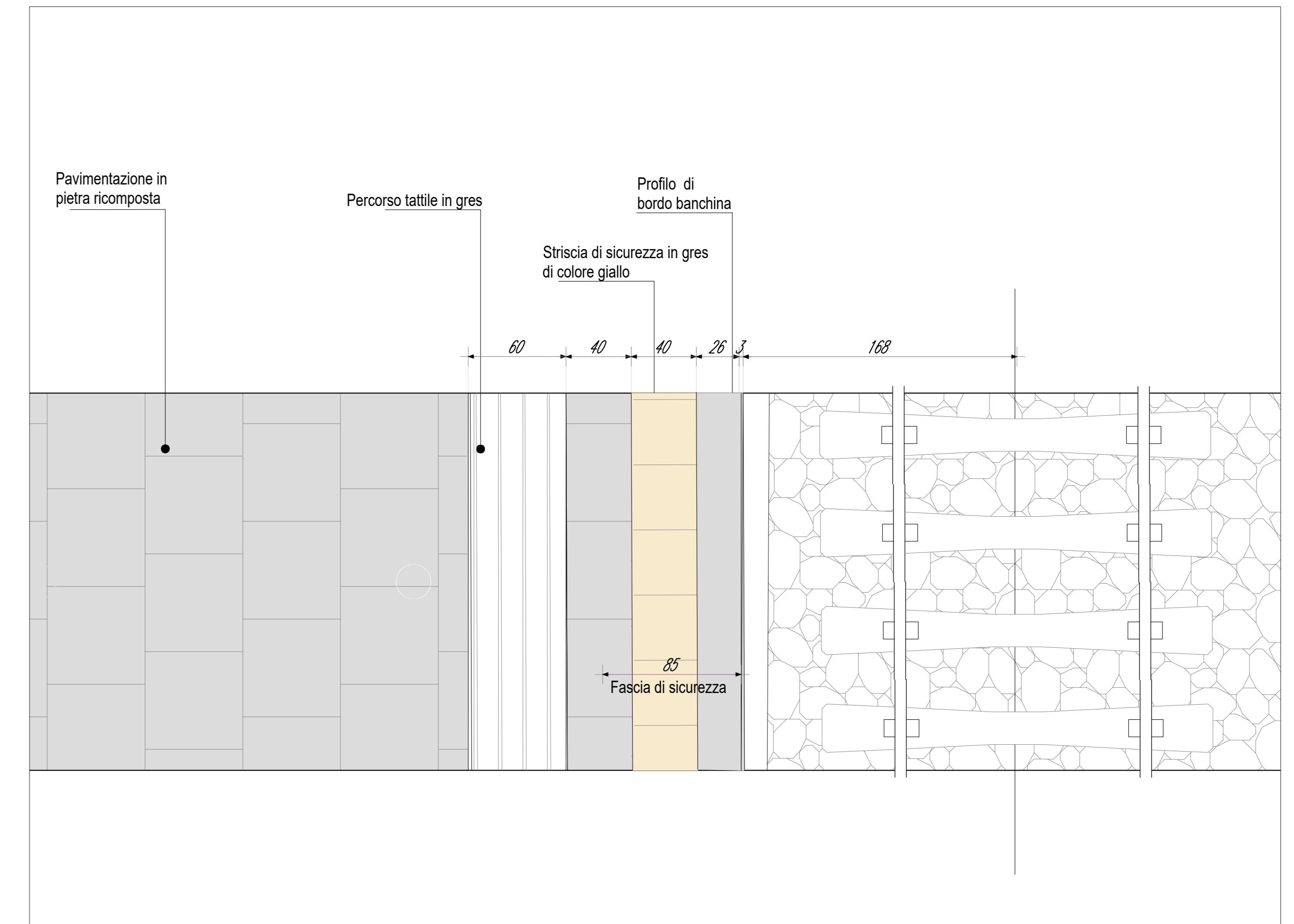
PIANTA PAVIMENTAZIONE BANCHINA 1:20
