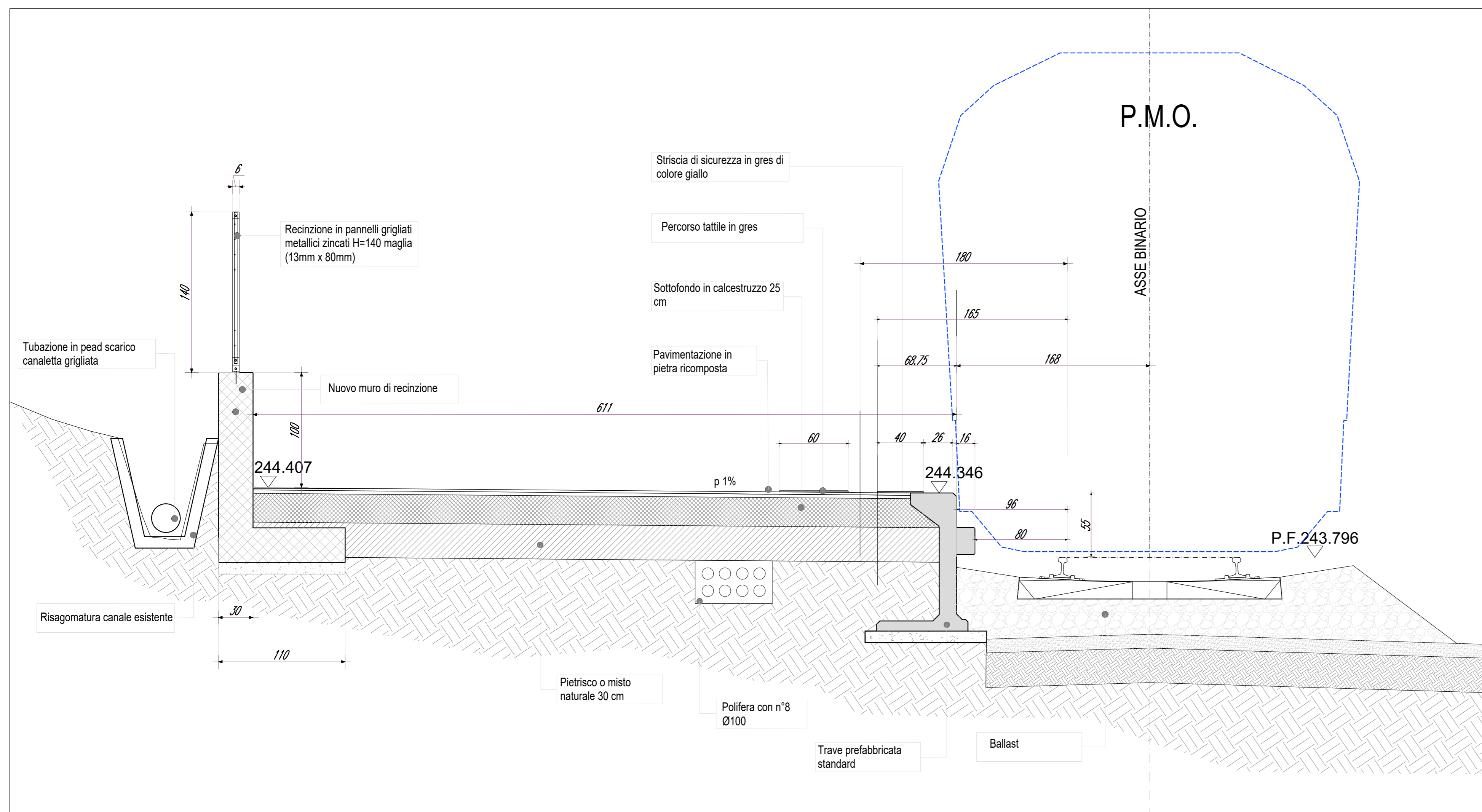
SEZIONE B-B 1:20
