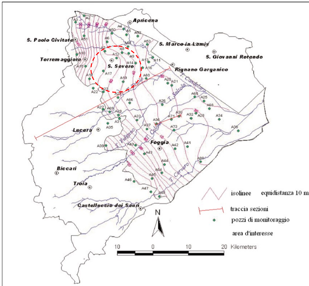
Fig. 5: Carta della piezometria gennaio-febbraio 2003 (Masciale R. 2004) modificata
