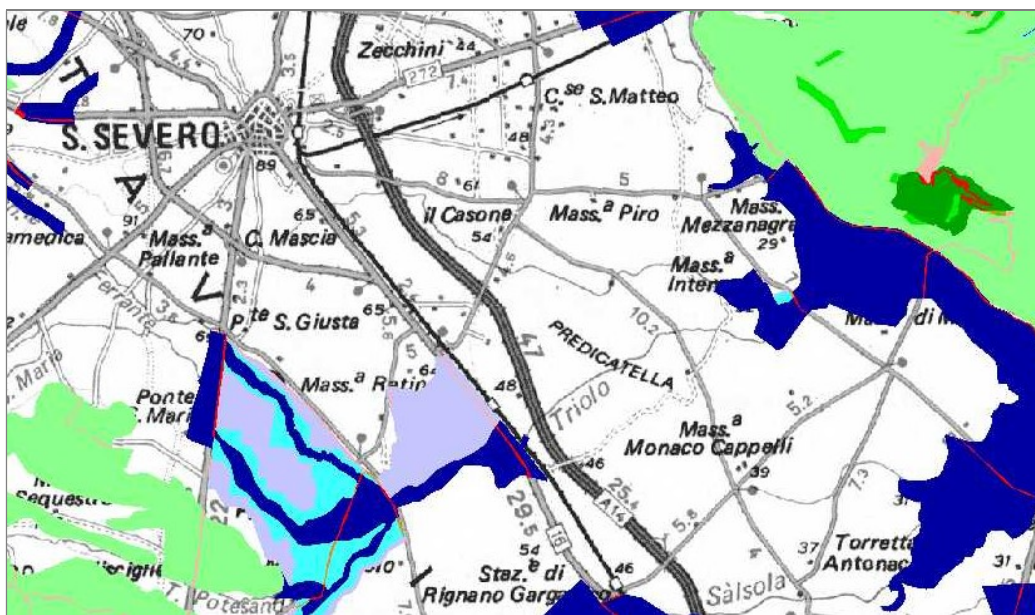
Fig 7: Aree sottoposte a vincolo P.A.I. - AdB Regione Puglia
