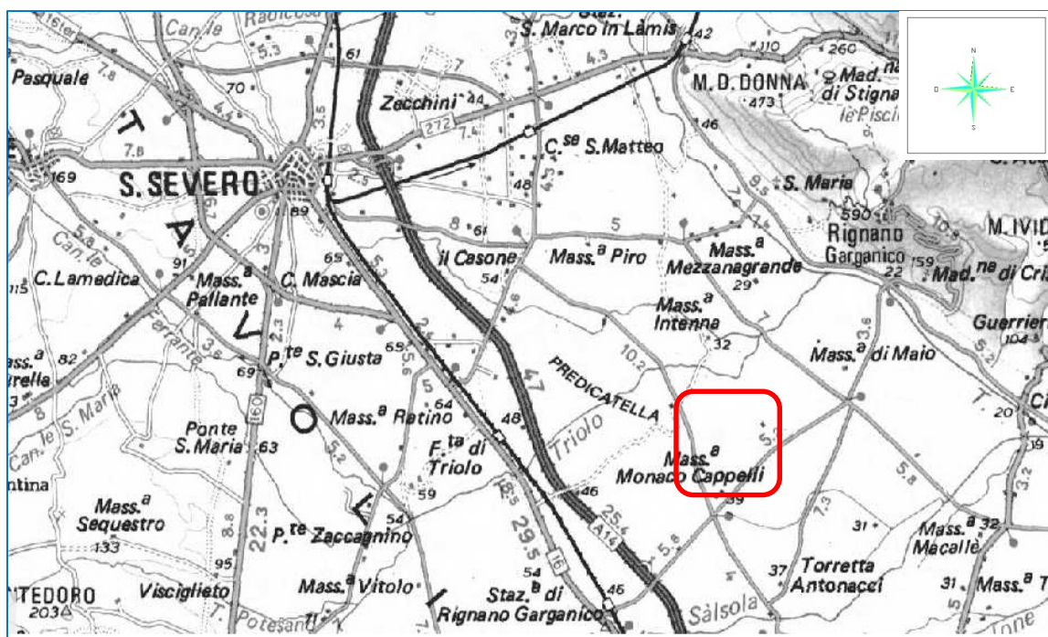
Fig. 1: Corografia IGM (non in scala) con indicazione dell'area d'intervento
