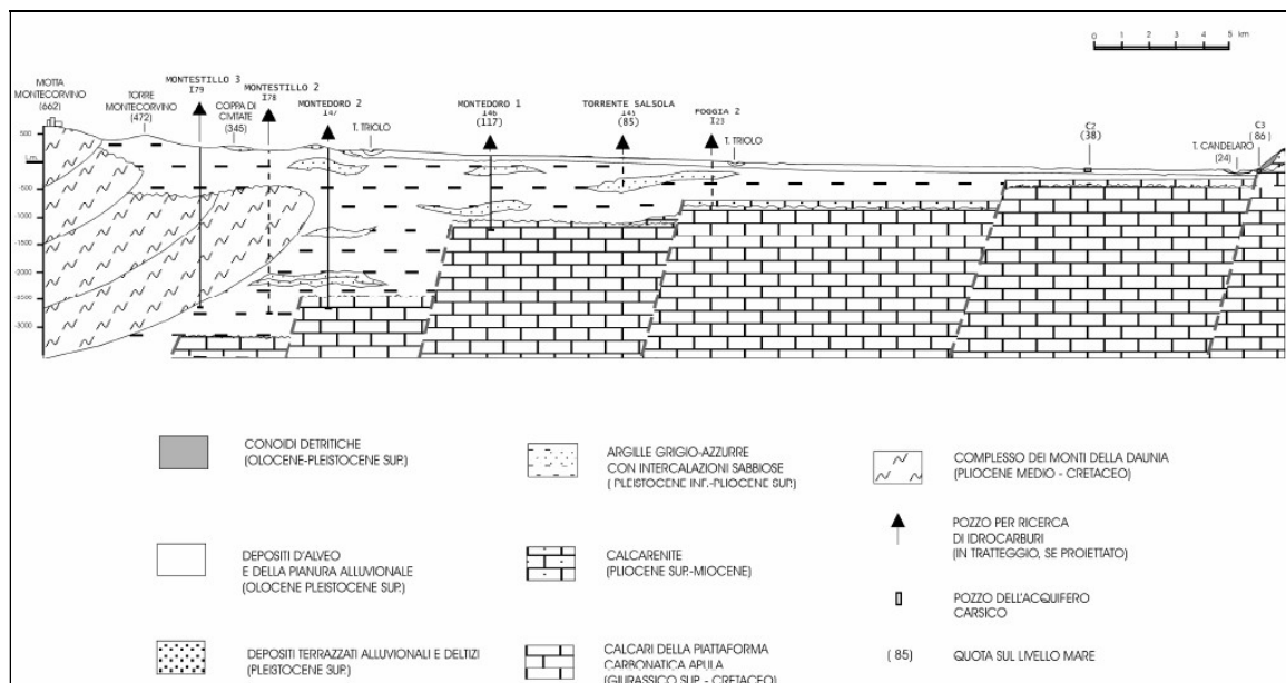
Fig. 4: Sezione geologica da Motta monte Corvino a Rignano Garganico.
