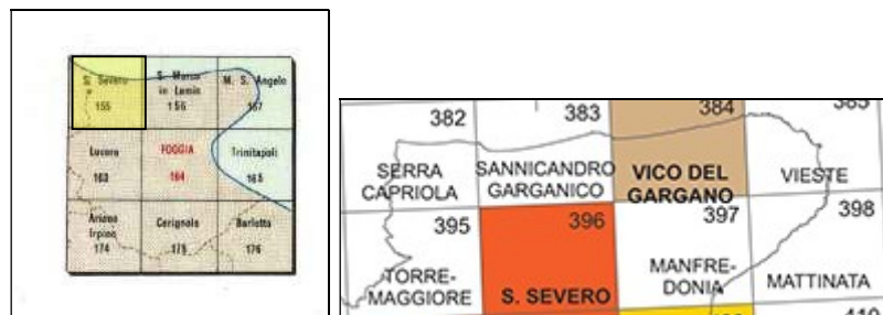
Fig. n. 3: Ubicazione geologica dell'area
