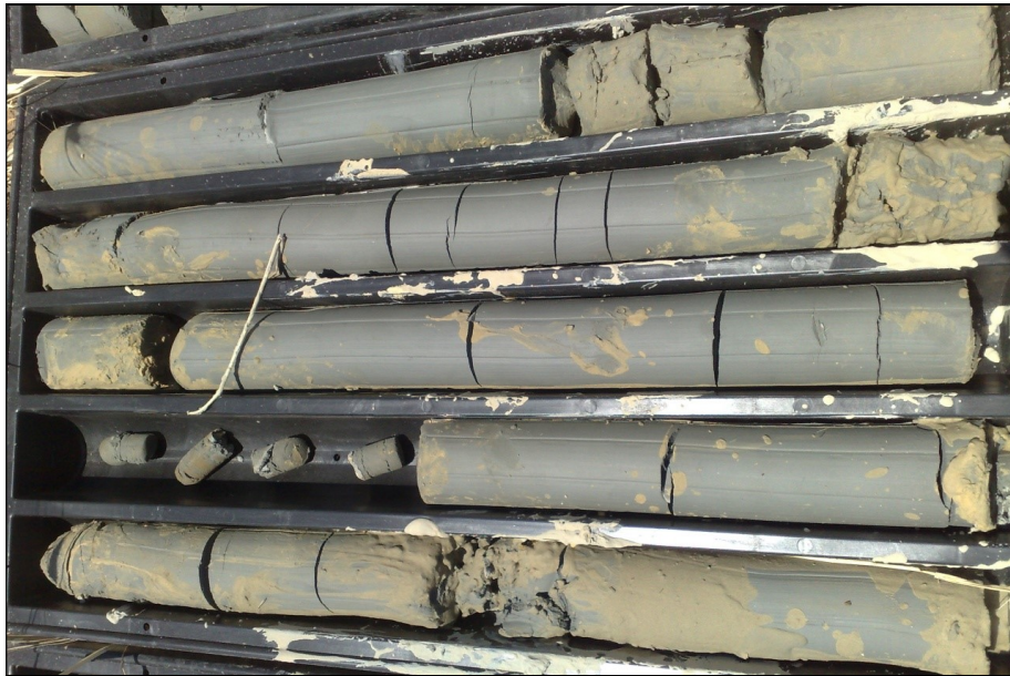
Sondaggio S1: da 20 m a 25 m
