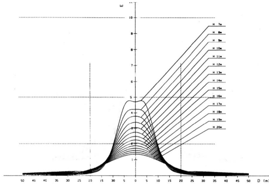
Fig. 1 Andamento tipico del campo di induzione magnetica.
