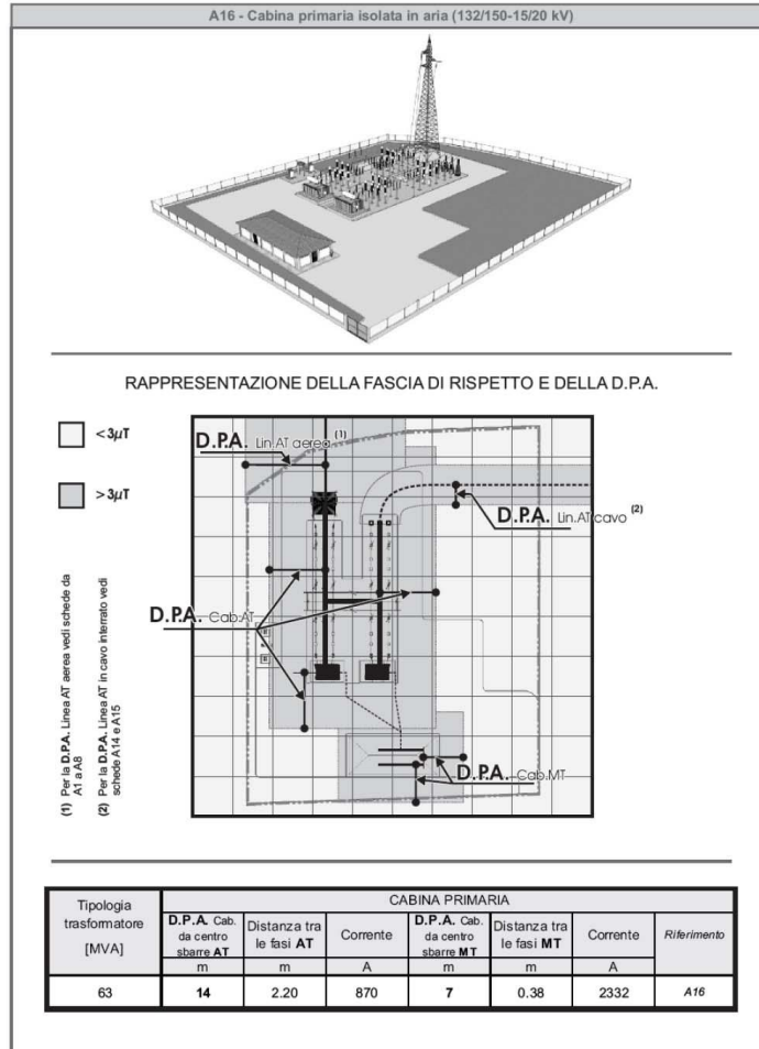
Fig. 2 - Fascia di rispetto cabina primaria 150kV. Fonte: ENEL
