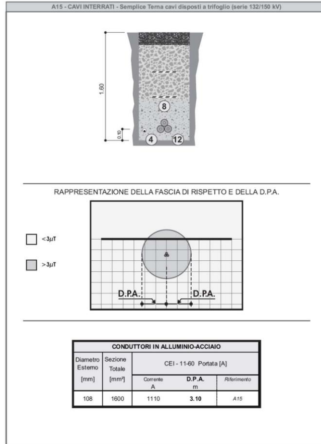
Fig. 1 - Fascia di rispetto cavi interrati 150kV. Fonte: ENEL
