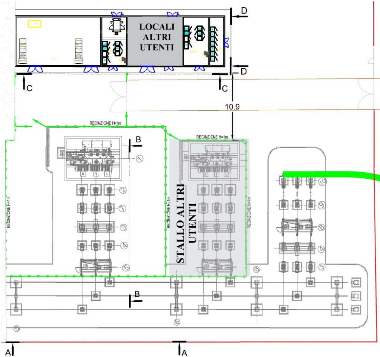
Fig. 2 – Layout in SSE Produttore in corso di autorizzazione.
