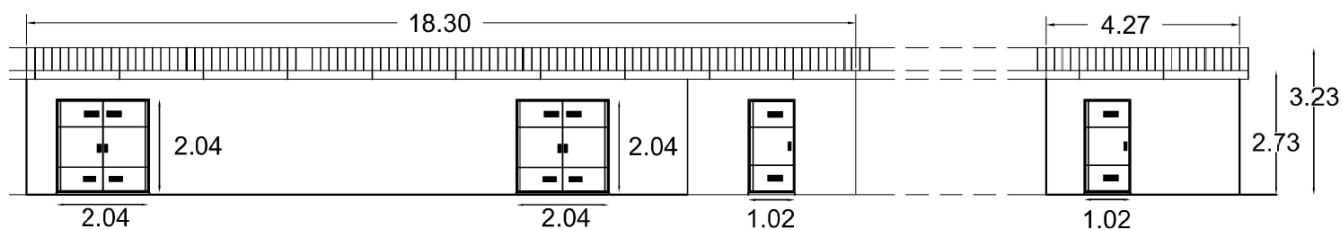
Fig. 3 – Prospetto fabbricato tecnologico.
