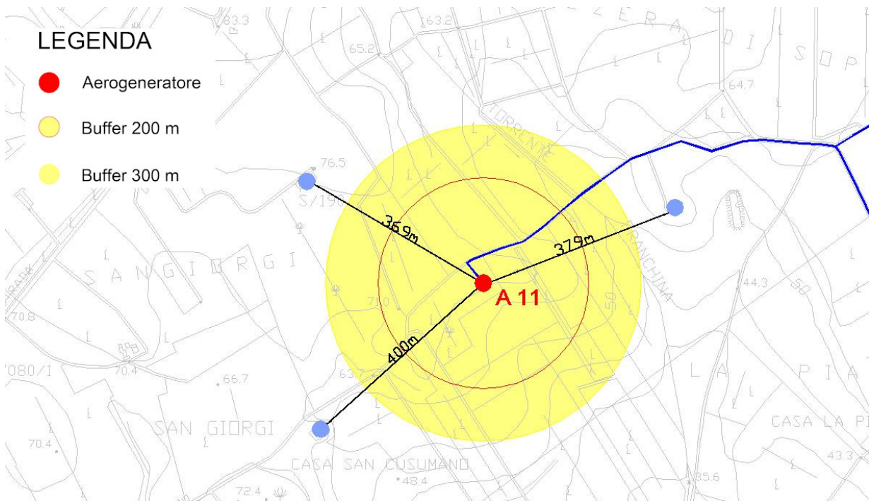
Individuazione aerogeneratori 11 con distanza dei fabbricati rilevati più vicini
