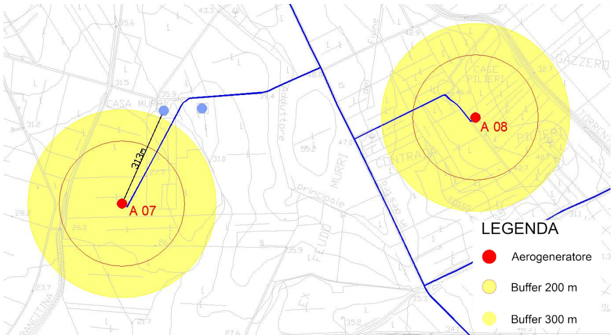
Individuazione aerogeneratori 07 – 08 con distanza dei fabbricati rilevati più vicini
