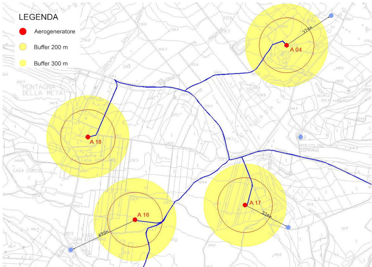
Individuazione aerogeneratori 06 – 16 – 17 – 18 con distanza dei fabbricati rilevati più vicini
