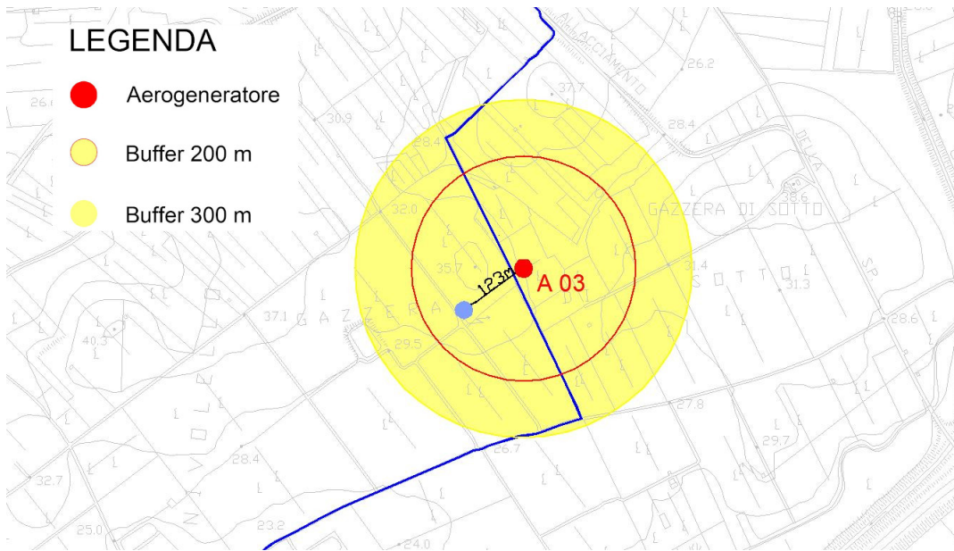
Individuazione aerogeneratori 03 con distanza dei fabbricati rilevati più vicini
