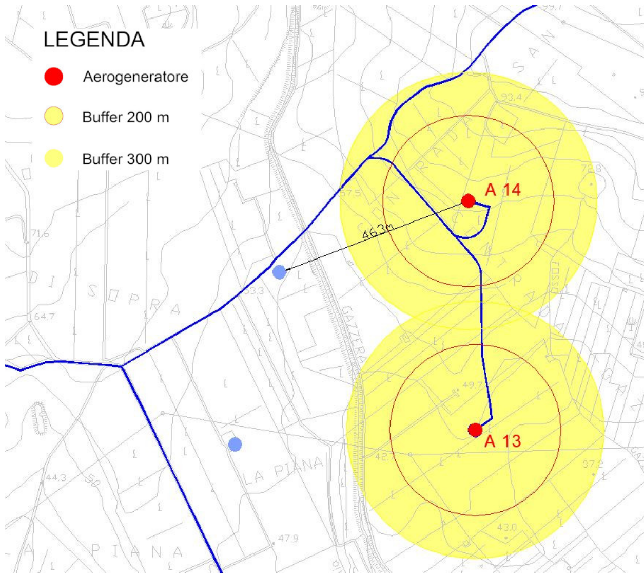
Individuazione aerogeneratori 14 - 13 con distanza dei fabbricati rilevati più vicini
