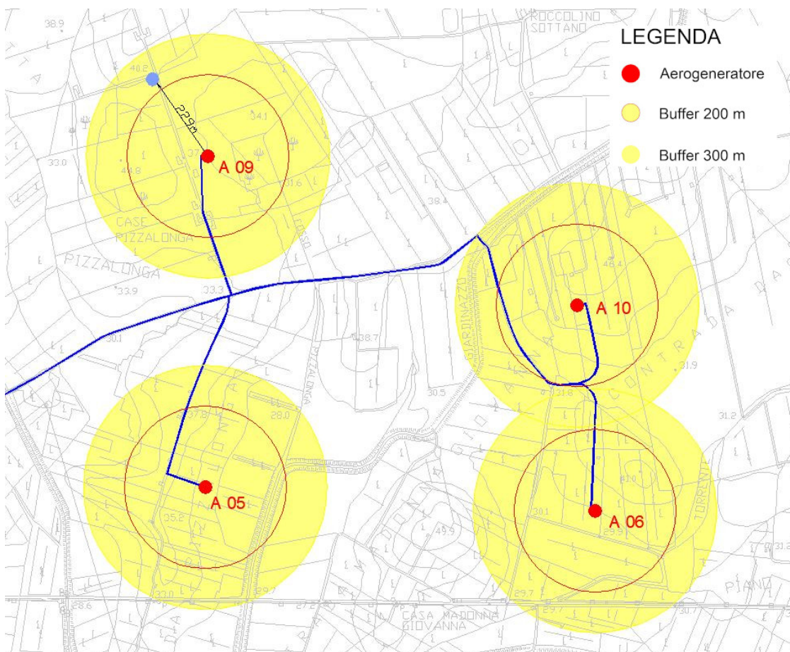
Individuazione aerogeneratori 05 – 06 – 09 – 10 con distanza dei fabbricati rilevati più vicini
