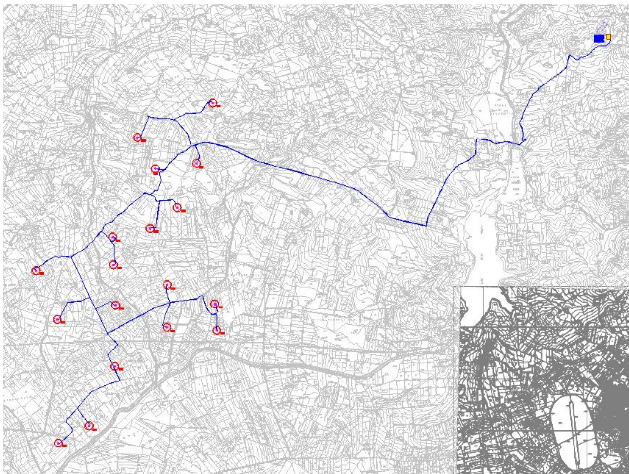
Layout di impianto su Carta Tecnica Regionale
