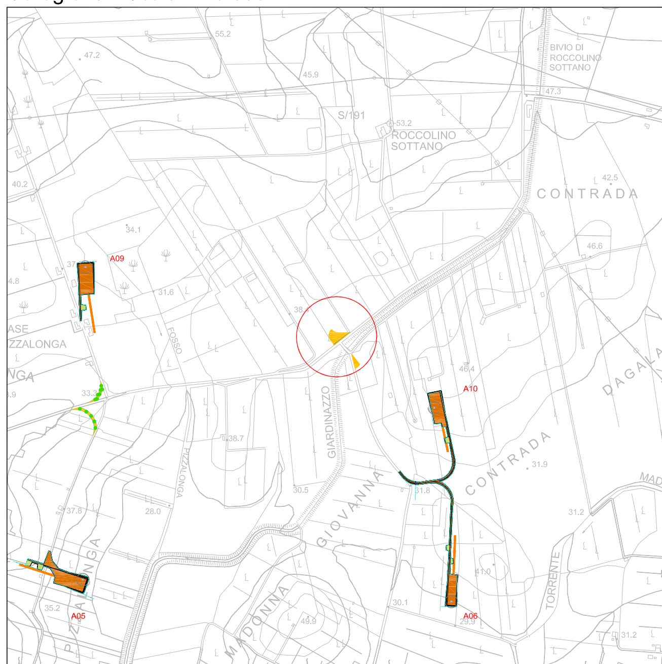
Corografia - Scala 1:10.000
