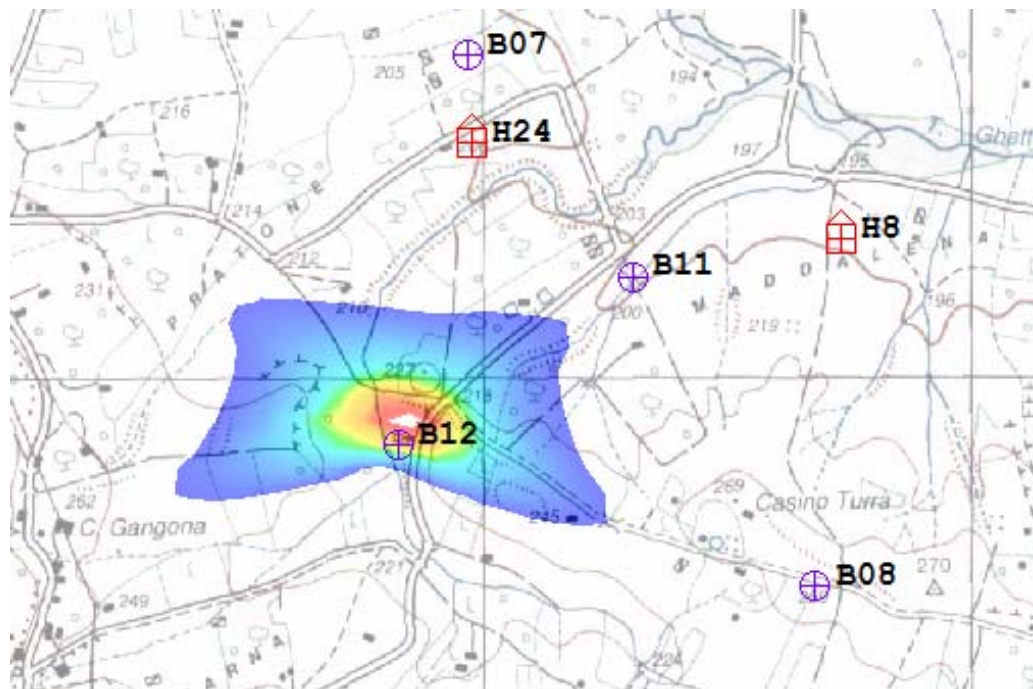
Figura 9: mappa di impatto potenziale per l'aerogeneratore 12
