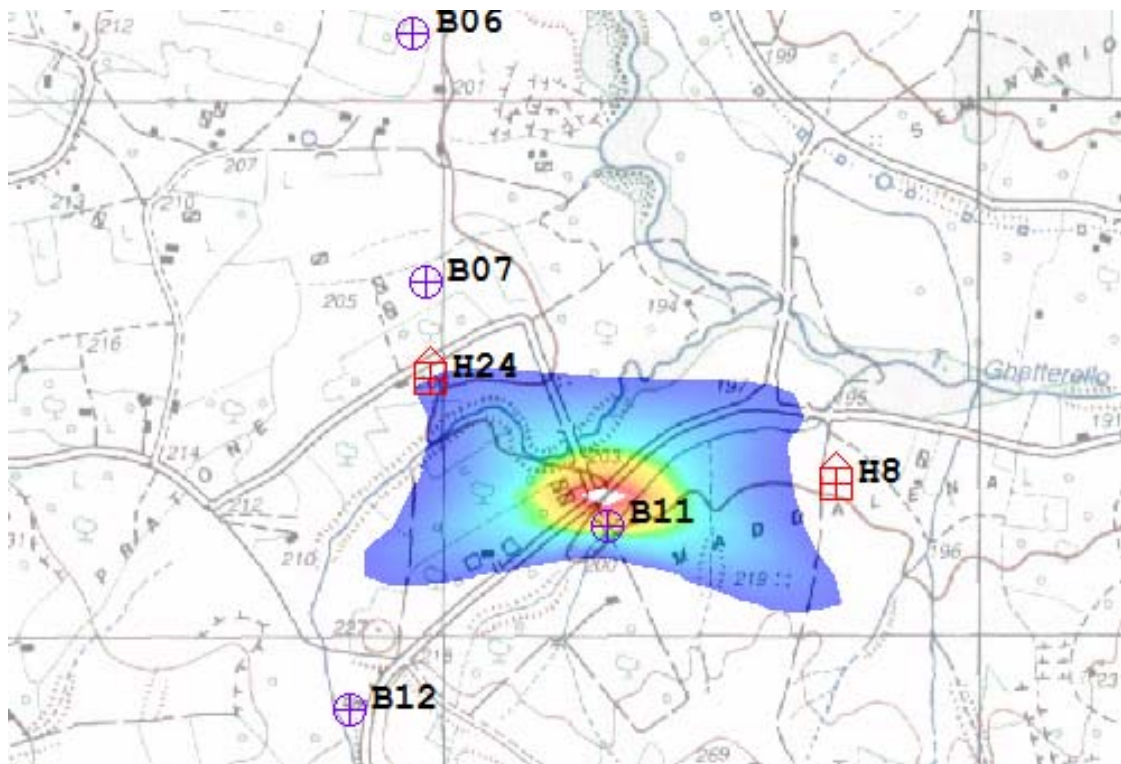
Figura 8: mappa di impatto potenziale per l'aerogeneratore 11
