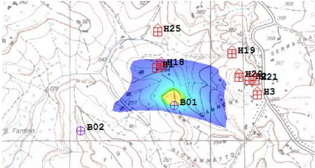
Figura 3: mappa di impatto potenziale per l'aerogeneratore 1
