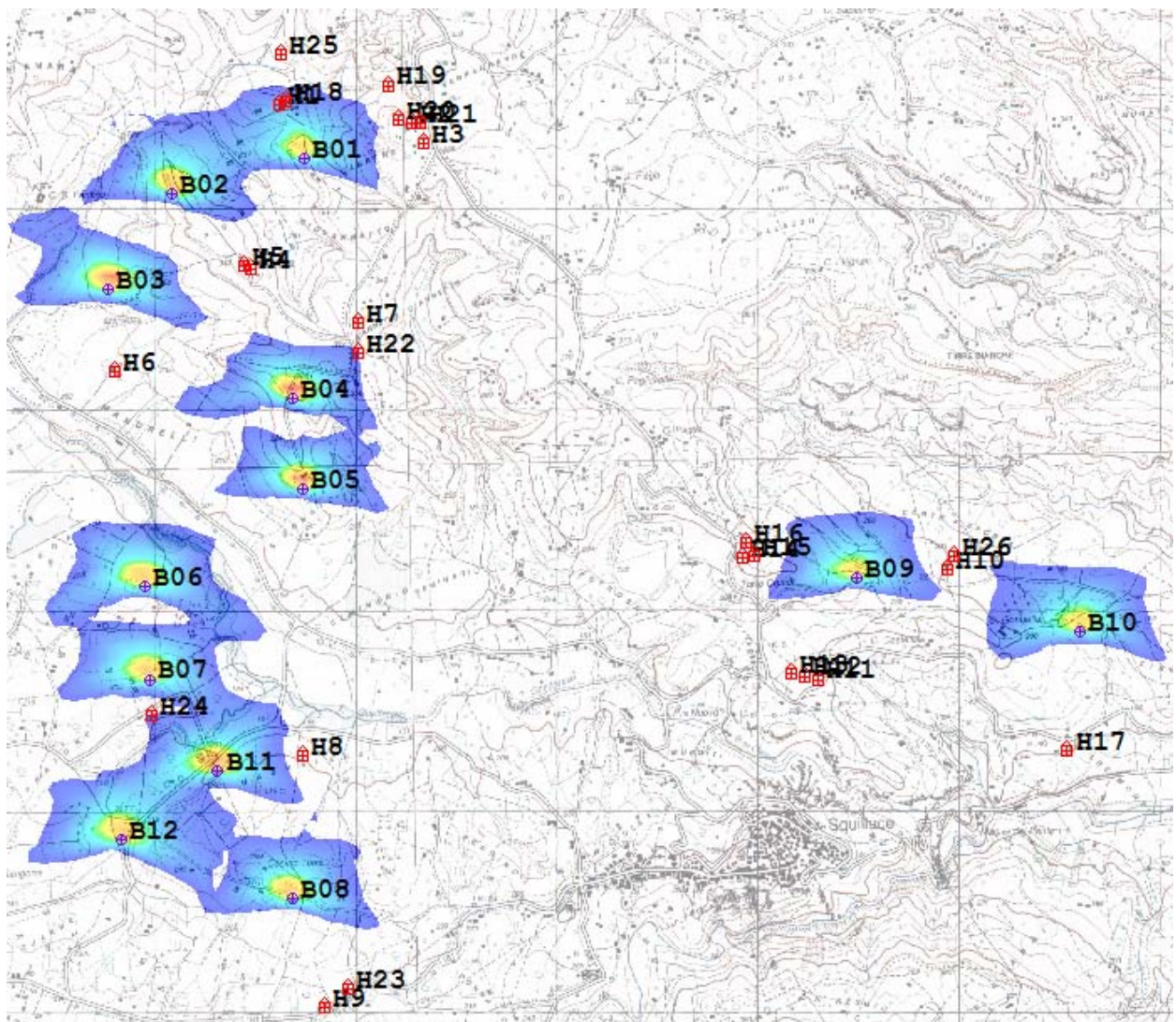
Figura 2: mappa di impatto potenziale (stralcio) da shadow flickering per il campo eolico in esame
