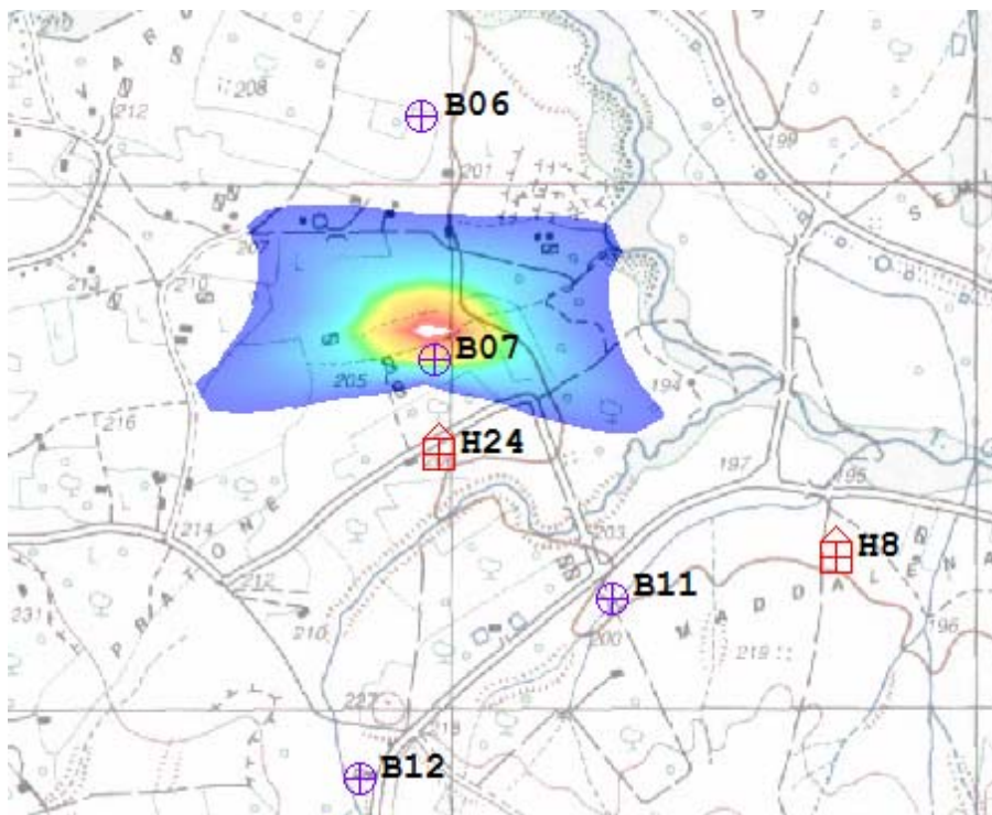
Figura 6: mappa di impatto potenziale per l'aerogeneratore 7
