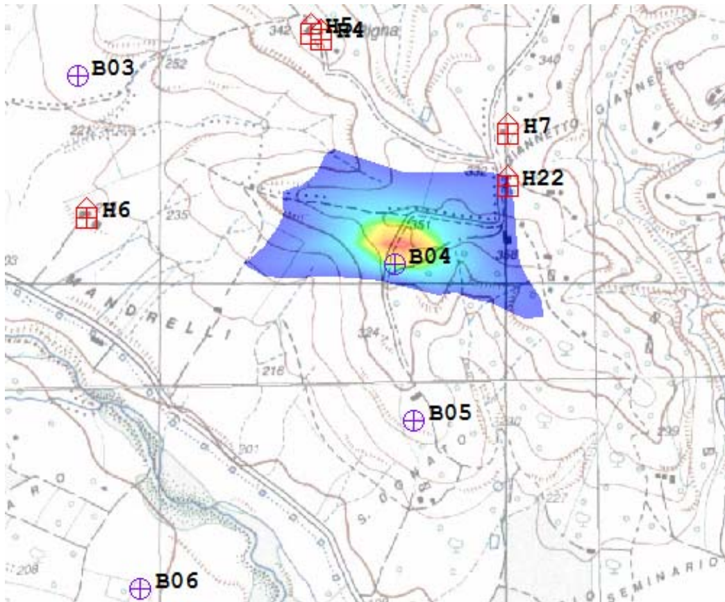
Figura 5: mappa di impatto potenziale per l'aerogeneratore 4
