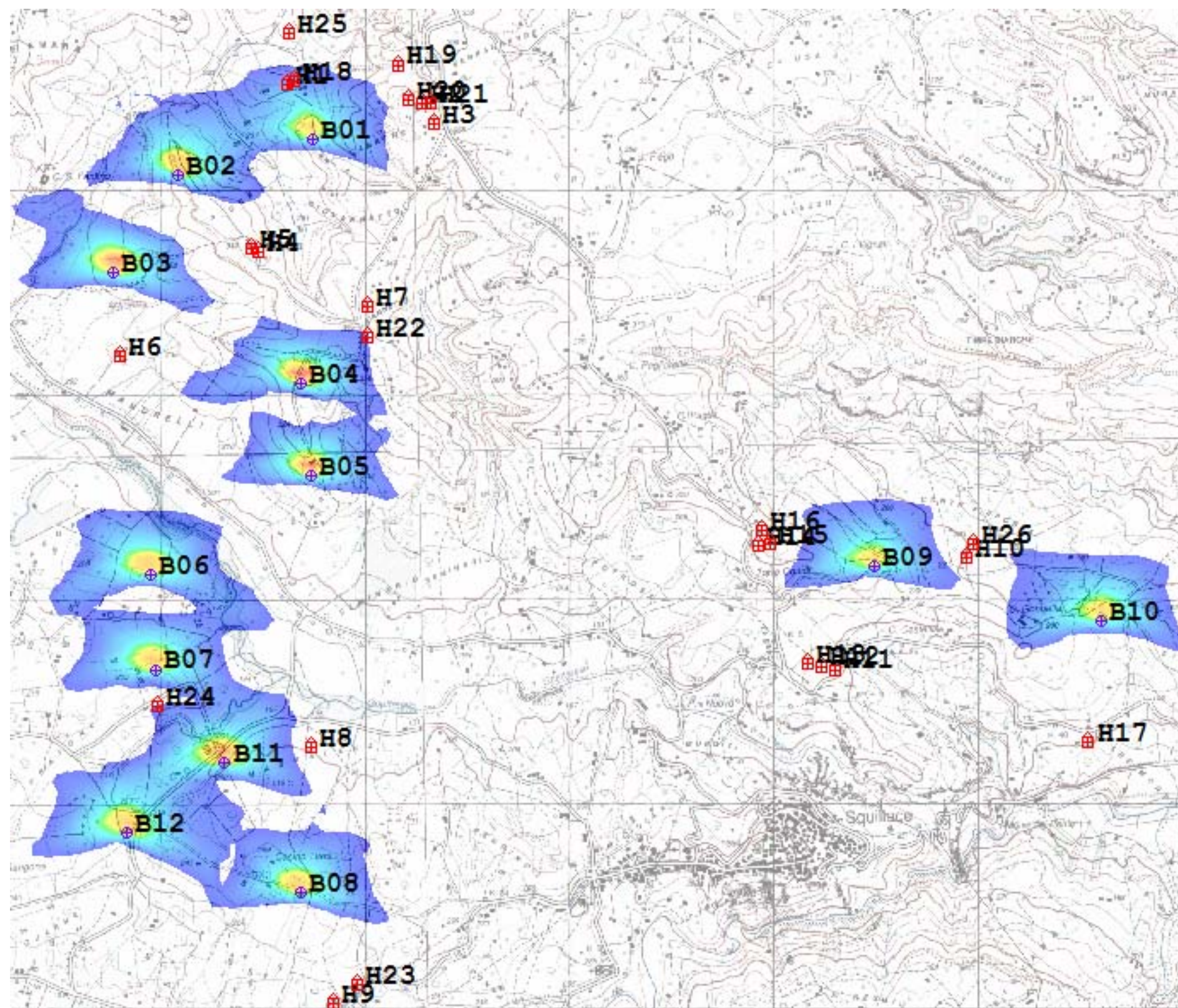
Figura 10: mappa di shadow flickering su base IGM
