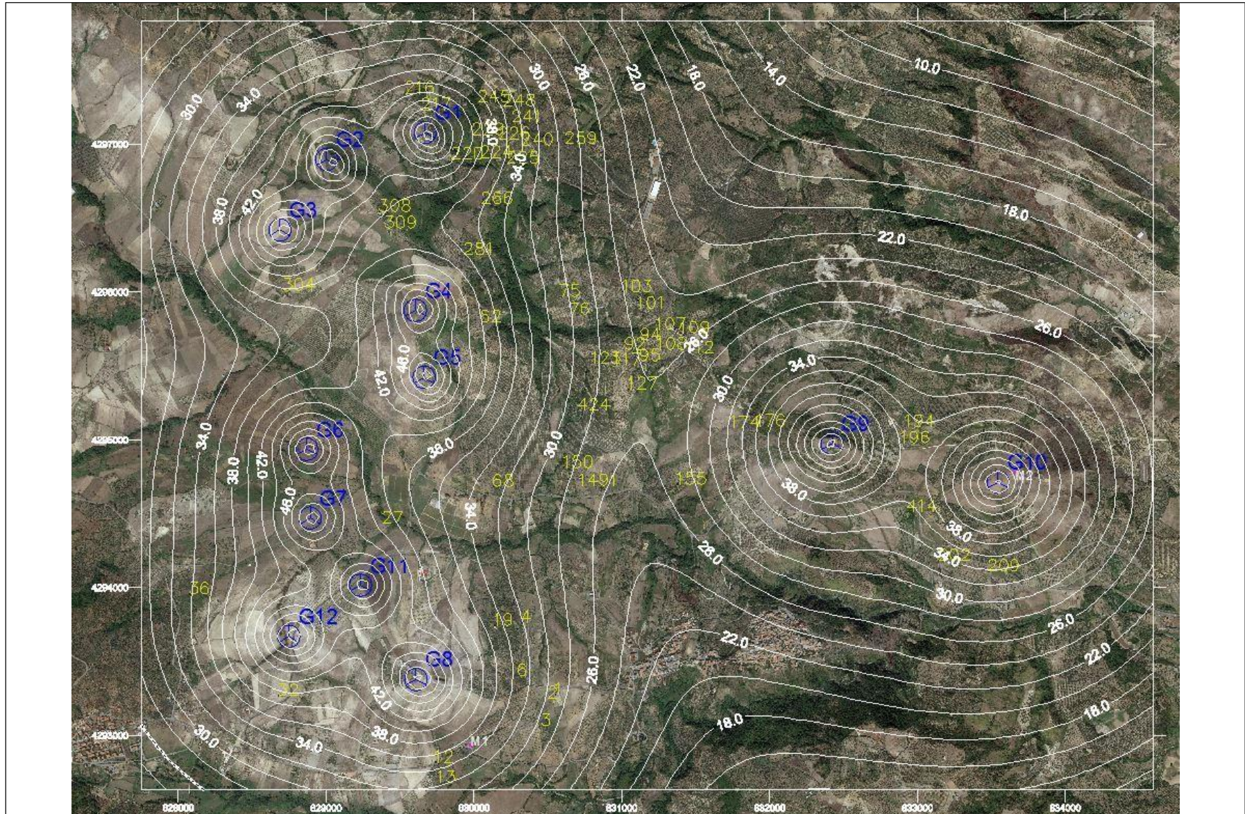
Fig. 5 – Isofoniche - Mappa a curve di livello della distribuzione del rumore indotto dagli aerogeneratori nell'area del Parco Eolico
