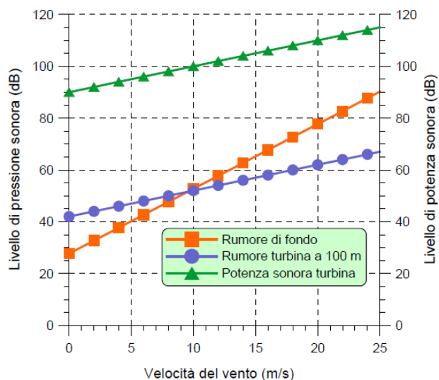
Fig. 3 – Livello rumore residuo in rapporto alla velocità del vento
