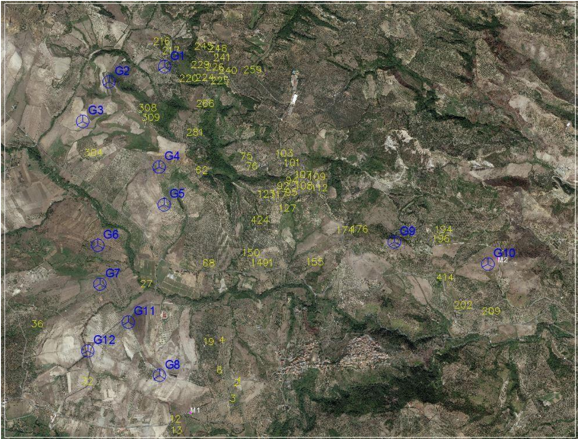
Fig. 1 – Layout del Parco Eolico "Bolina"
