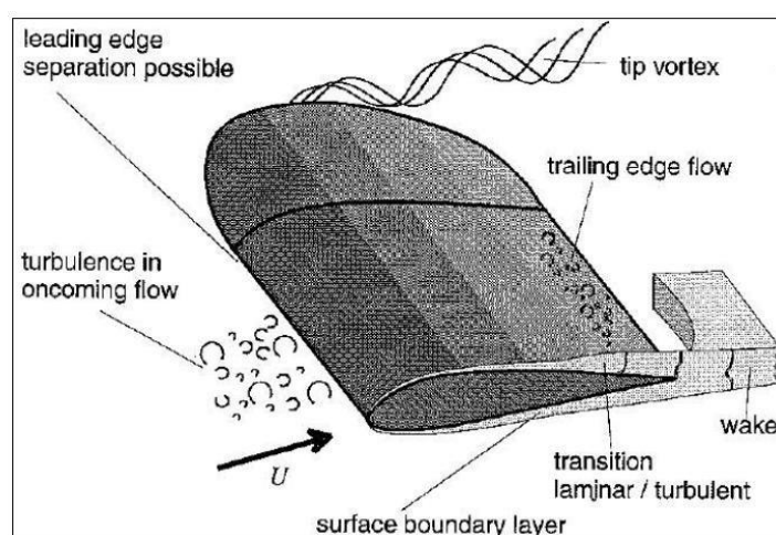
Fig. 2 – Flusso dell'aria sul profilo della pala
