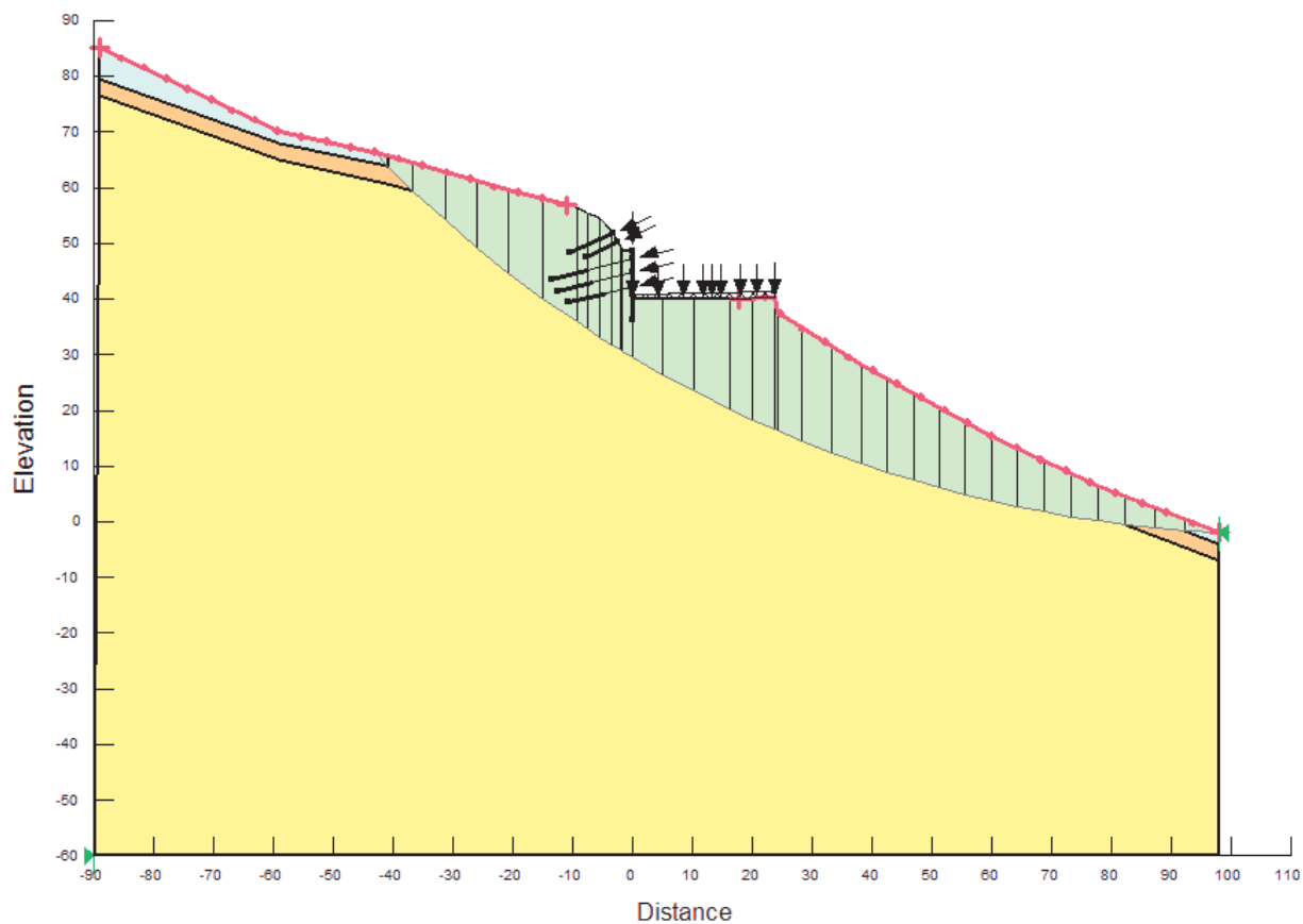
Figura 16 Coefficiente di sicurezza minimo per la stabilit  globale in condizioni sismiche (EQK+M2) (-)
