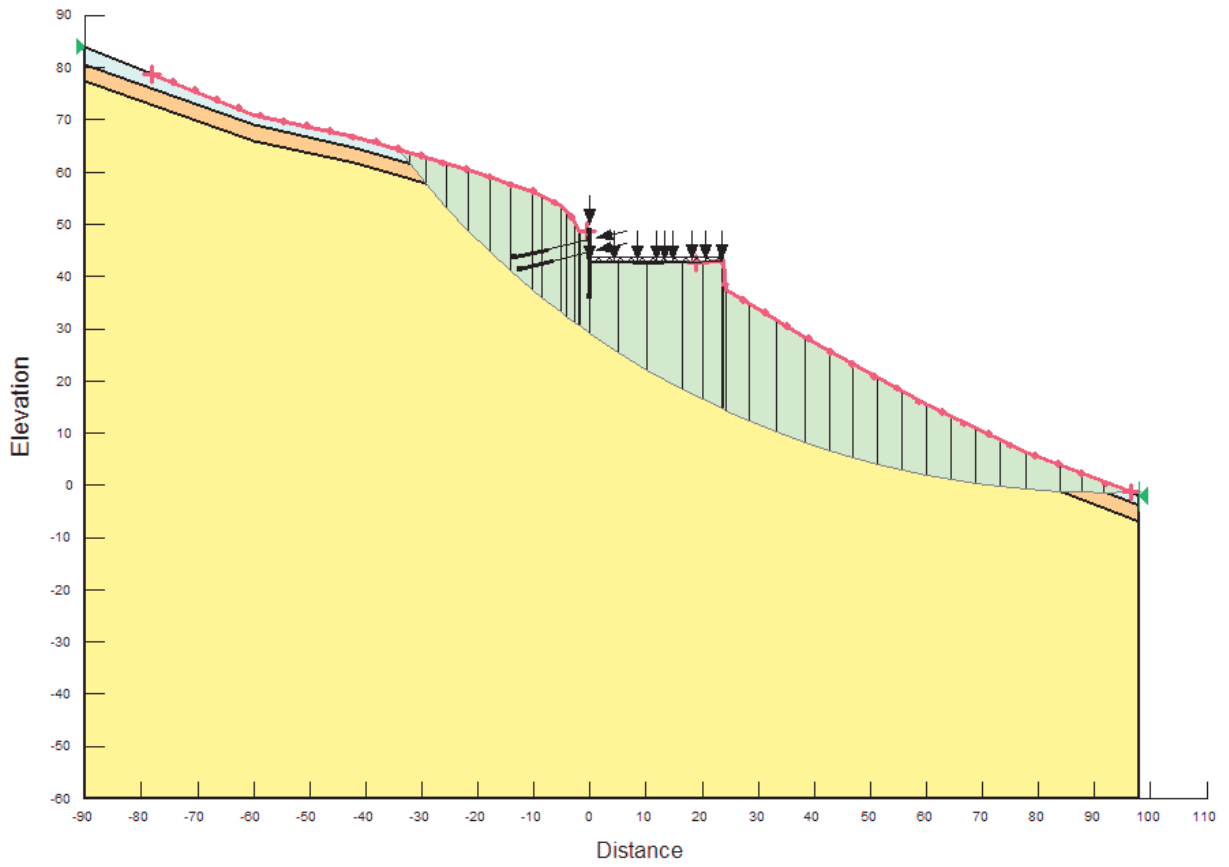
Figura 13 Coefficiente di sicurezza minimo per la stabilità globale in condizioni sismiche (EQK+M2) (-)
