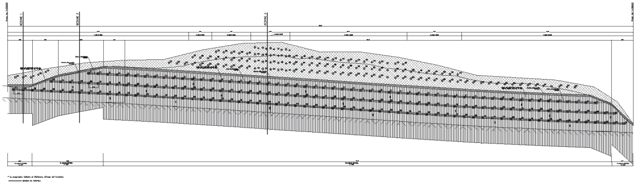
Figura 1 Sviluppata della paratia OM08
