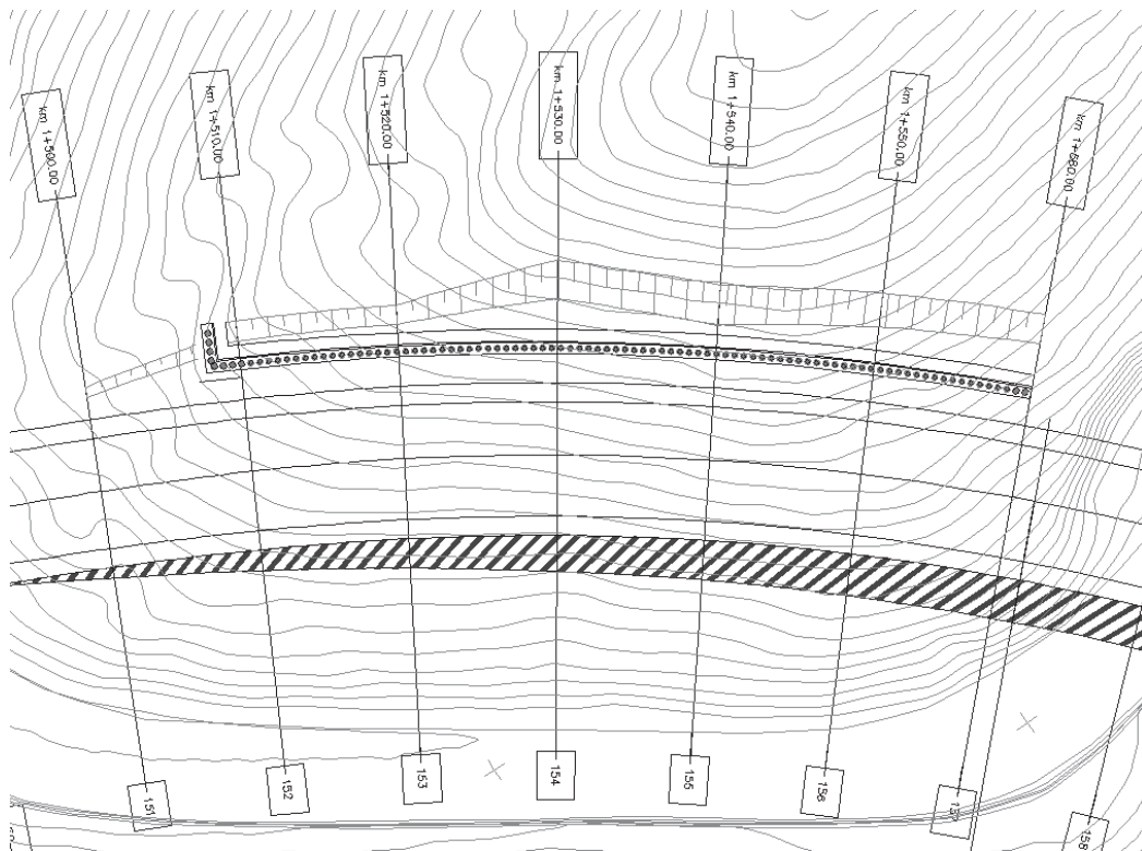
Figura 2 Planimetria d'intervento della paratia OM03
