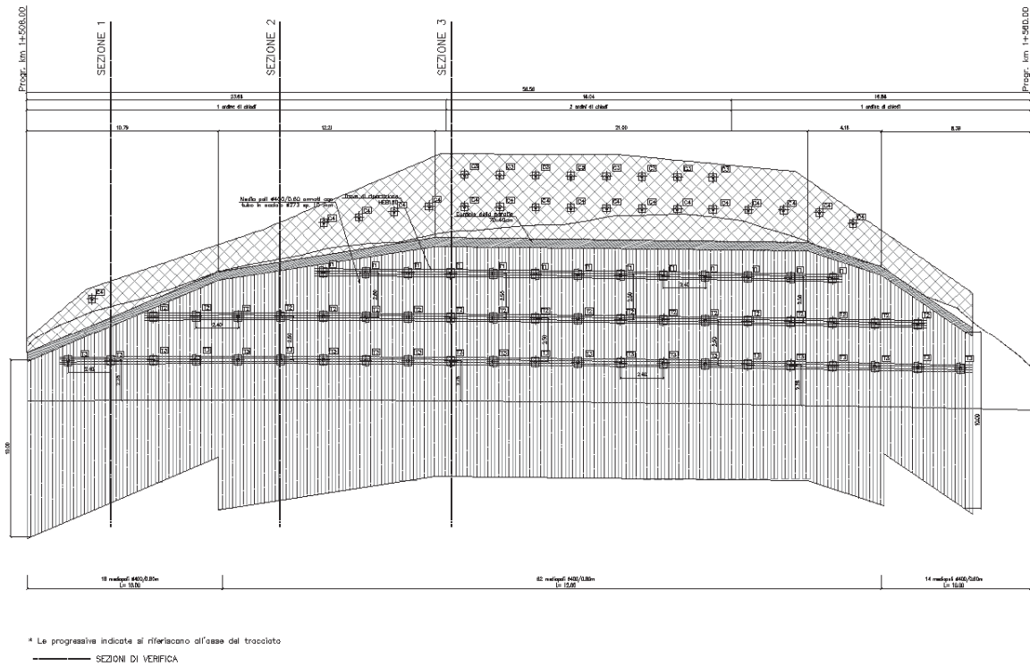
Figura 1 Sviluppata della paratia OM09
