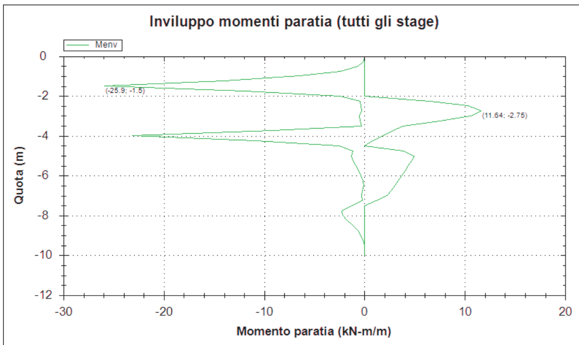
Figura 21: Diagramma dei momenti flettenti (A1+M1+R1)
