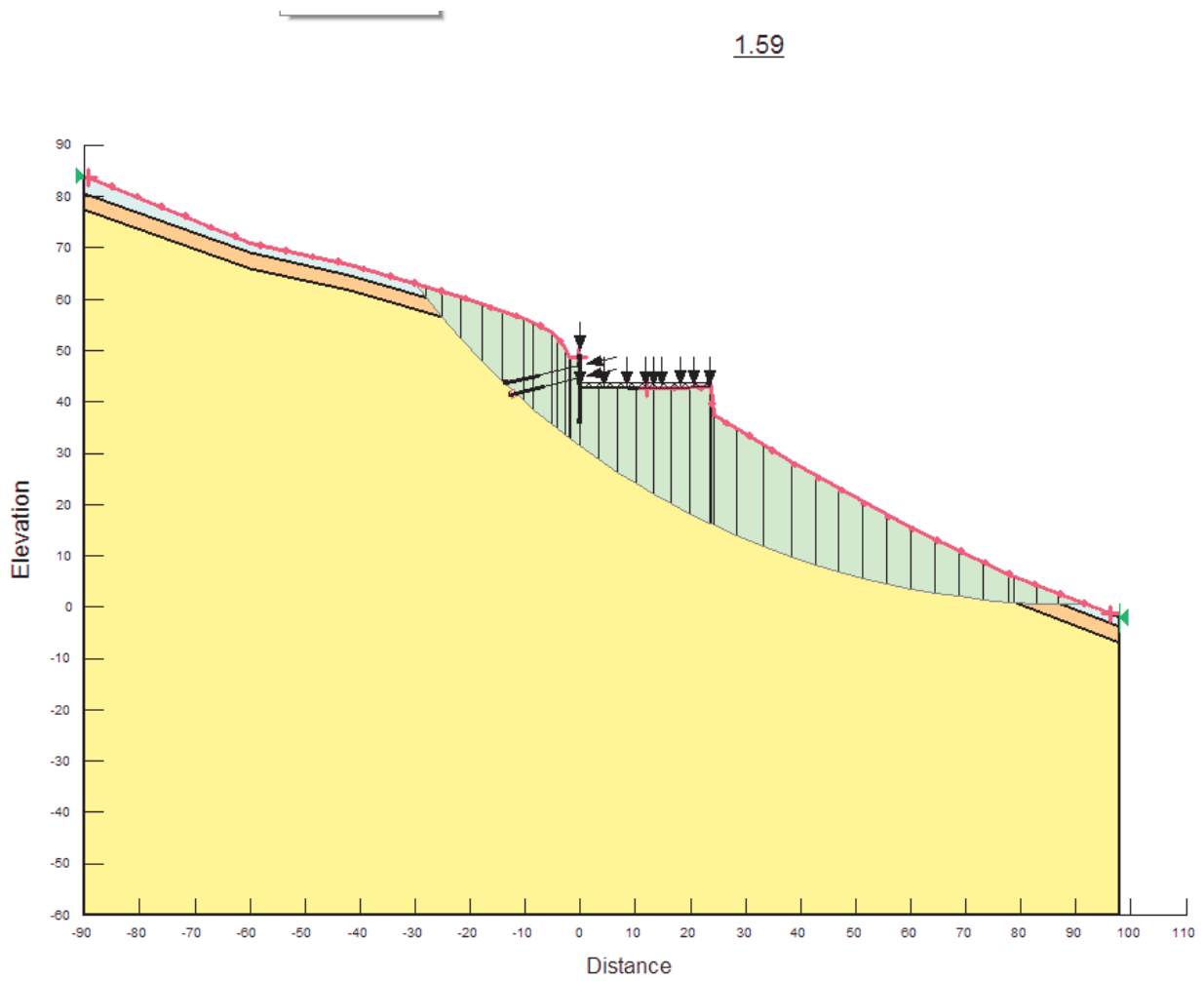
Figura 11 Coefficiente di sicurezza minimo per la stabilità globale in condizioni statiche (A2+M2)
