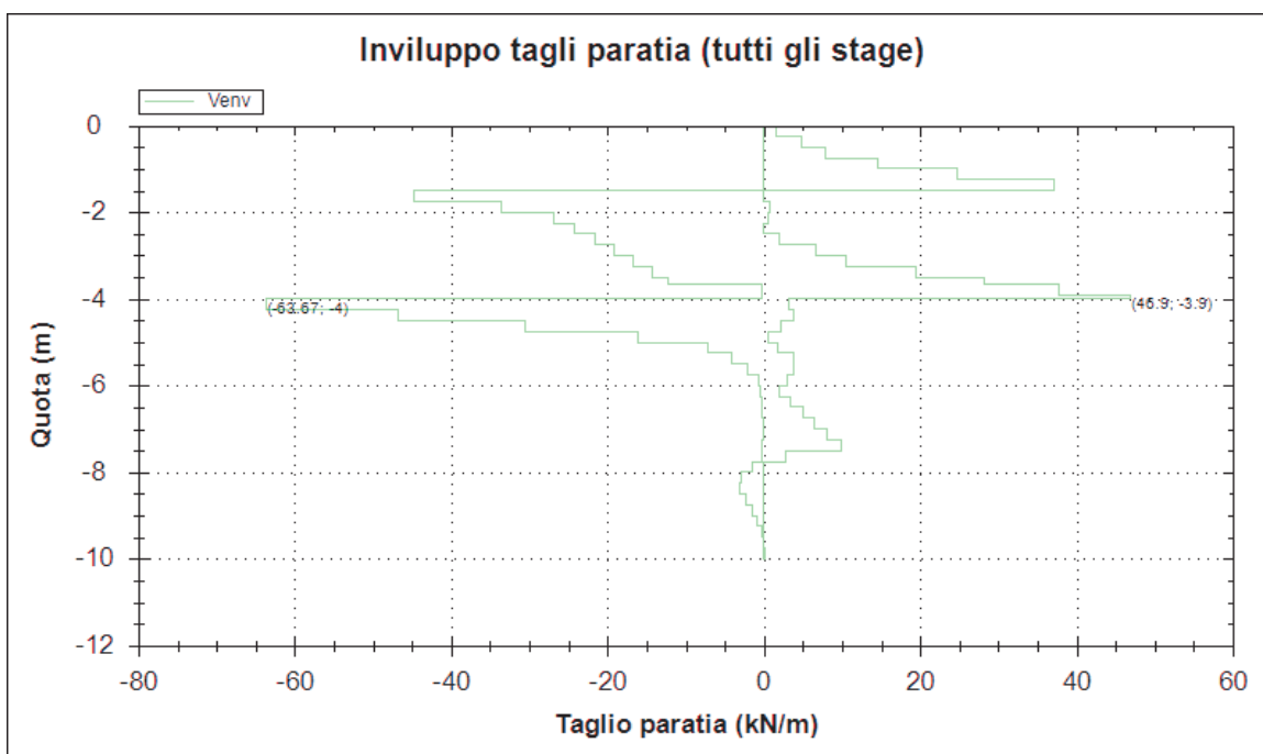
Figura 24: Diagramma del taglio (EQK+M1+R1)
