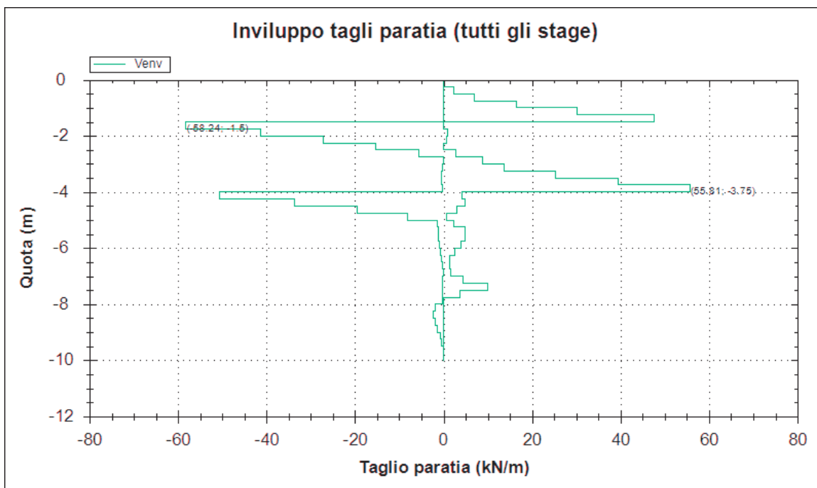
Figura 23: Diagramma del taglio (A1+M1+R1)
