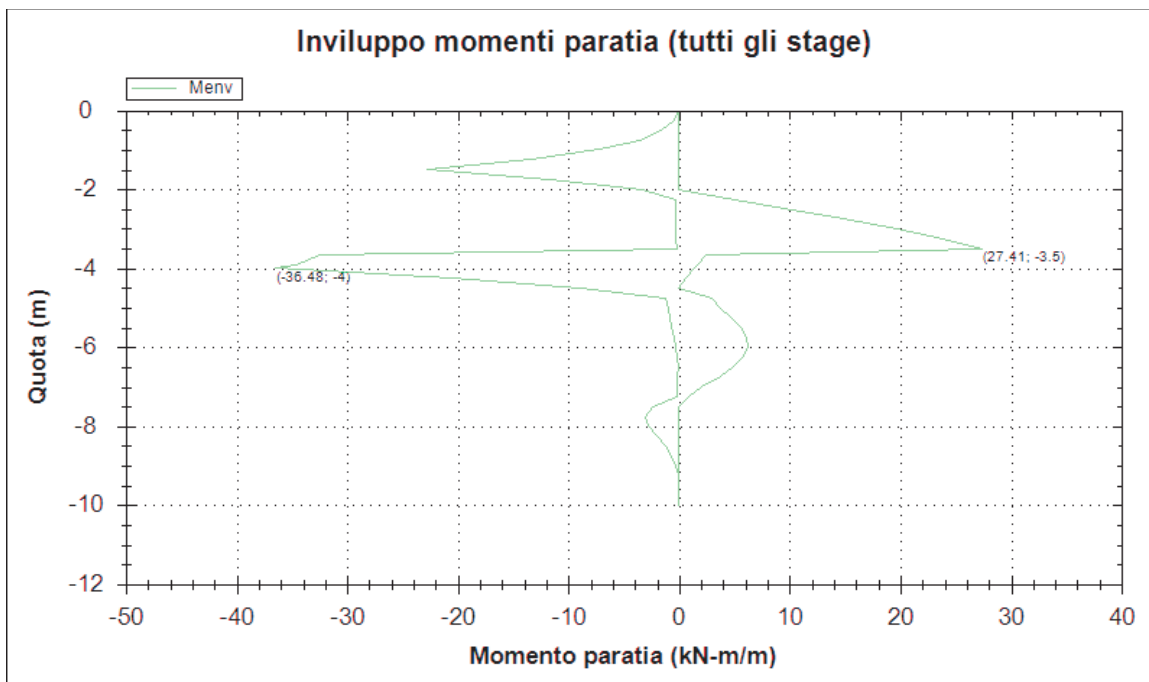
Figura 22: Diagramma dei momenti flettenti (EQK+M1+R1)
