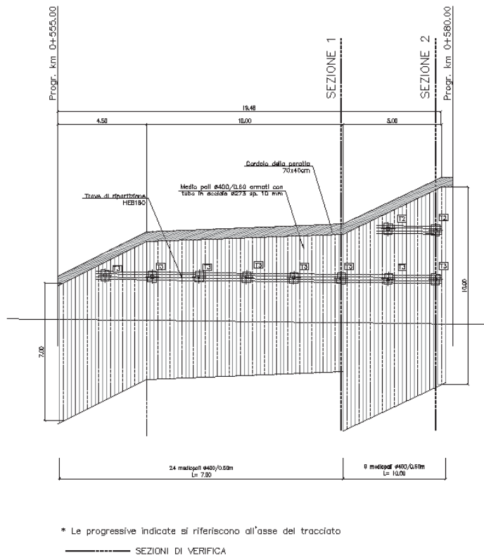
Figura 1 Sviluppata della paratia OM11
