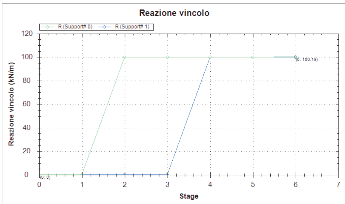
Figura 26: Reazioni tiranti (EQK+M1+R1)
