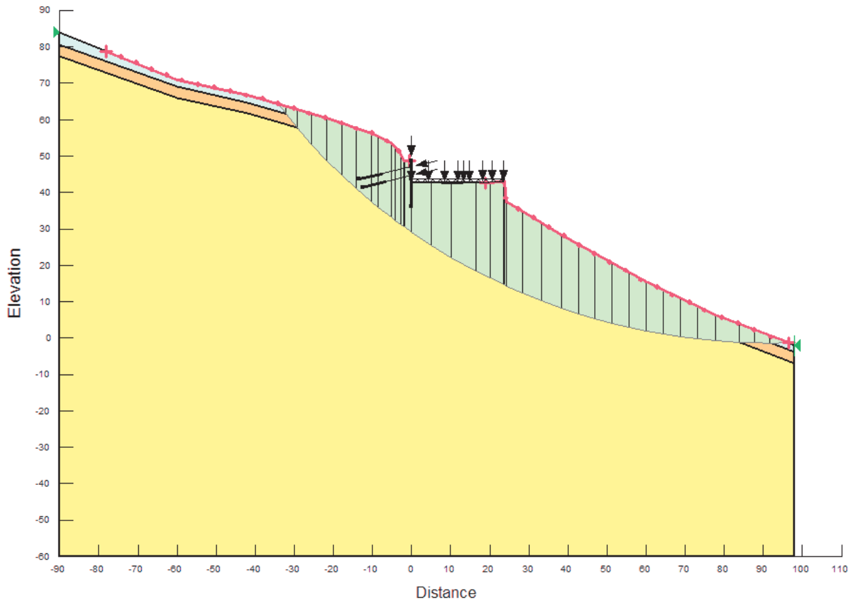
Figura 12 Coefficiente di sicurezza minimo per la stabilità globale in condizioni sismiche (EQK+M2) (+)
