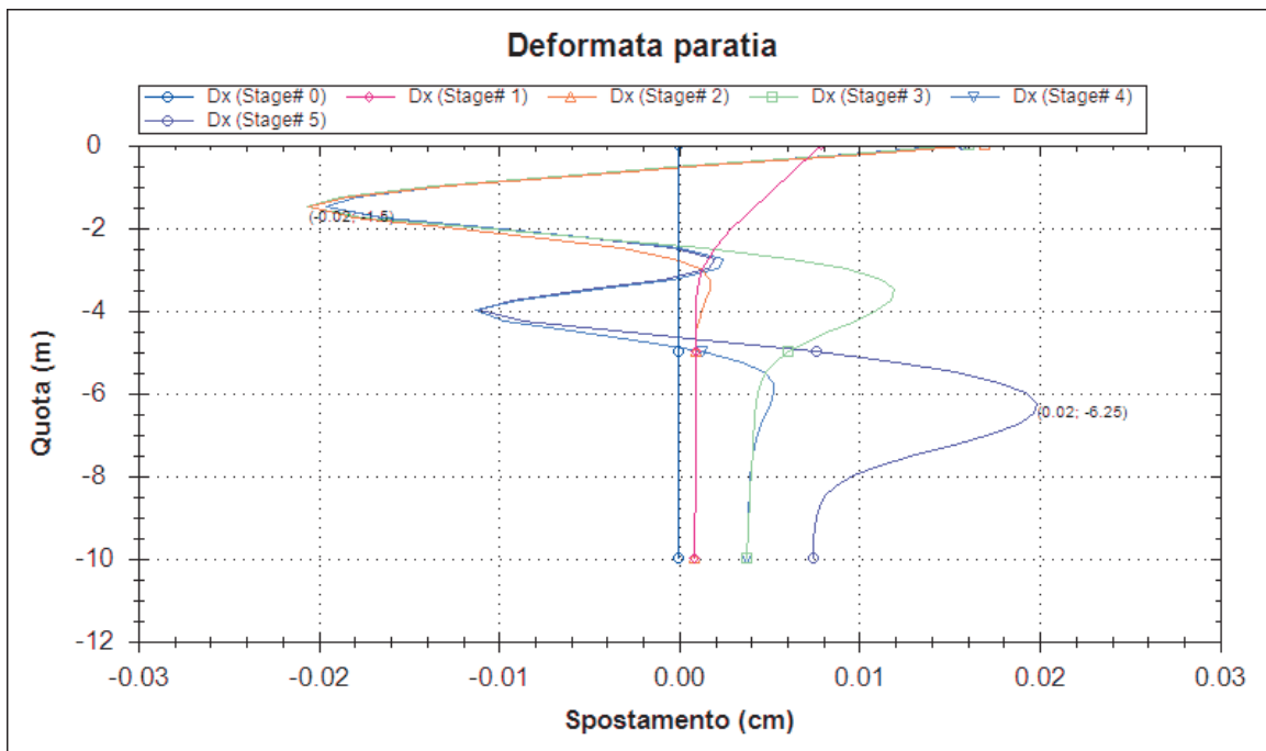
Figura 27: Diagramma degli spostamenti orizzontali (SLE)
