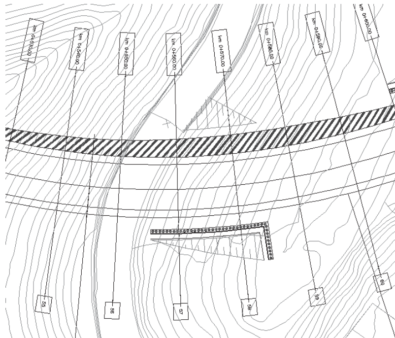
Figura 2 Planimetria d'intervento della paratia OM11
