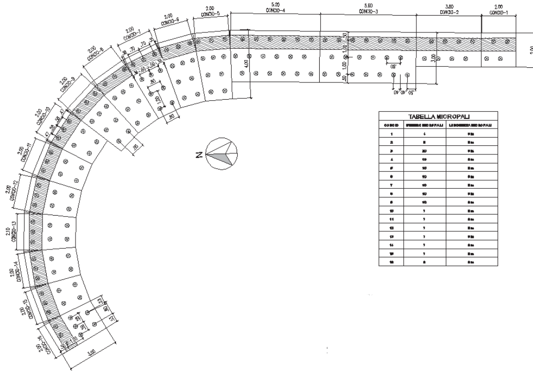
Figura 3: pianta del muro
