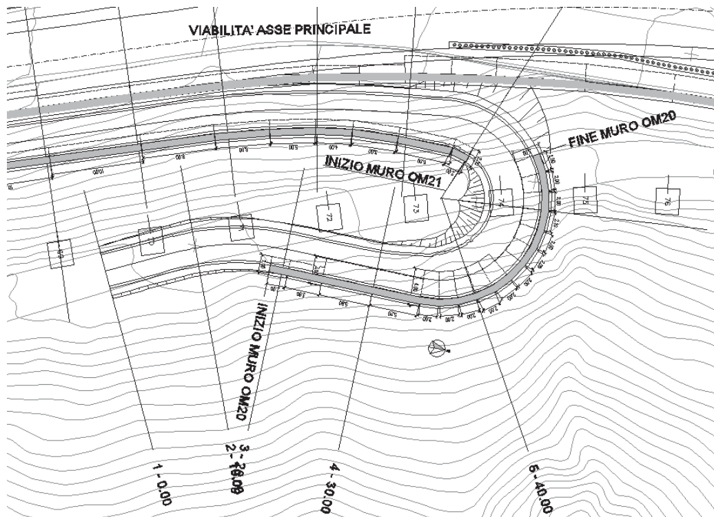
Figura 4: planimetria del muro
