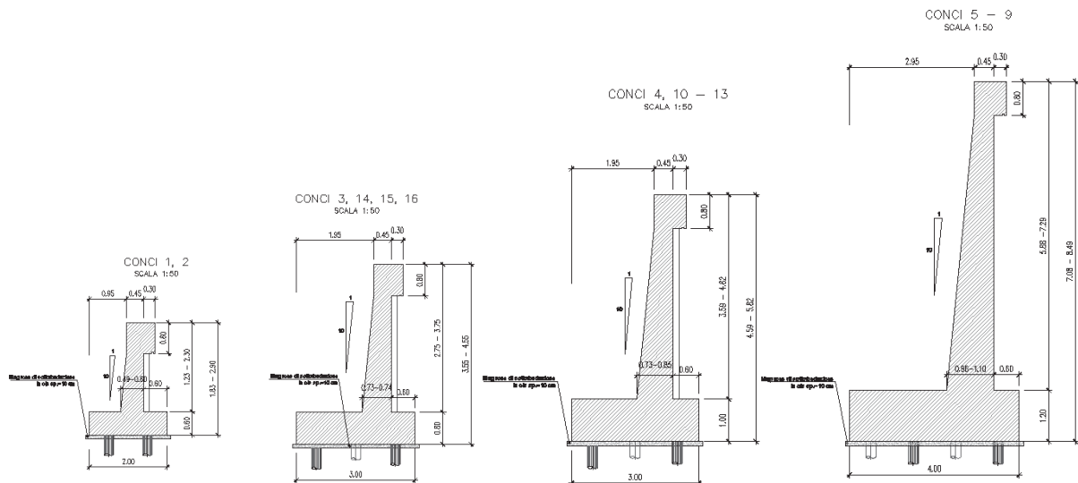
Figura 2: carpenteria del muro
