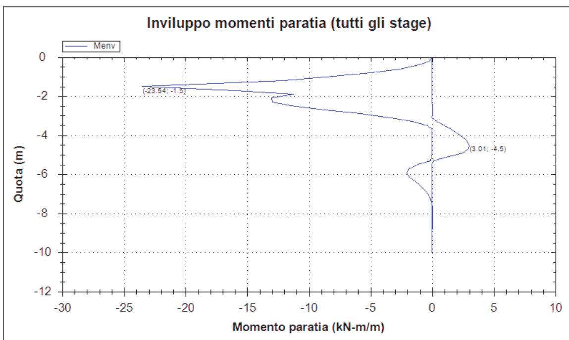
Figura 14: Diagramma dei momenti flettenti (EQK+M1+R1)
