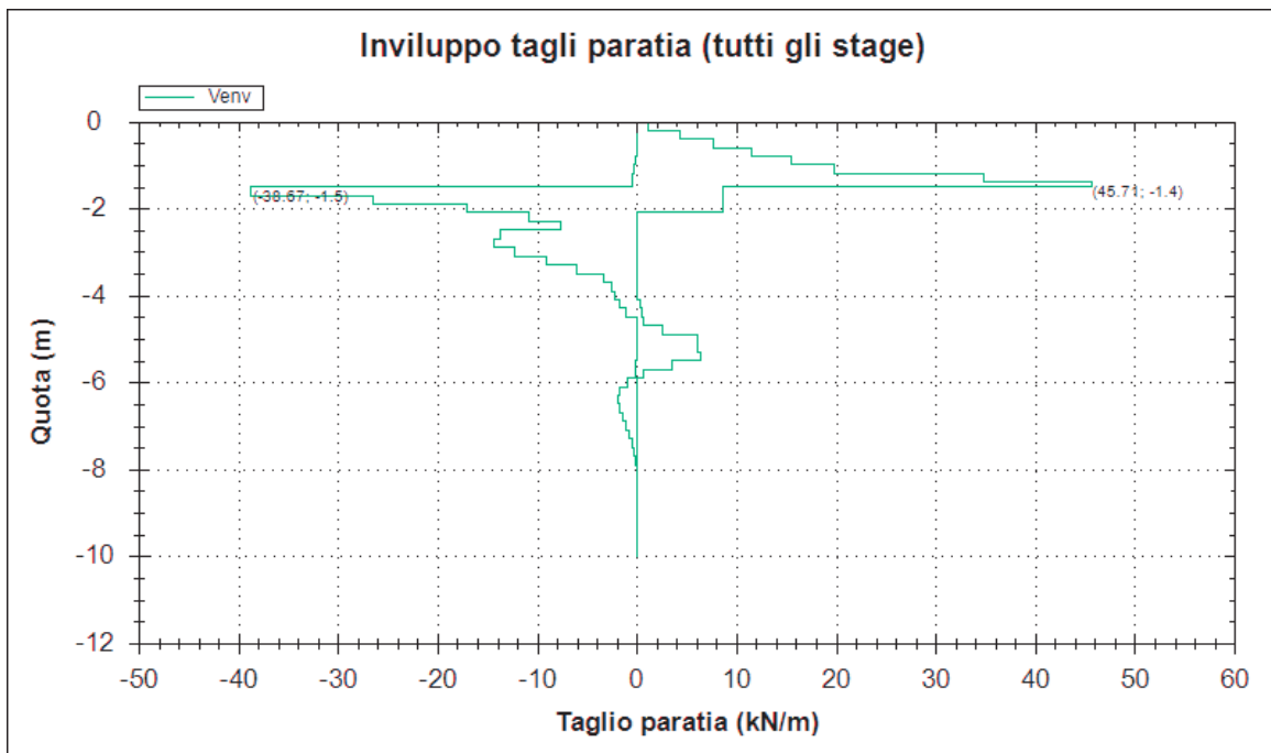
Figura 16: Diagramma del taglio (EQK+M1+R1)
