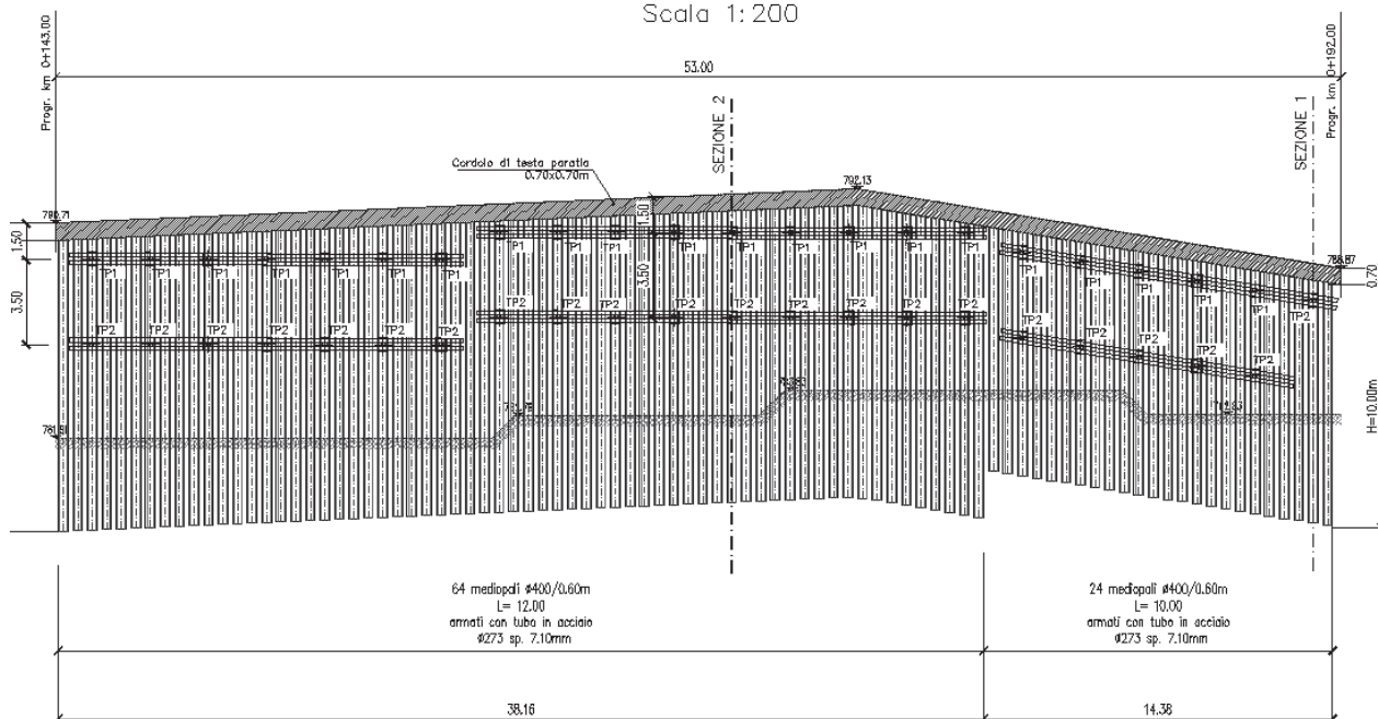
Figura 3: sviluppata paratia provvisoriale
