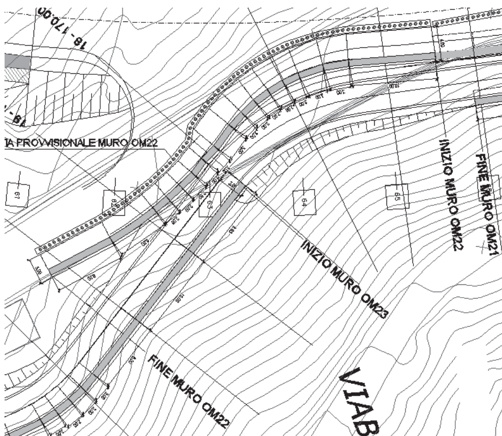
Figura 4 Planimetria d'intervento
