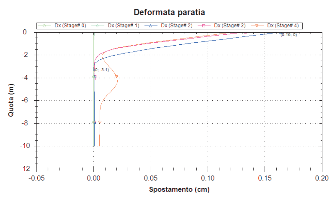
Figura 19: Diagramma degli spostamenti orizzontali (SLE)
