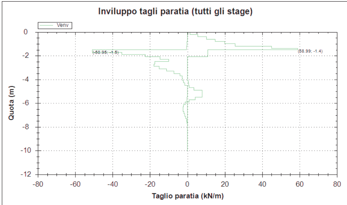
Figura 15: Diagramma del taglio (A1+M1+R1)
