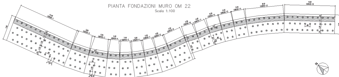
Figura 2: carpenteria del muro
