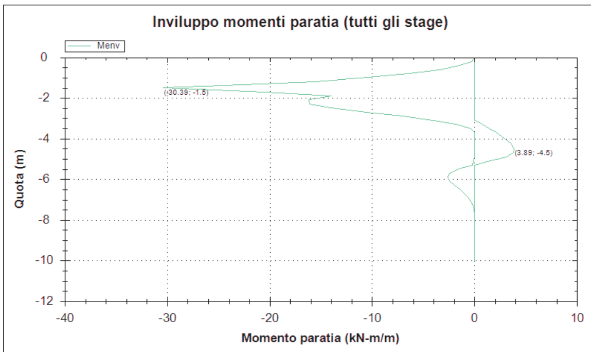
Figura 13: Diagramma dei momenti flettenti (A1+M1+R1)
