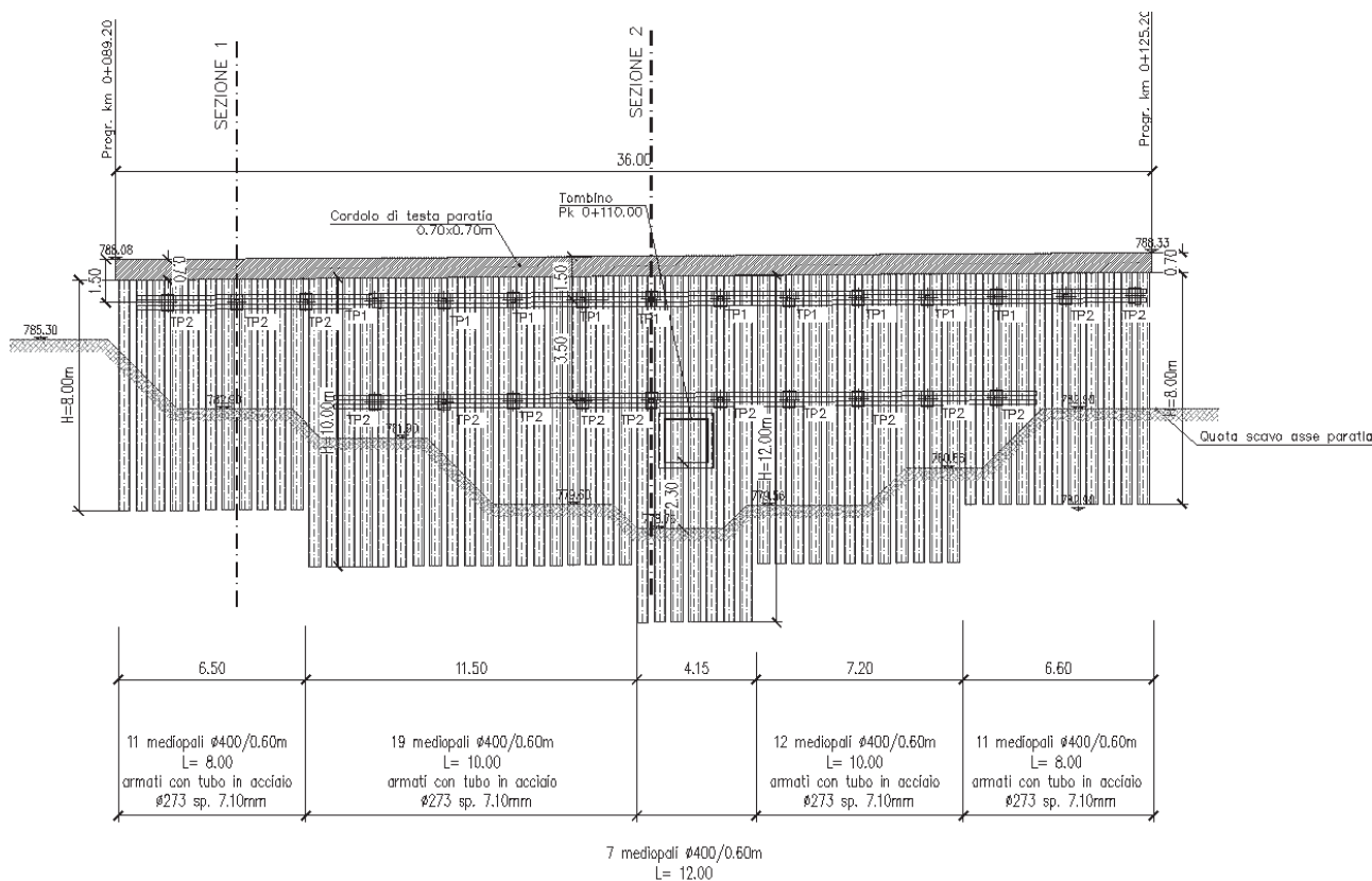
Figura 3: sviluppata paratia provvisoria
