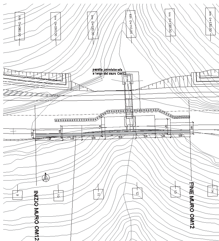
Figura 4 Planimetria d'intervento
