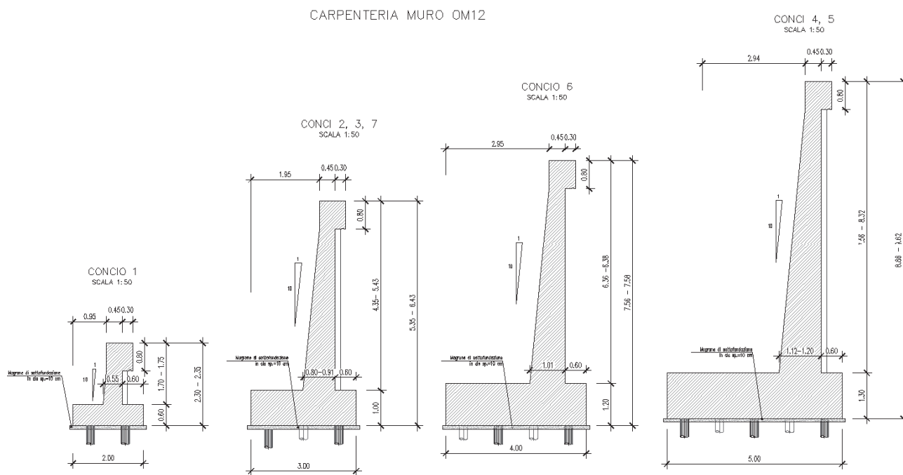
Figura 2: carpenteria del muro
