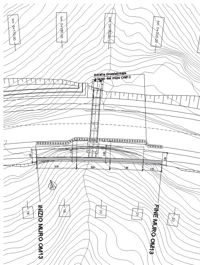
Figura 4 Planimetria d'intervento
