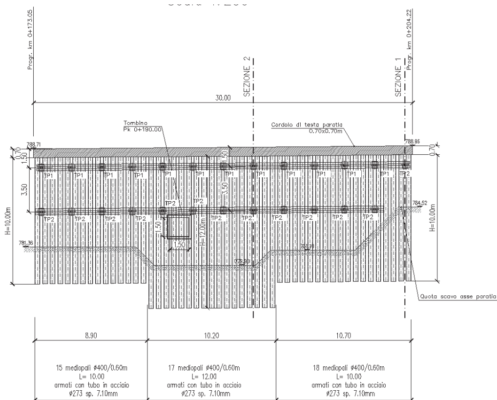
Figura 3: sviluppata paratia provvisoria
