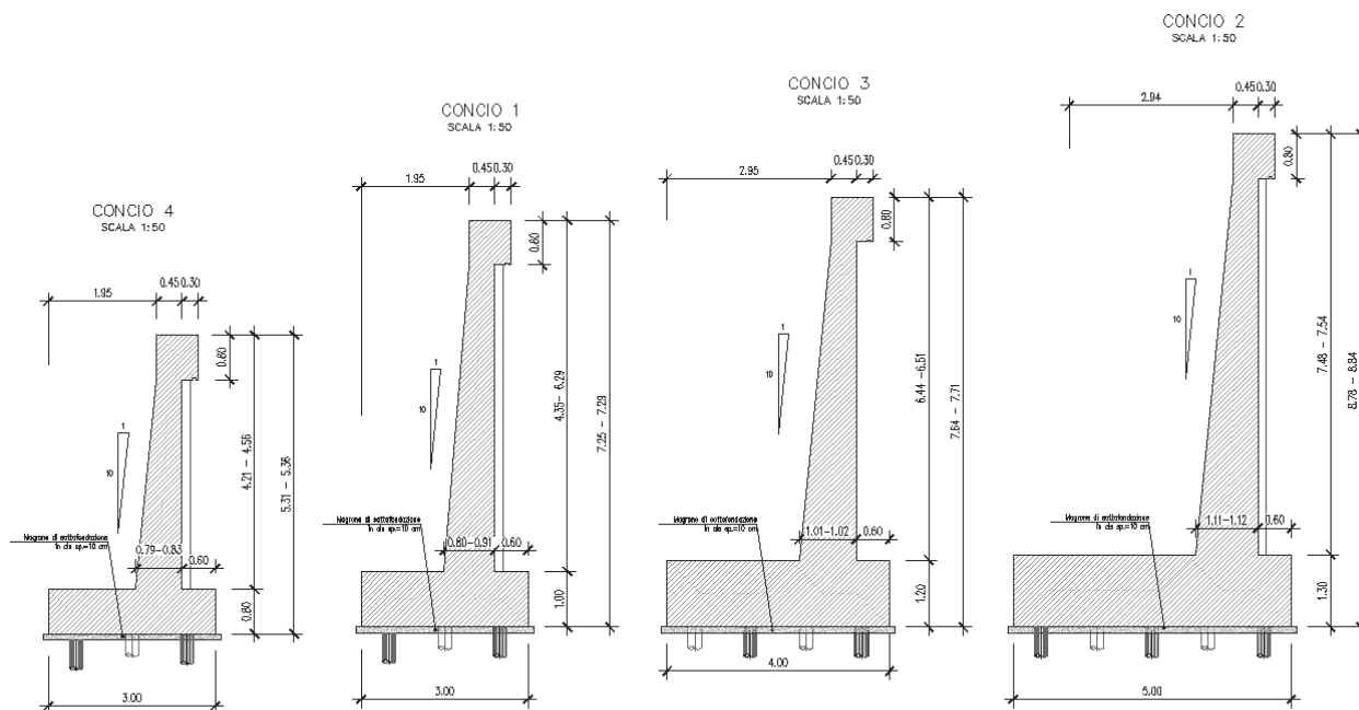
Figura 2: carpenteria del muro
