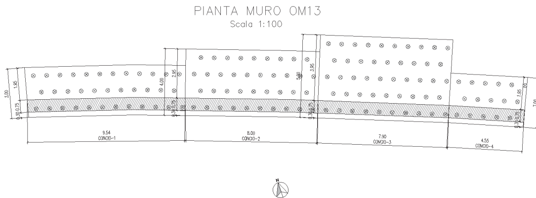
Figura 3: pianta del muro
