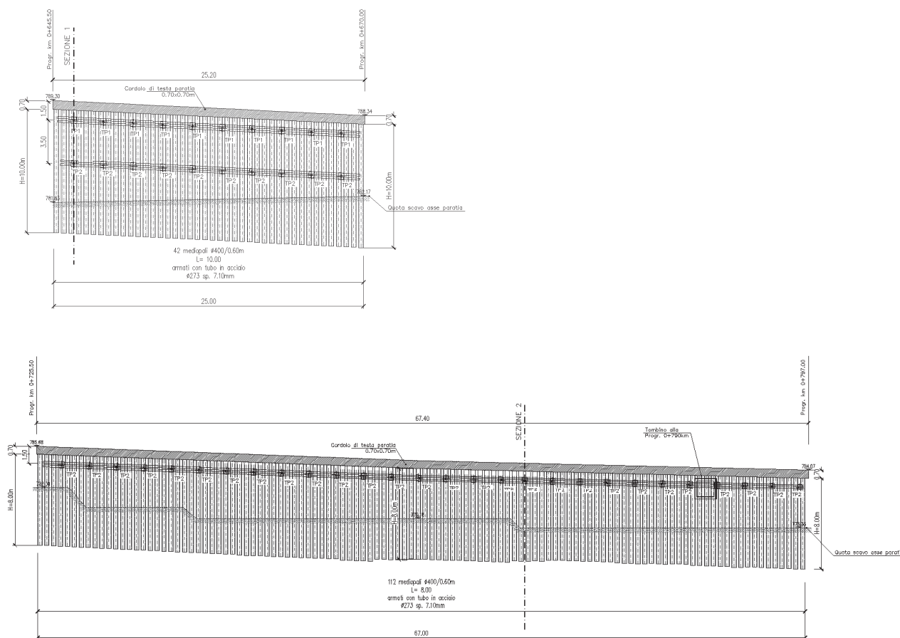
Figura 3: sviluppata paratia provvisoria
