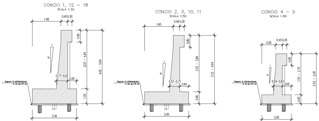
Figura 2: carpenteria del muro
