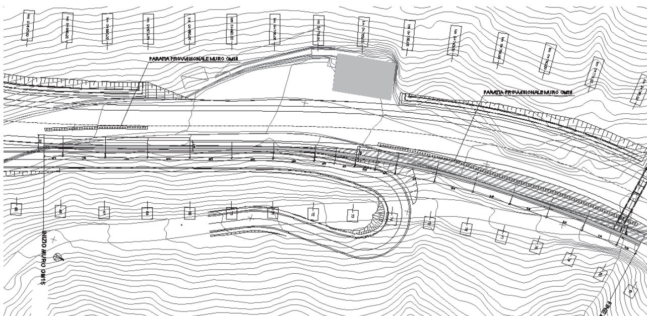
Figura 4 Planimetria d'intervento
