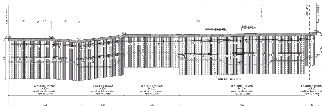
Figura 3: sviluppata paratia provvisoria
