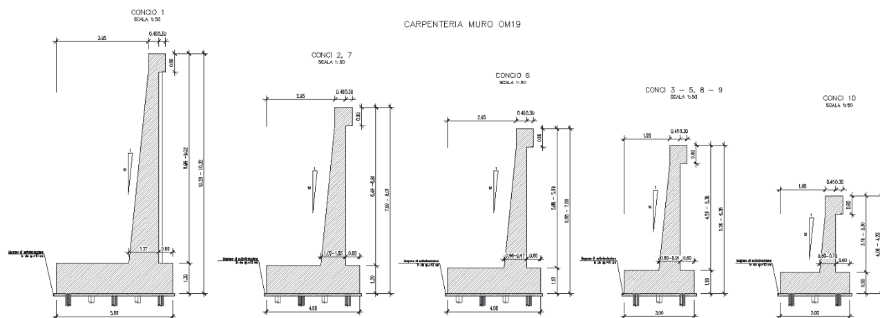
Figura 2: carpenteria del muro
