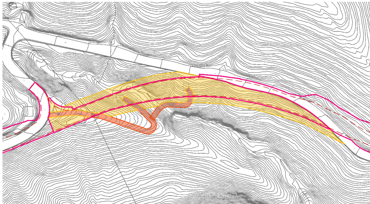
In giallo è rappresentato il perimetro dell'area di cantiere operativo. Estratto Planimetria aree do cantiere e viabilità di cantiere "T00CA00CANPL01A".
