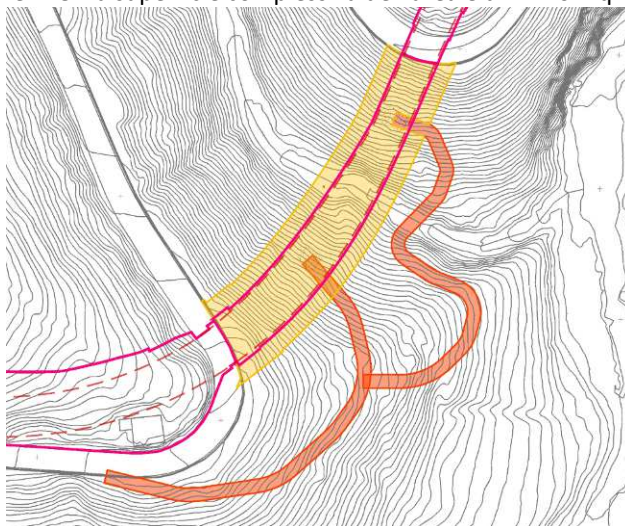
In giallo è rappresentato il perimetro dell'area di cantiere operativo. Estratto Planimetria aree da cantiere e viabilità di cantiere "TOOCAOOCANPLO1A".
