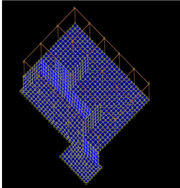
Figura 3 – deformazioni in condizioni SLO sisma Y
