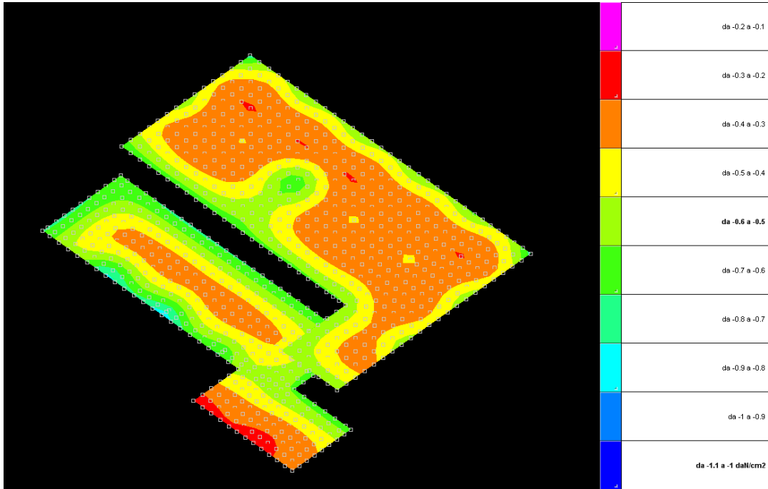
Figura 7 – pressioni sul terreno (massime)
