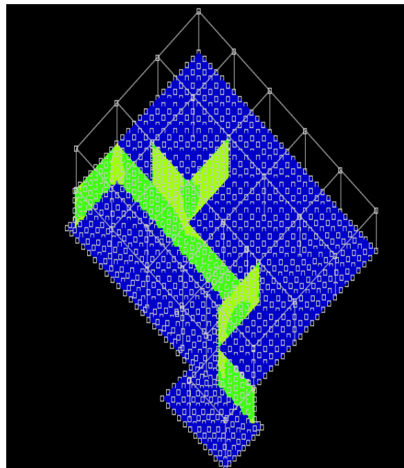
Figura 4 – sollecitazioni Moo massime
