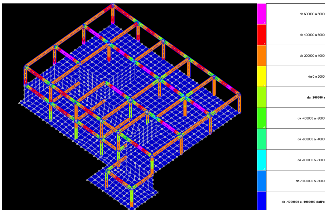
Figura 6 – sollecitazioni massime aste
