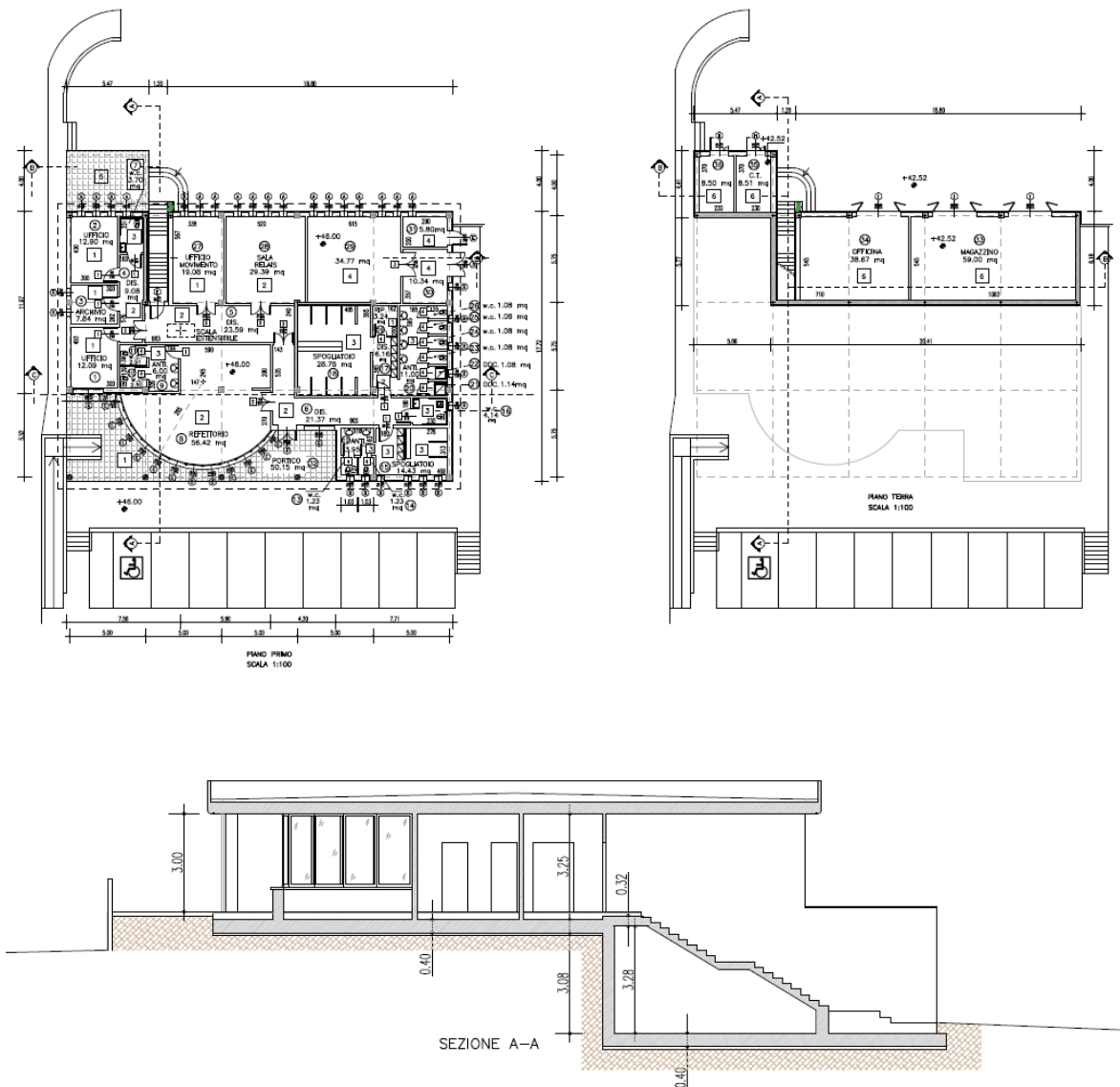
Figura 1 – piante e sezione dell'intervento
