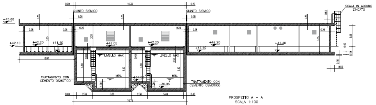
Figura 1 – pianta e sezioni dell'intervento
