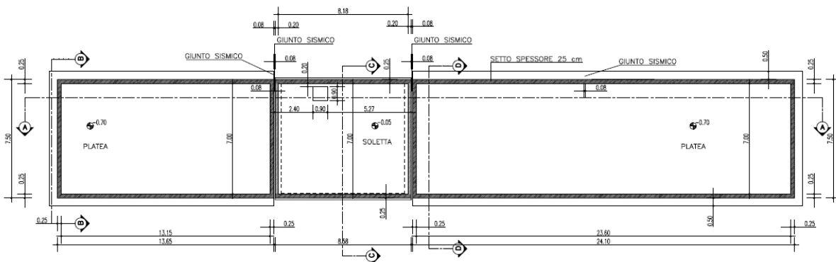
PIANTA PLATEA E SPICCATO PILASTRI SCALA 1:100
