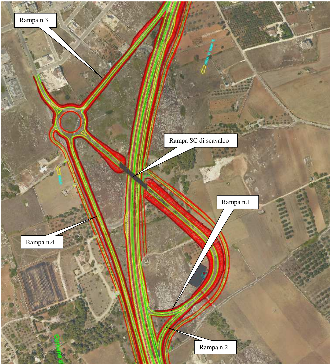
Figura 18: Svincolo 7 – SCORRANO SUD configurazione di progetto
