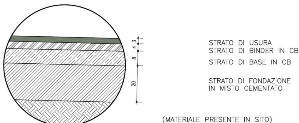
Fig. 10. Sezione pavimentazione rampe di svincolo
