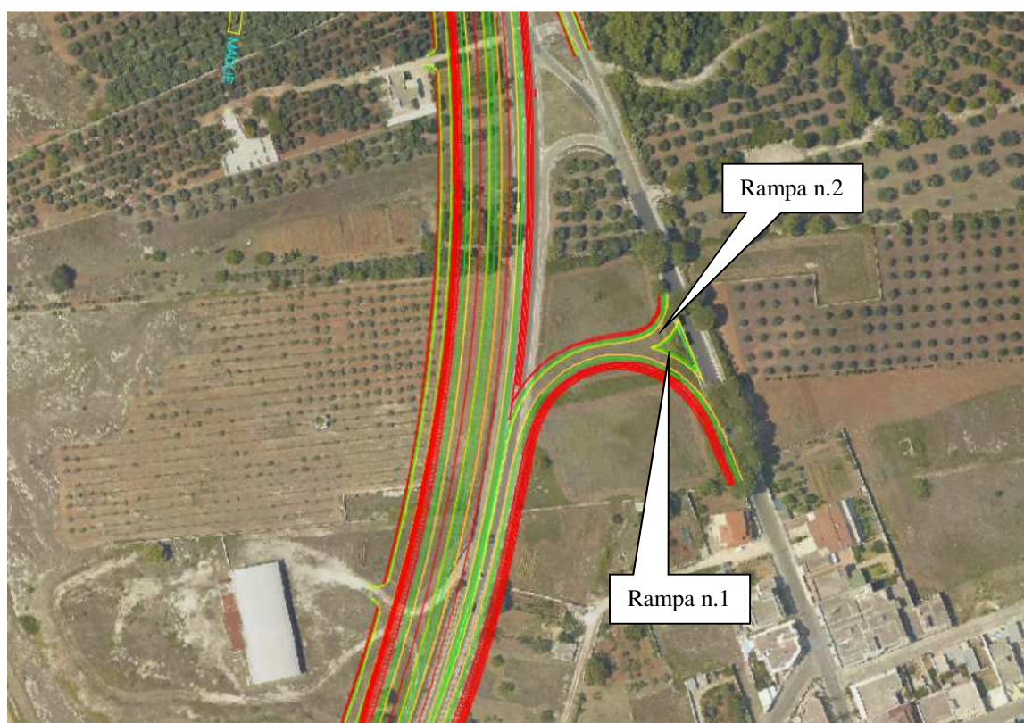
Figura 21: Svincolo 9b – NOCIGLIA NORD – configurazione di progetto
