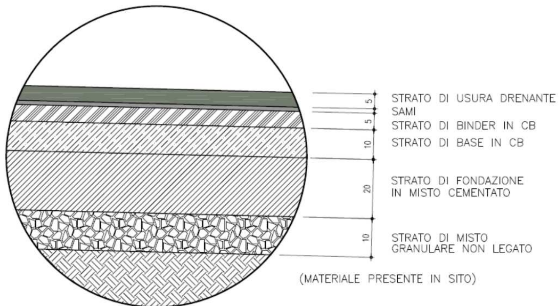
Figura 9. Sezione pavimentazione dell'asse principale e corsie dedicate
