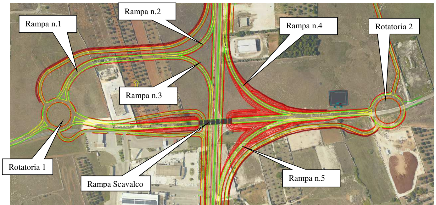
Figura 23: Svincolo 10 – SURANO – RUFFANO configurazione di progetto
