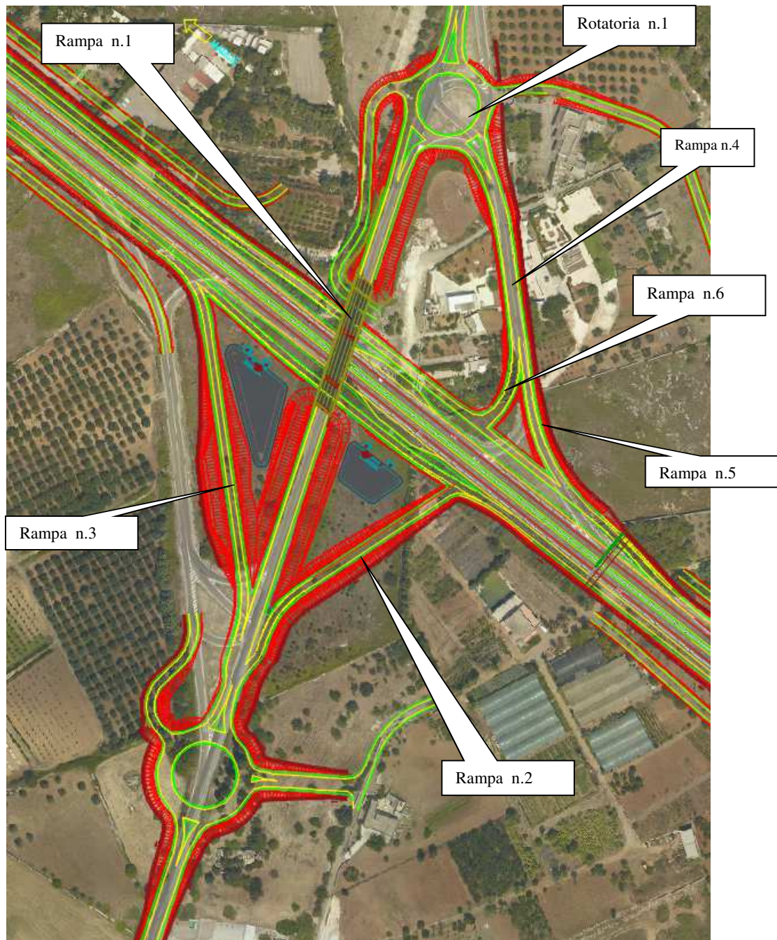
Figura 13: Svincolo 2 – CURSI – nuova configurazione di progetto
