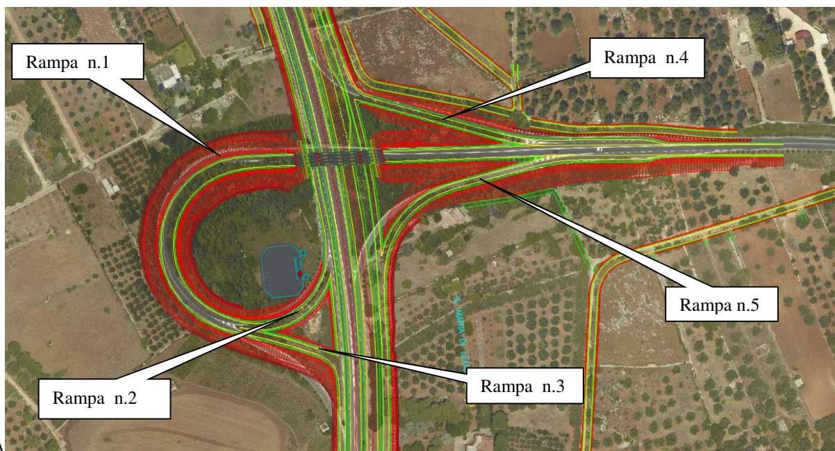
Figura 15: Svincolo 4 - SANTA CESAREA TERME – configurazione di progetto
