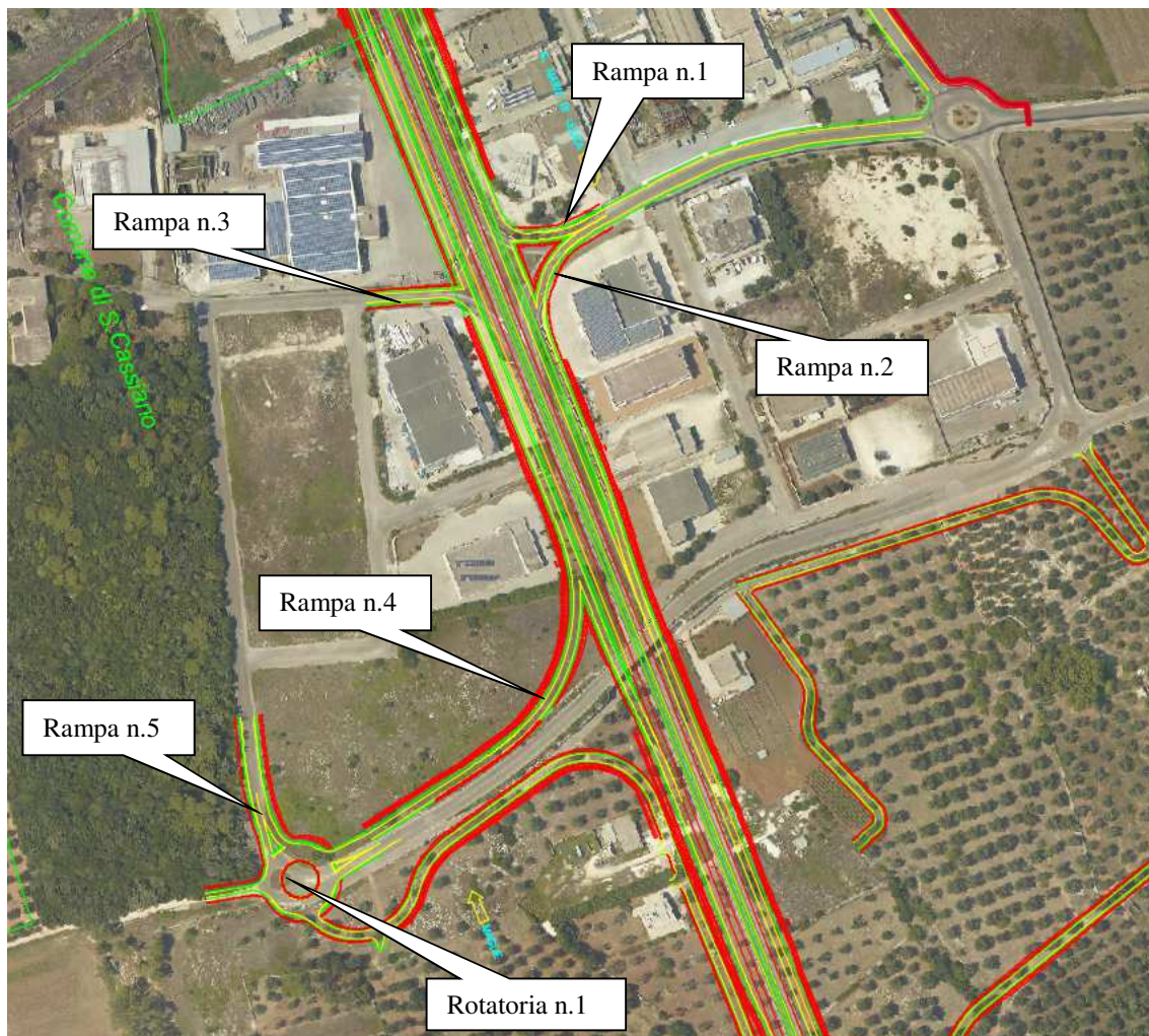
Figura 20: Svincolo 8 b – BOTRUGNO SUD – nuova configurazione di progetto
