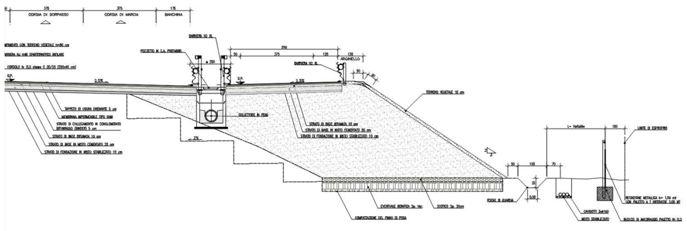
Fig. 8. Sezione Corsia Dedicata
