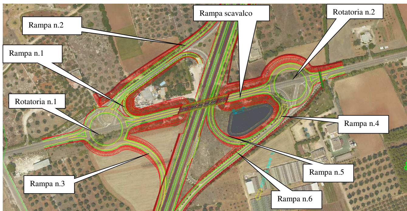
Figura 17: Svincolo 6 - SCORRANO NORD - configurazione di progetto
