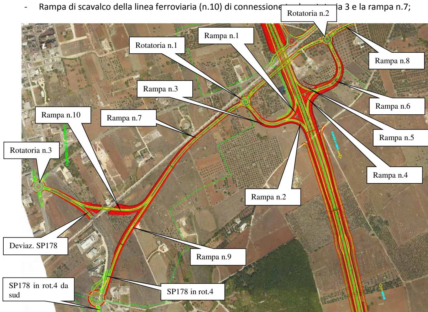
Figura 25: Svincolo 12 – Montesano – Andrano configurazione di progetto
