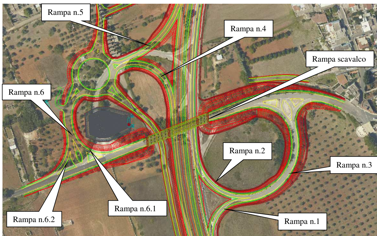
Figura 22: Svincolo 9 – NOCIGLIA – configurazione di progetto
