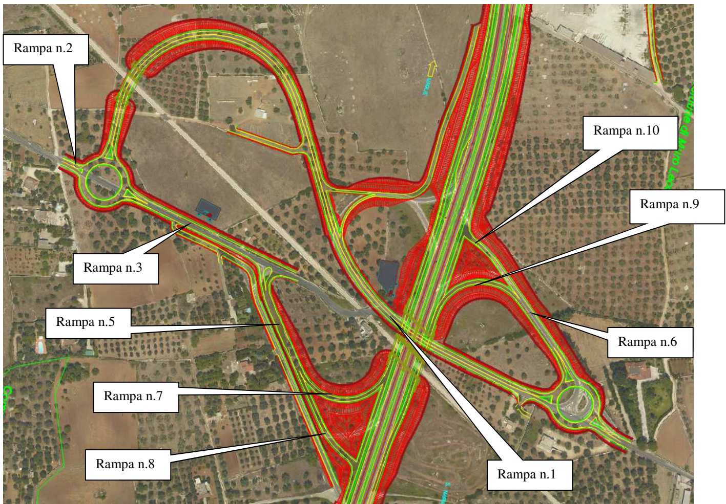
Figura 16: Svincolo 5 – MURO LECCESE – configurazione di progetto
