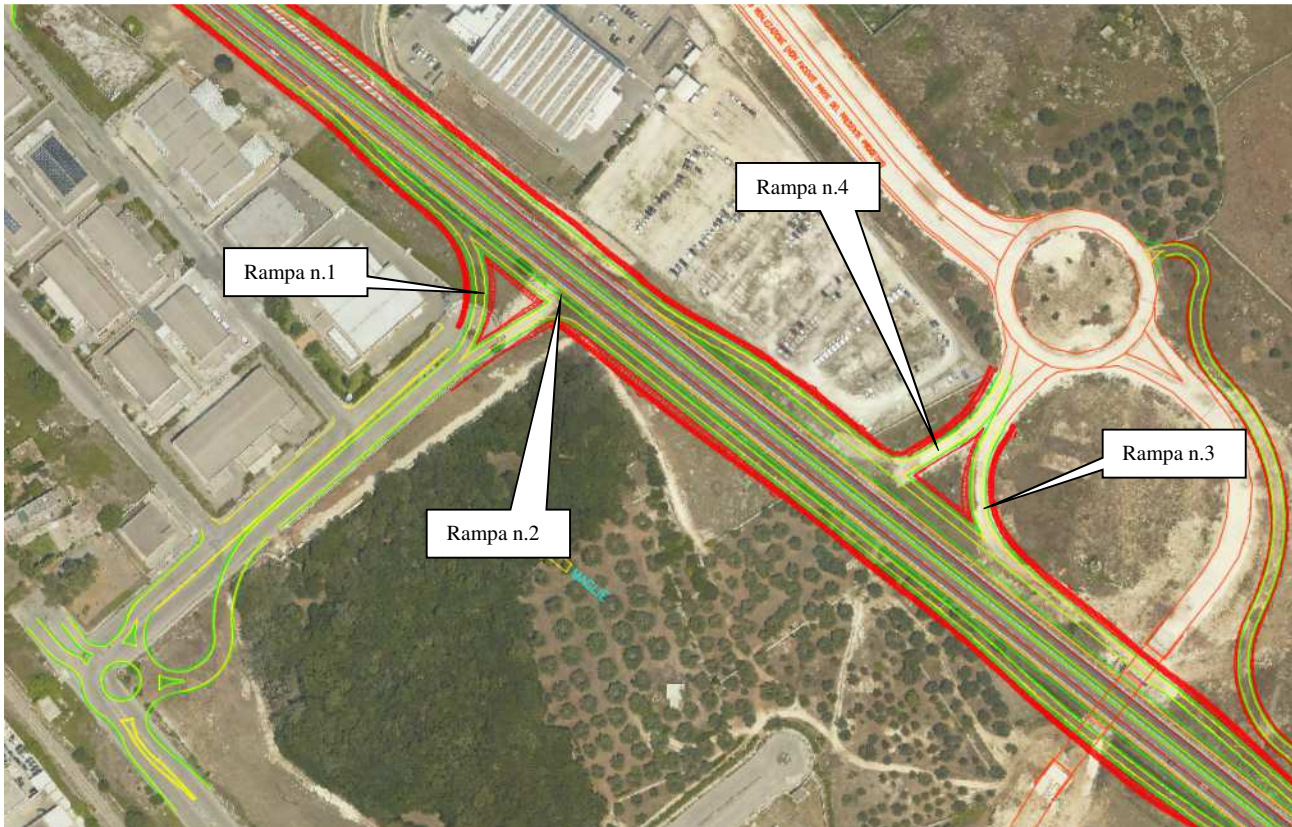
Figura 12: Svincolo 1 bis - Z.I. Maglie – nuova configurazione di progetto
