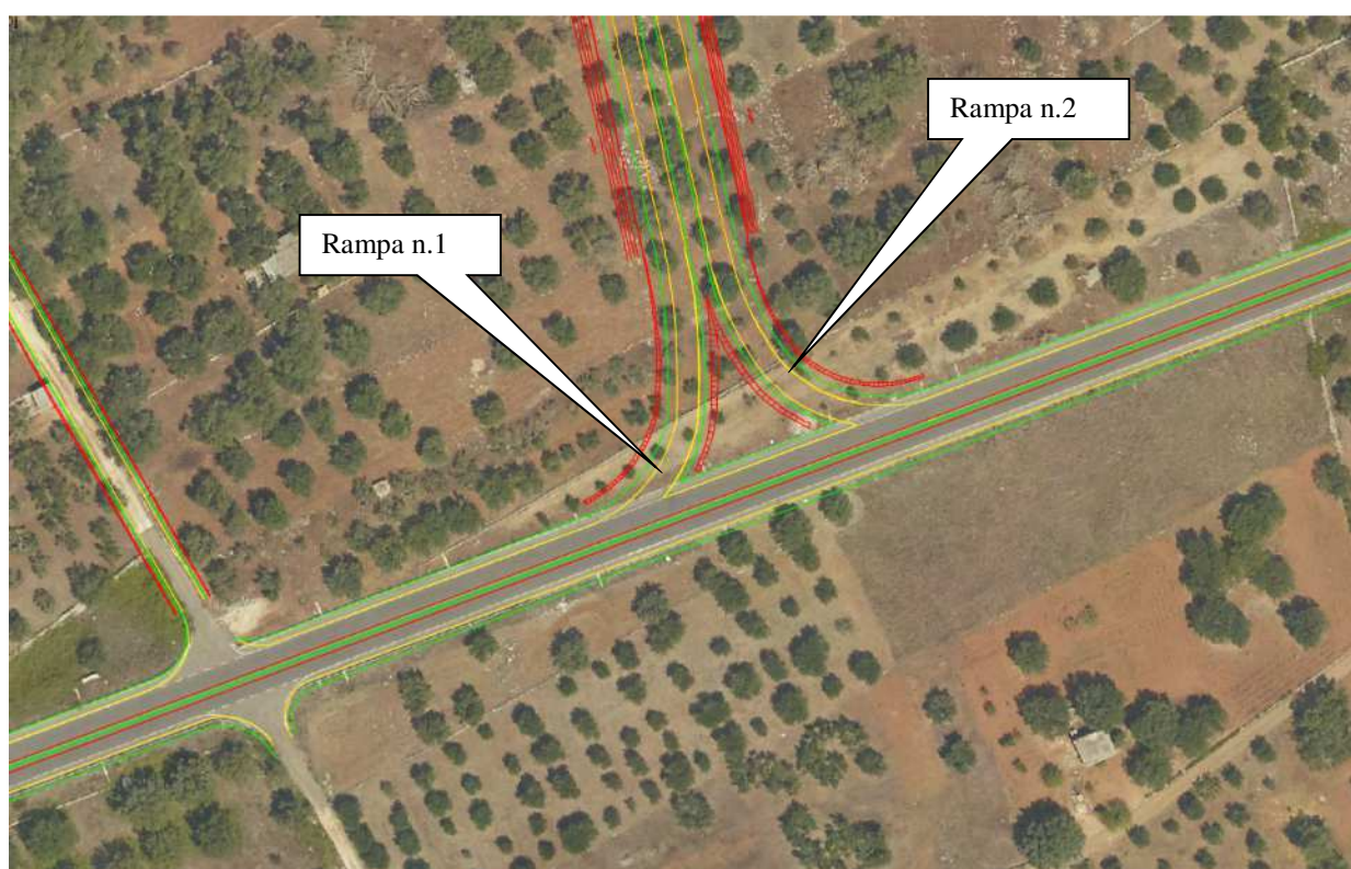
Figura 26: Fine Lotto - Zona Artigianale di Tricase configurazione di progetto
