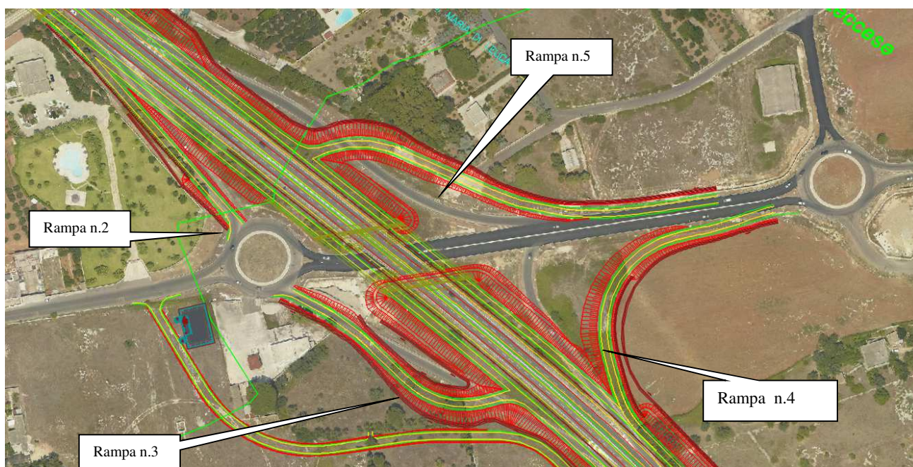
Figura 14: Svincolo 3 – Otranto SS 16 - configurazione di progetto
