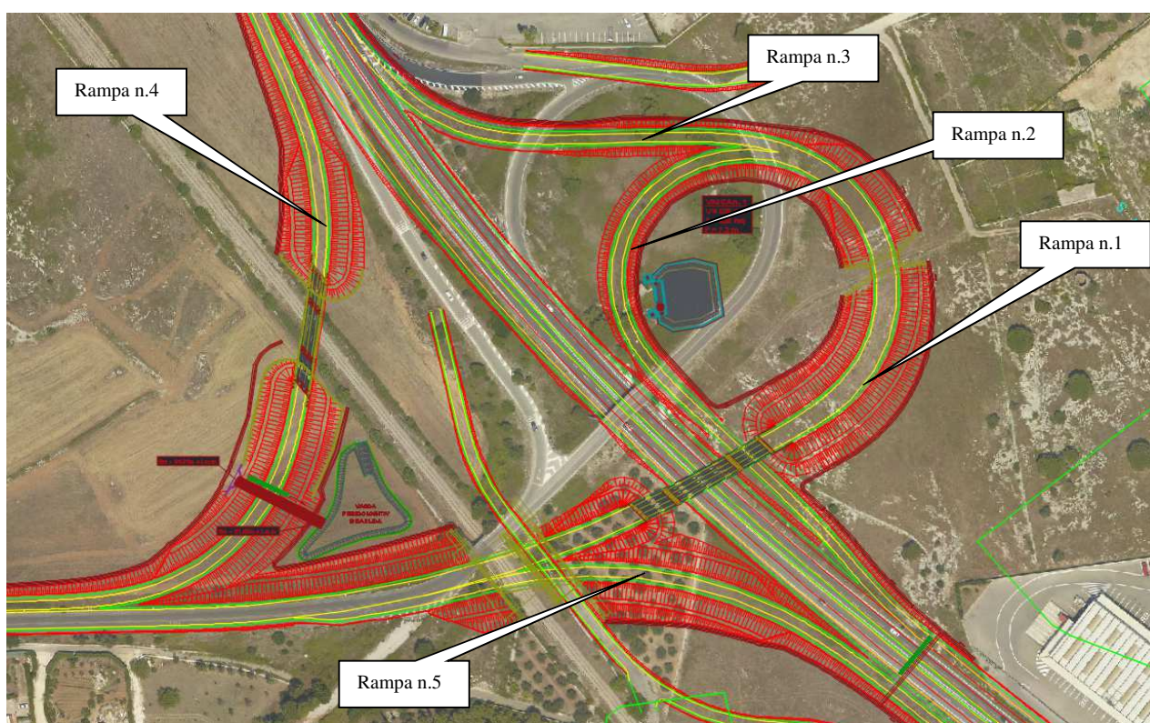
Figura 11: Svincolo n.1 Maglie Nord – configurazione di Progetto
