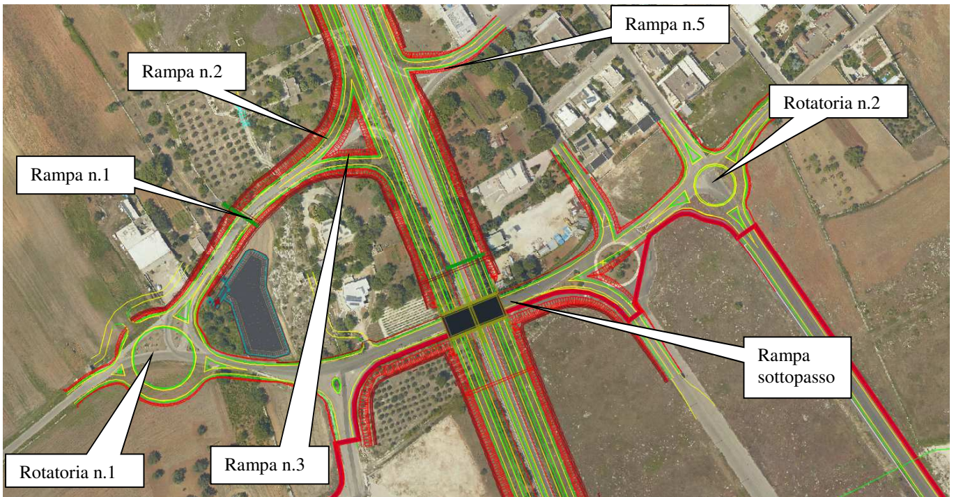
Figura 19: Svincolo 8 – BOTRUGNO SAN CASSIANO – nuova configurazione di progetto
