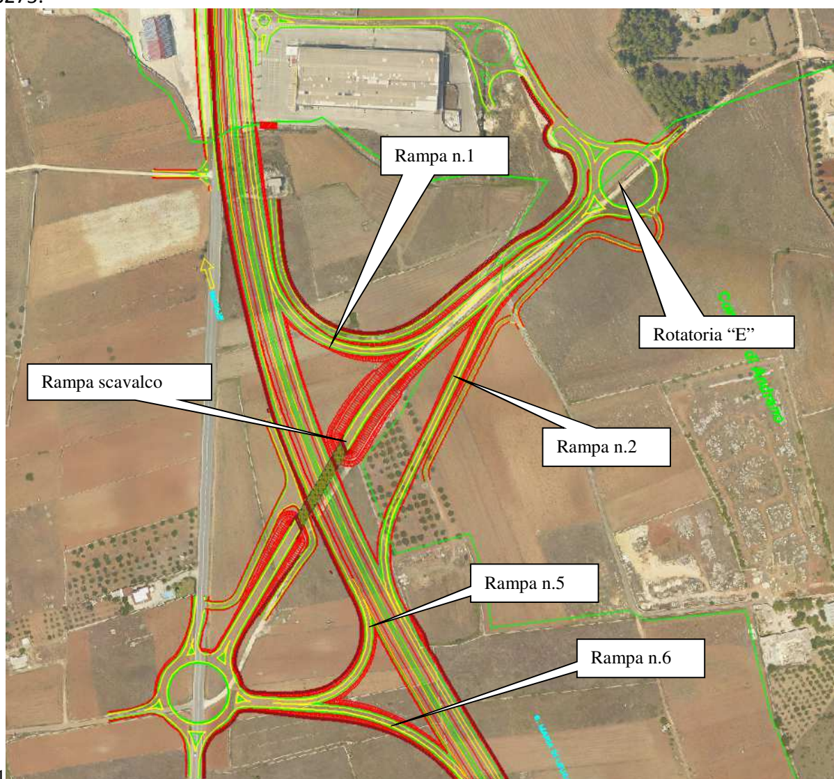
Figura 24: Svincolo 11 – Montesano Nord configurazione di progetto
