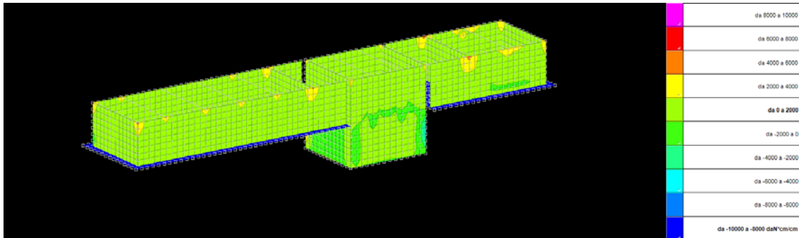
Figura 4 – sollecitazioni Mo0 massime pareti
