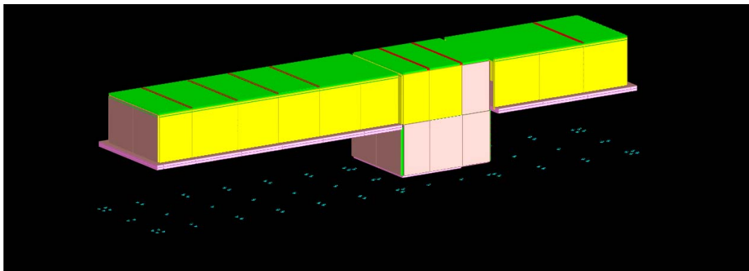
Figura 2 – schema strutturale
