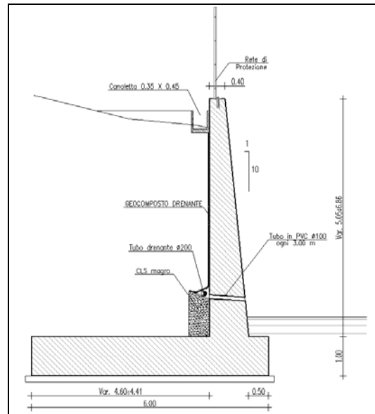
Sezione tipo con drenaggio
