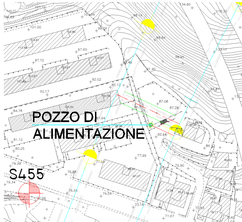
Figura 4 – Stralcio planimetrico sondaggio
