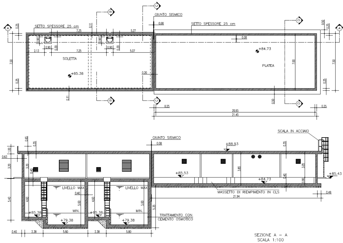
pianta e sezioni dell'intervento
