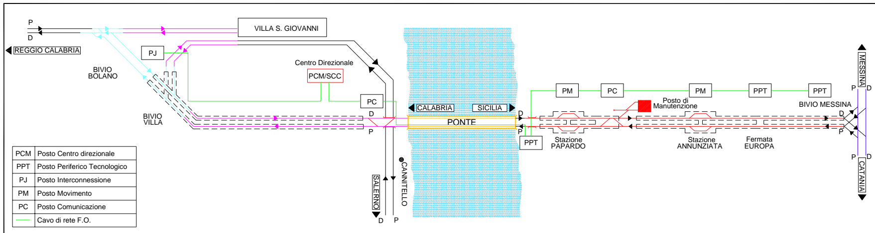
Figura 1 Descrizione ACCM Ponte Messina
