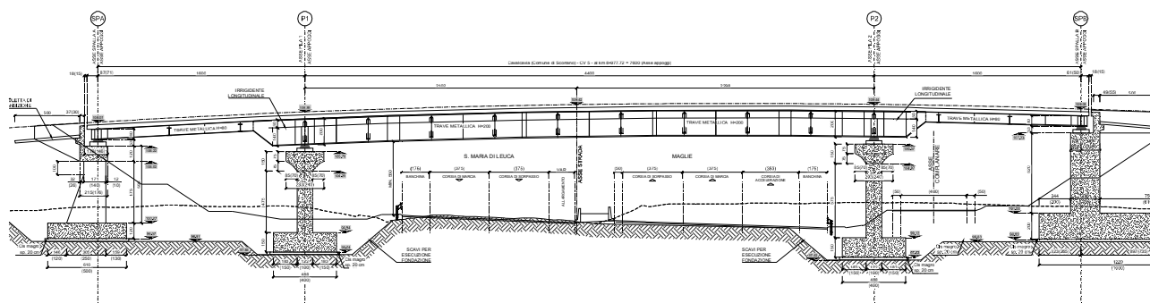
Figura 1-1: Prospetto longitudinale
