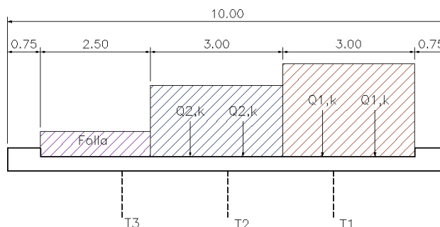
Figura 6-1 – Disposizione eccentrica dei carichi mobili
