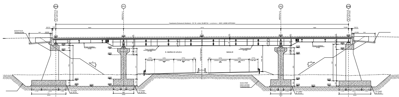
Figura 1-1: Prospetto longitudinale
