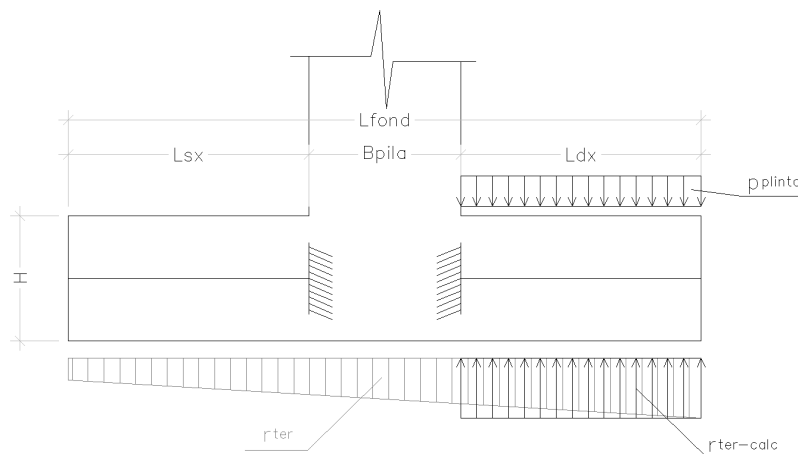
F 17. Schema di calcolo plinto di fondazione pila – Direzione longitudinale
