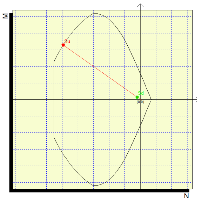
F 16. Dominio di interazione N-M
