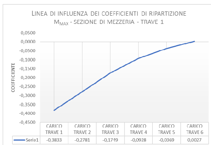
F 11. Linea d'influenza dei coefficienti di ripartizione
