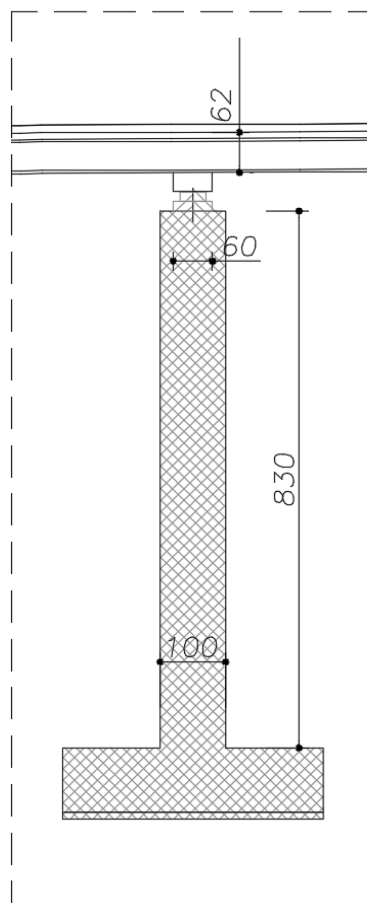
F 13. Sezione trasversale pila
