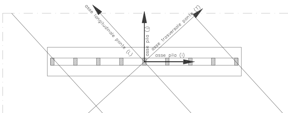
F 15. Schema degli assi principali "i-j" assunti nella verifica della pila
