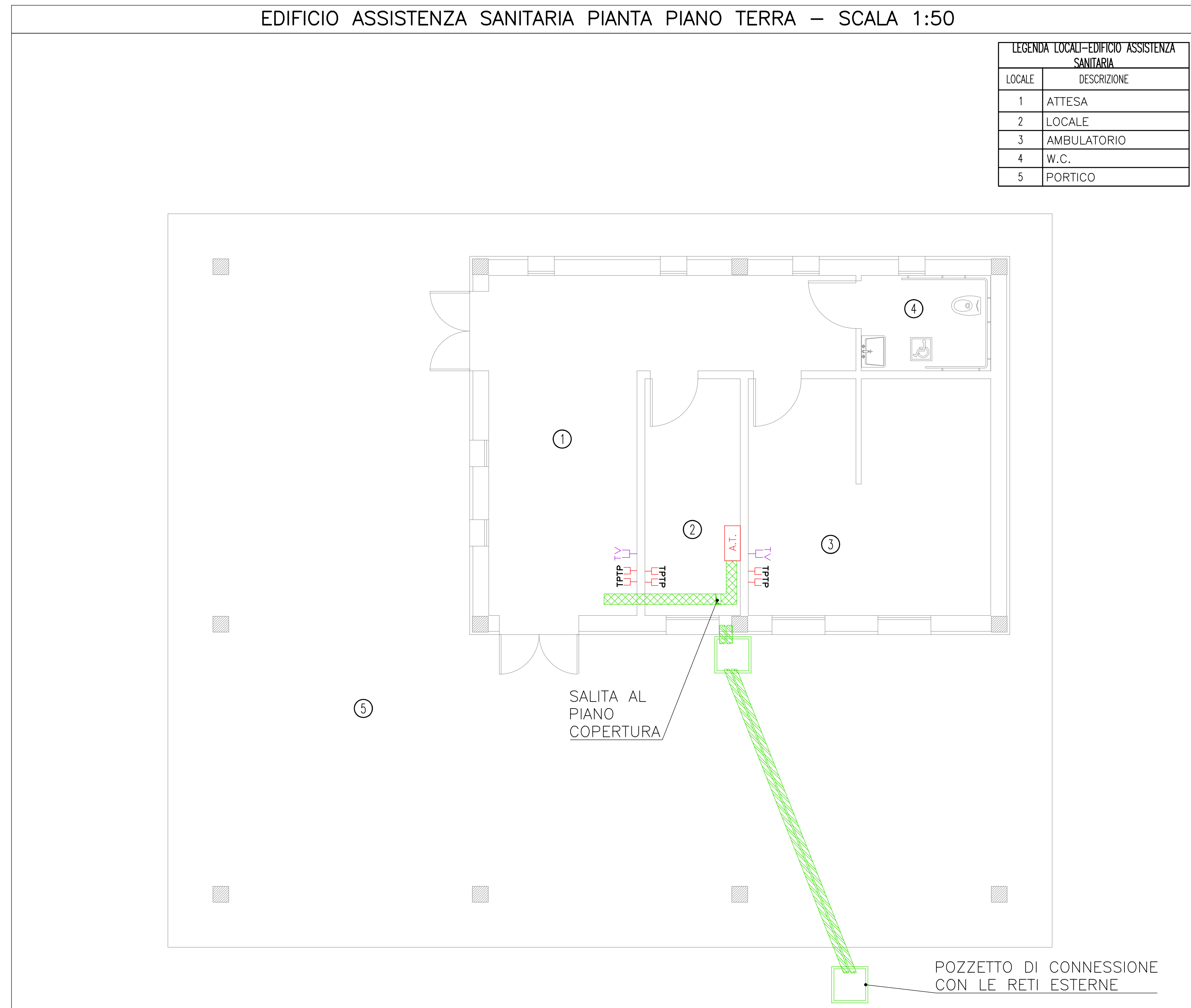
EDIFICIO ASSISTENZA SANITARIA PIANTA PIANO TERRA – SCALA 1:50
