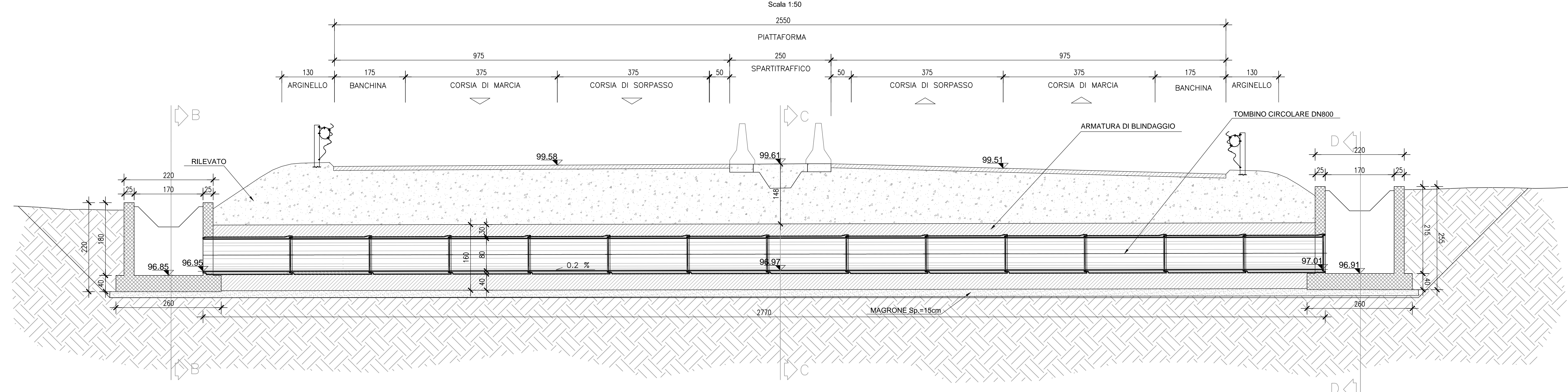
SEZIONE LONGITUDINALE A-A
