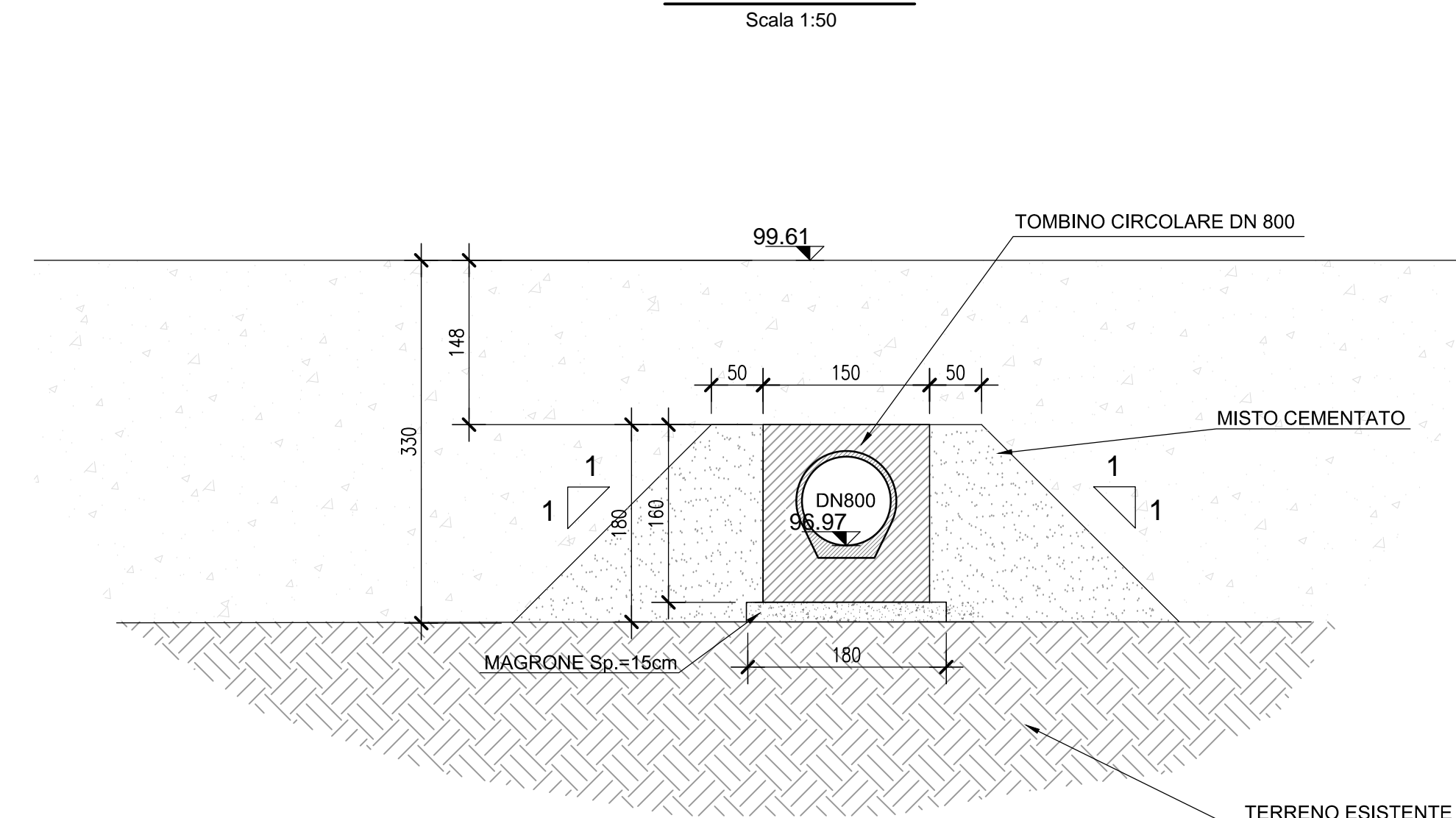
SEZIONE C-C
