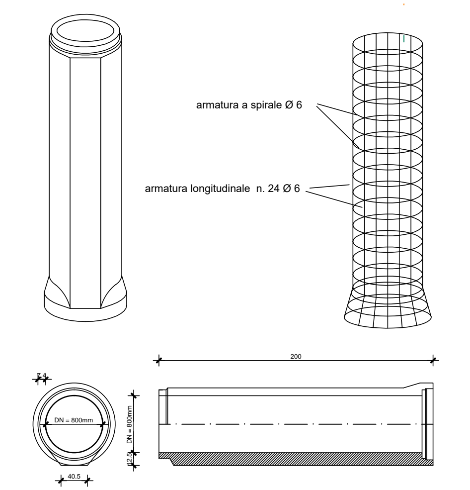
SCHEMA TUBO
