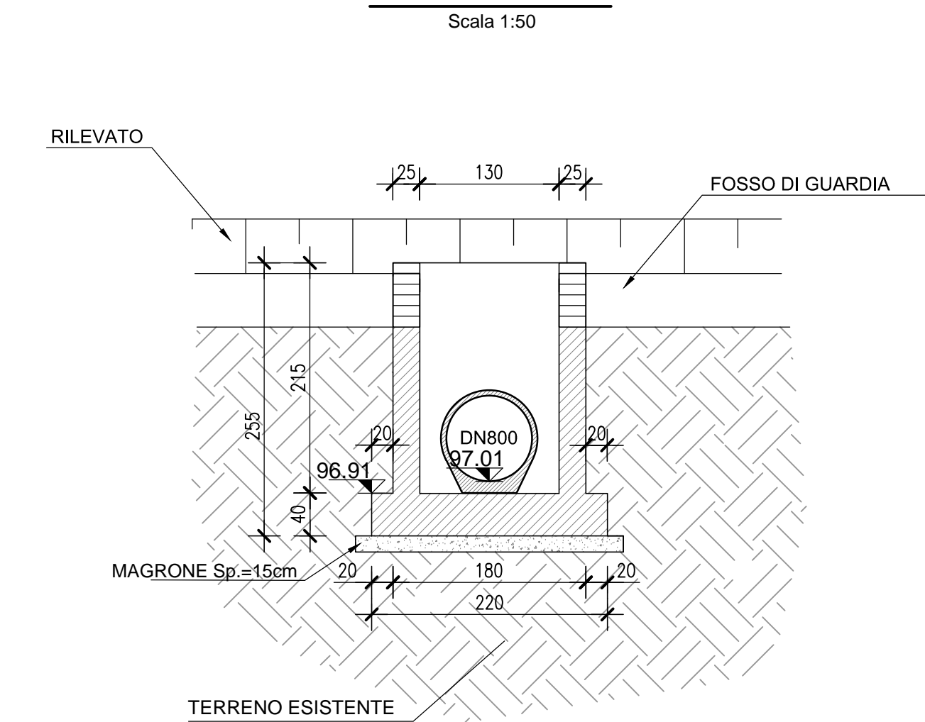
SEZIONE D-D
