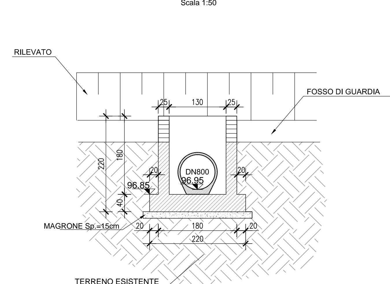
SEZIONE B-B
