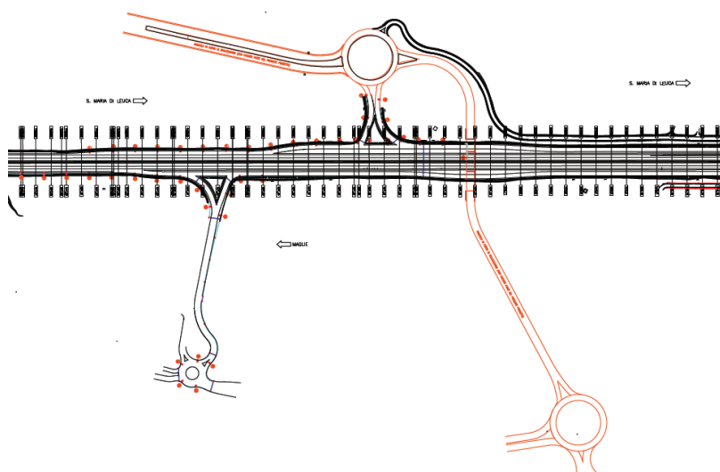
Figura 1 – Planimetria dello svincolo SV1B di Maglie Melpigliano
